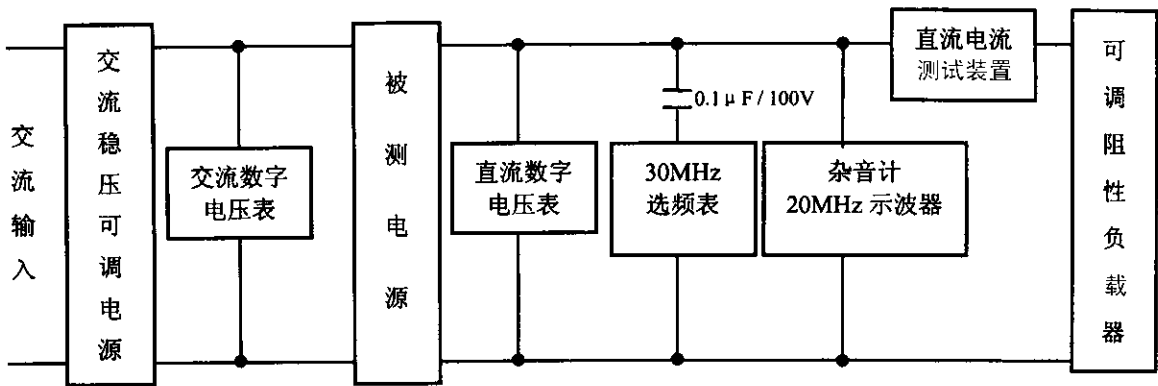
图3 杂音电压试验电路
