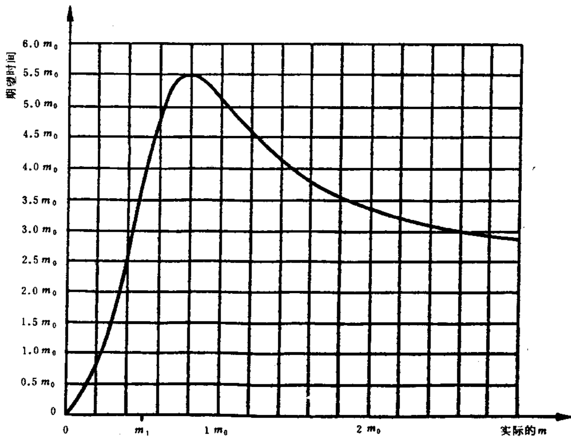
图 7 试验方案4:2判定的期望相关试验时间
