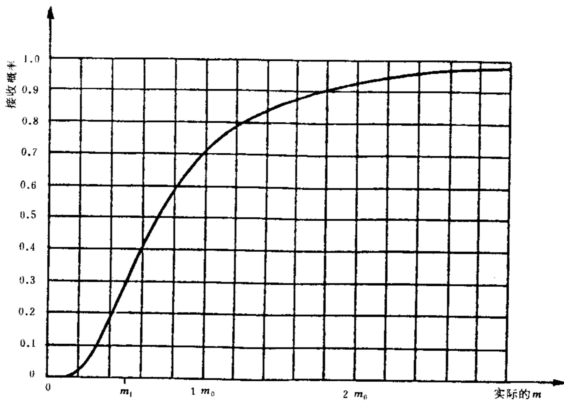
图 27 试验方案4:9工作特性曲线
