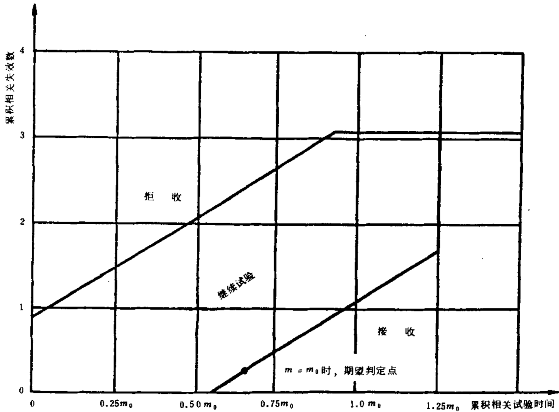
图 11 试验方案4:4 ( \alpha=0.10, \beta=0.10, D_m=5.0 )
