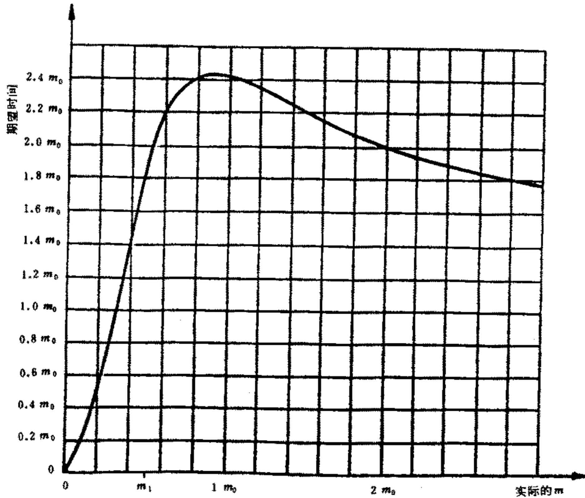
图 19 试验方案4:6判定的期望相关试验时间
