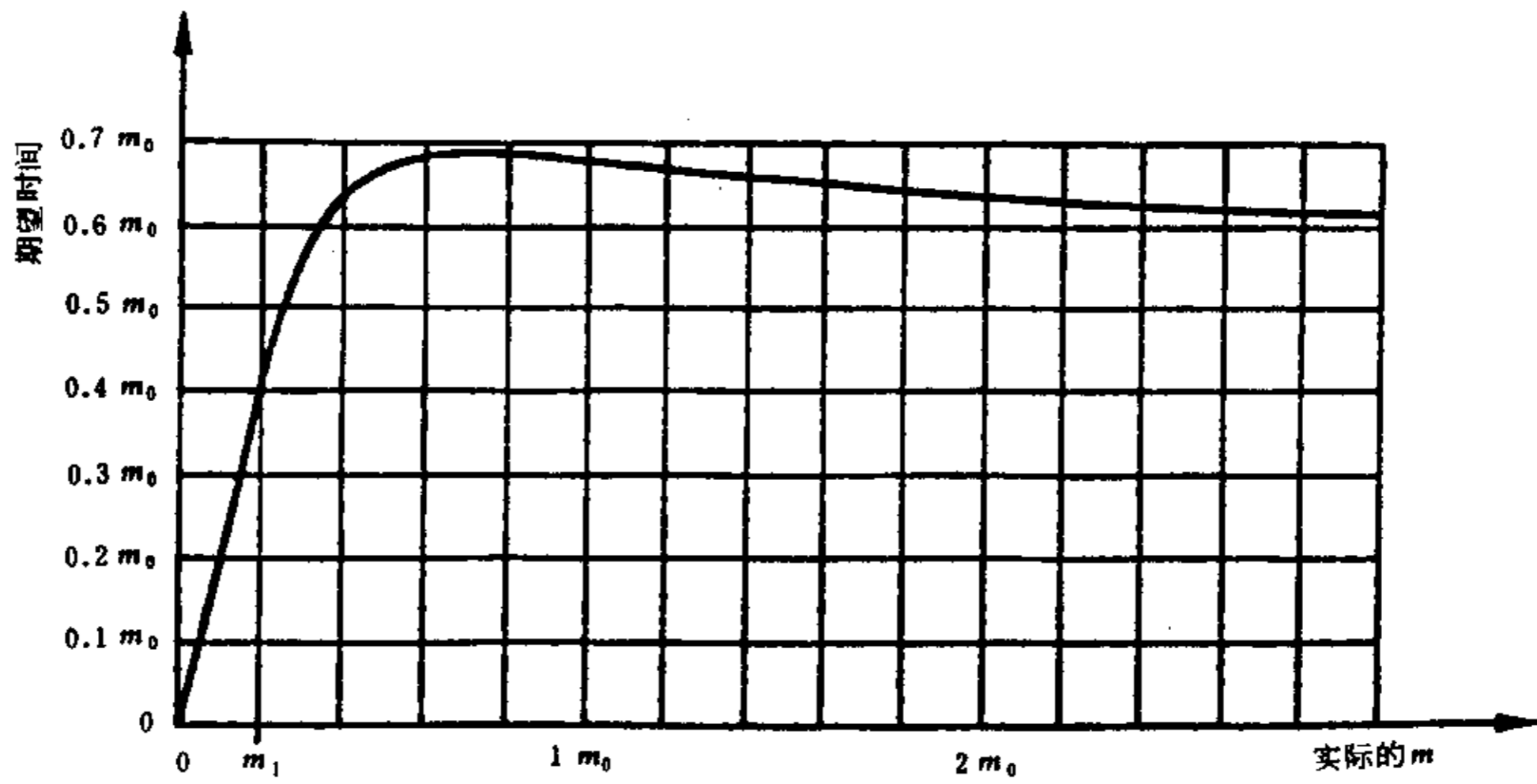
图 13 试验方案4:4判定的期望相关试验时间
