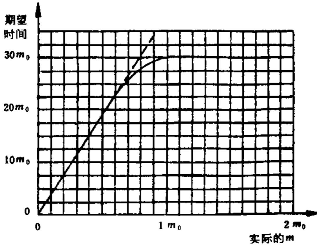
图 33 试验方案5:1判定的期望相关试验时间
