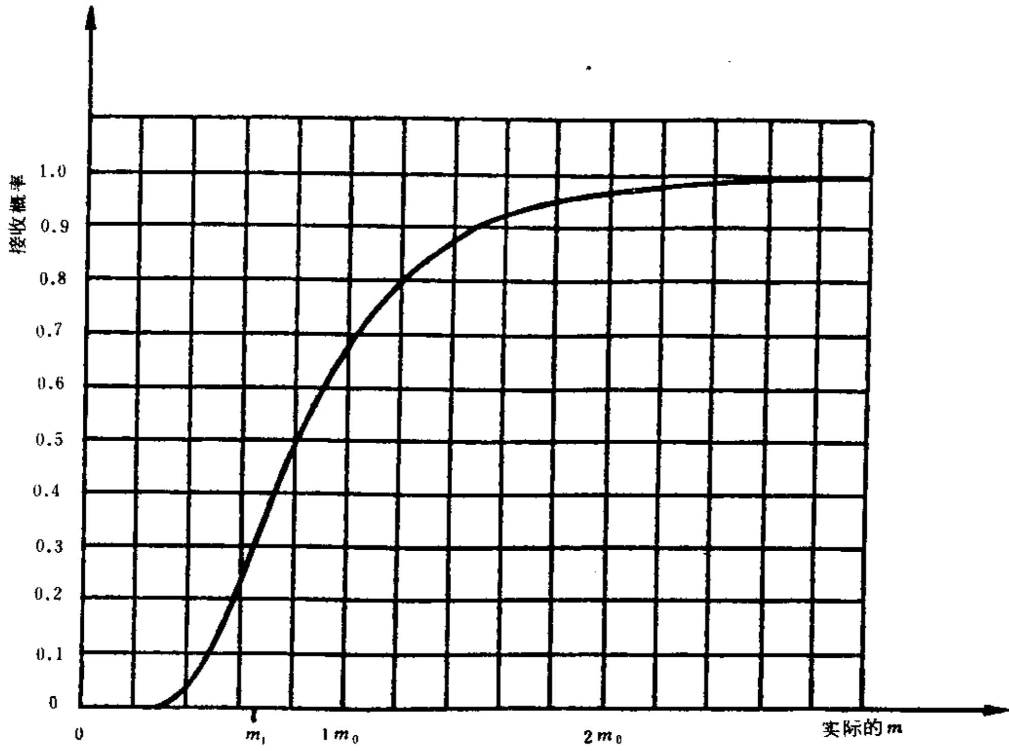
图 24 试验方案4:8工作特性曲线
