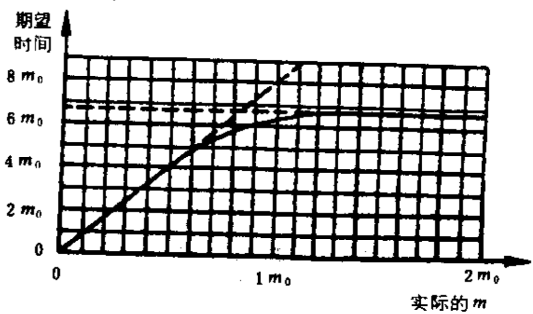
图 44 试验方案5:10判定的期望相关试验时间
