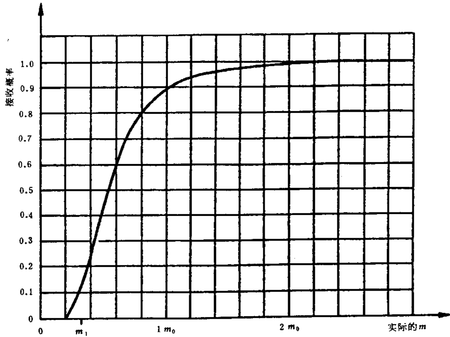
图 9 试验方案4:3工作特性曲线
