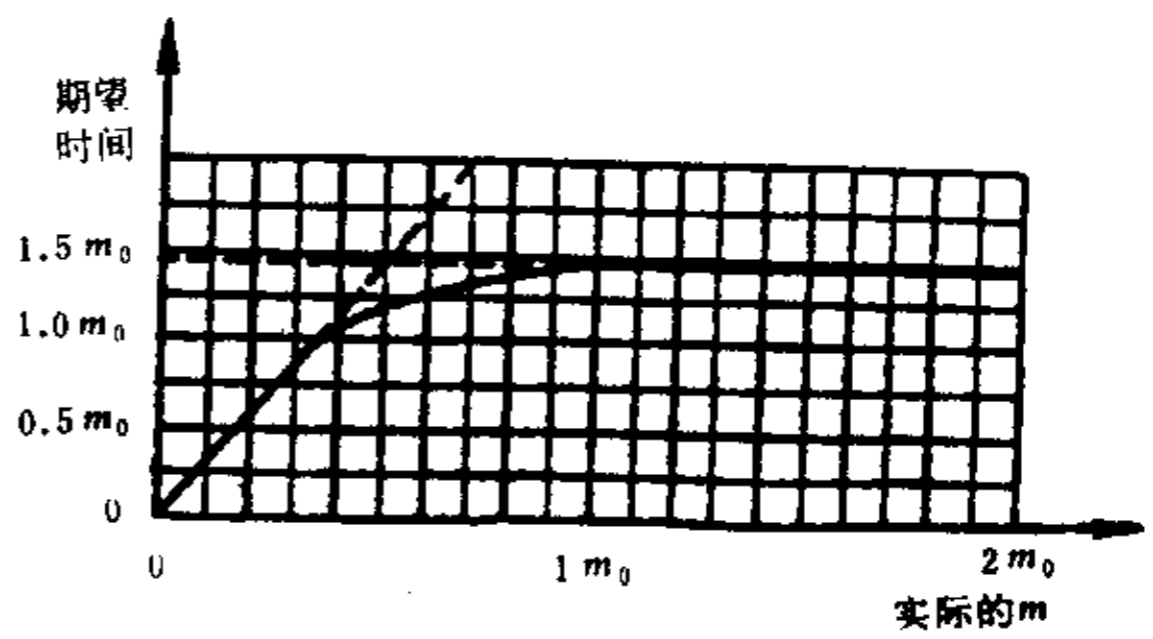
图 39 试验方案5:6判定的期望相关试验时间 图 40 试验方案5:7判定的期望相关试验时间
