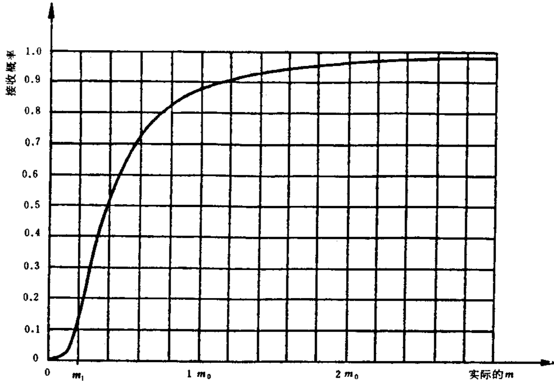
图 12 试验方案4:4工作特性曲线
