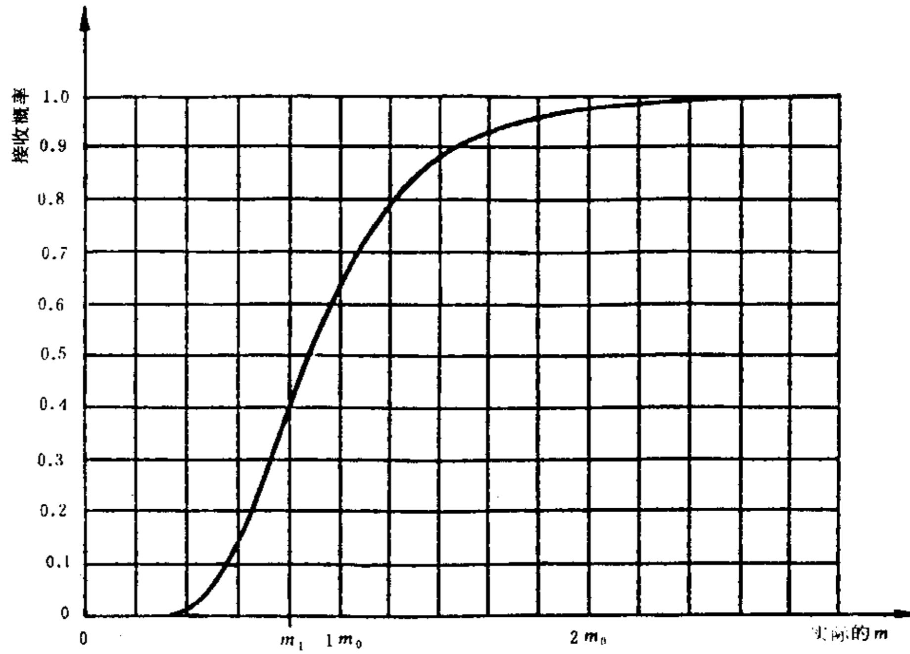
图 30 试验方案4:10工作特性曲线
