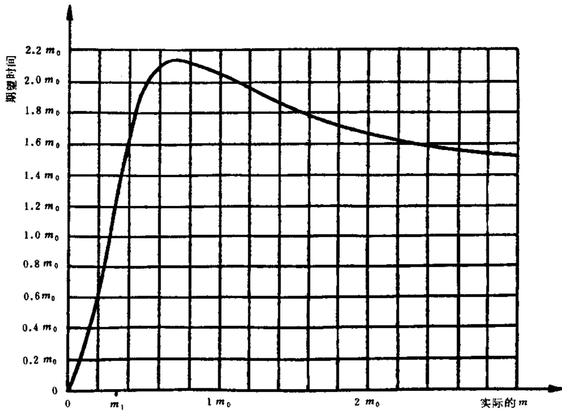
图 10 试验方案4:3判定的期望相关试验时间
