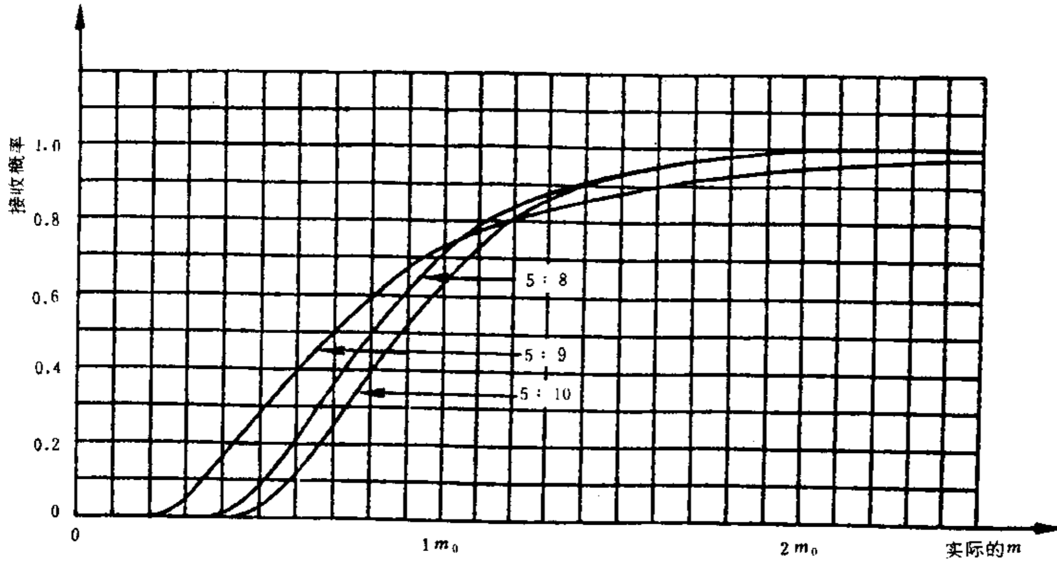
图 41 试验方案5:8, 5:9和5:10工作特性曲线
