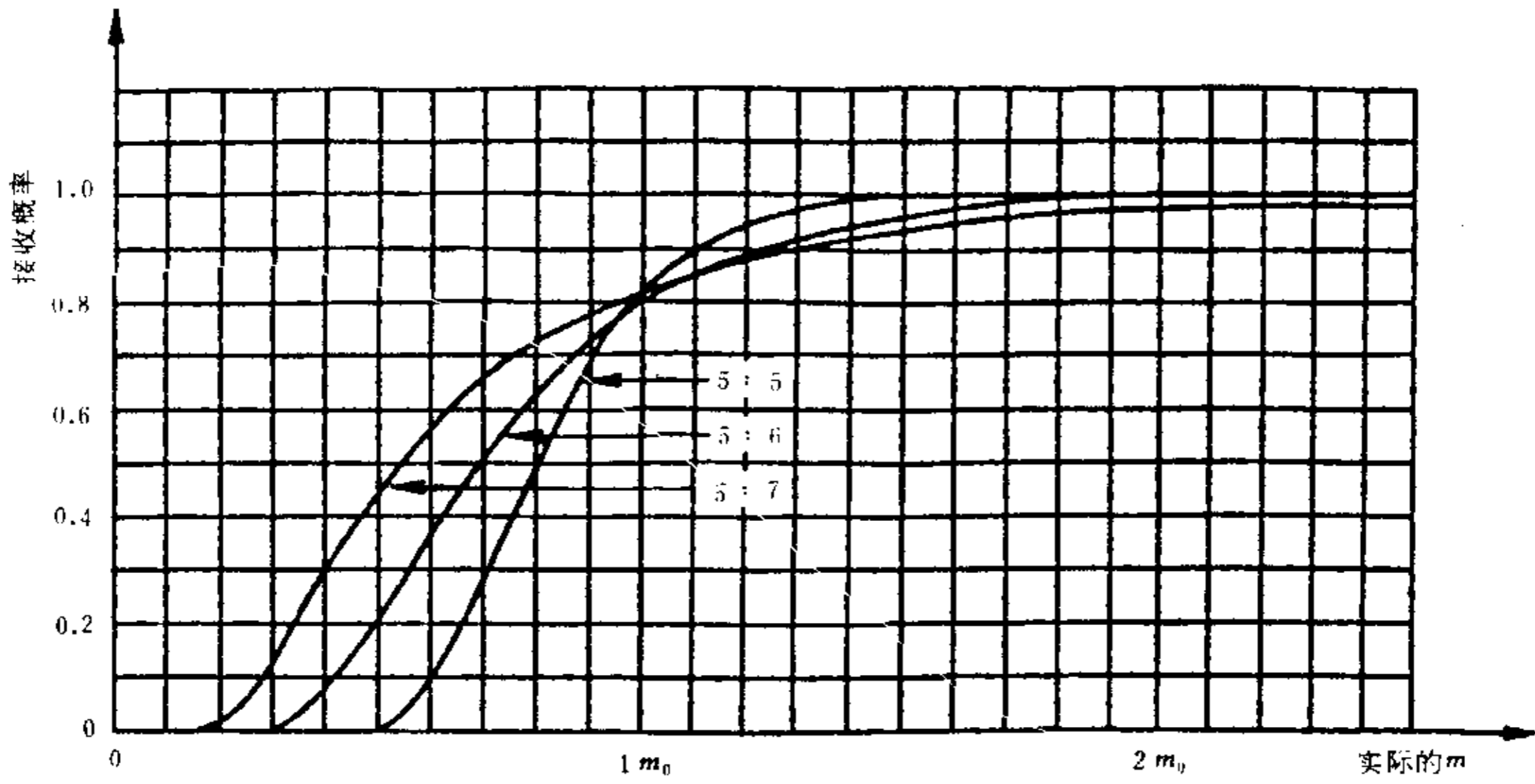
图 37 试验方案5:5, 5:6, 5:7 工作特性曲线
