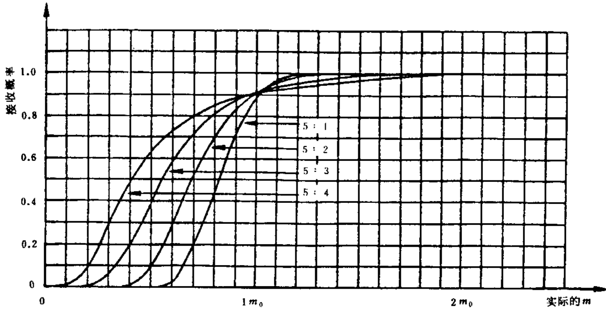
图 32 试验方案5:1, 5:2, 5:3和5:4工作特性曲线
