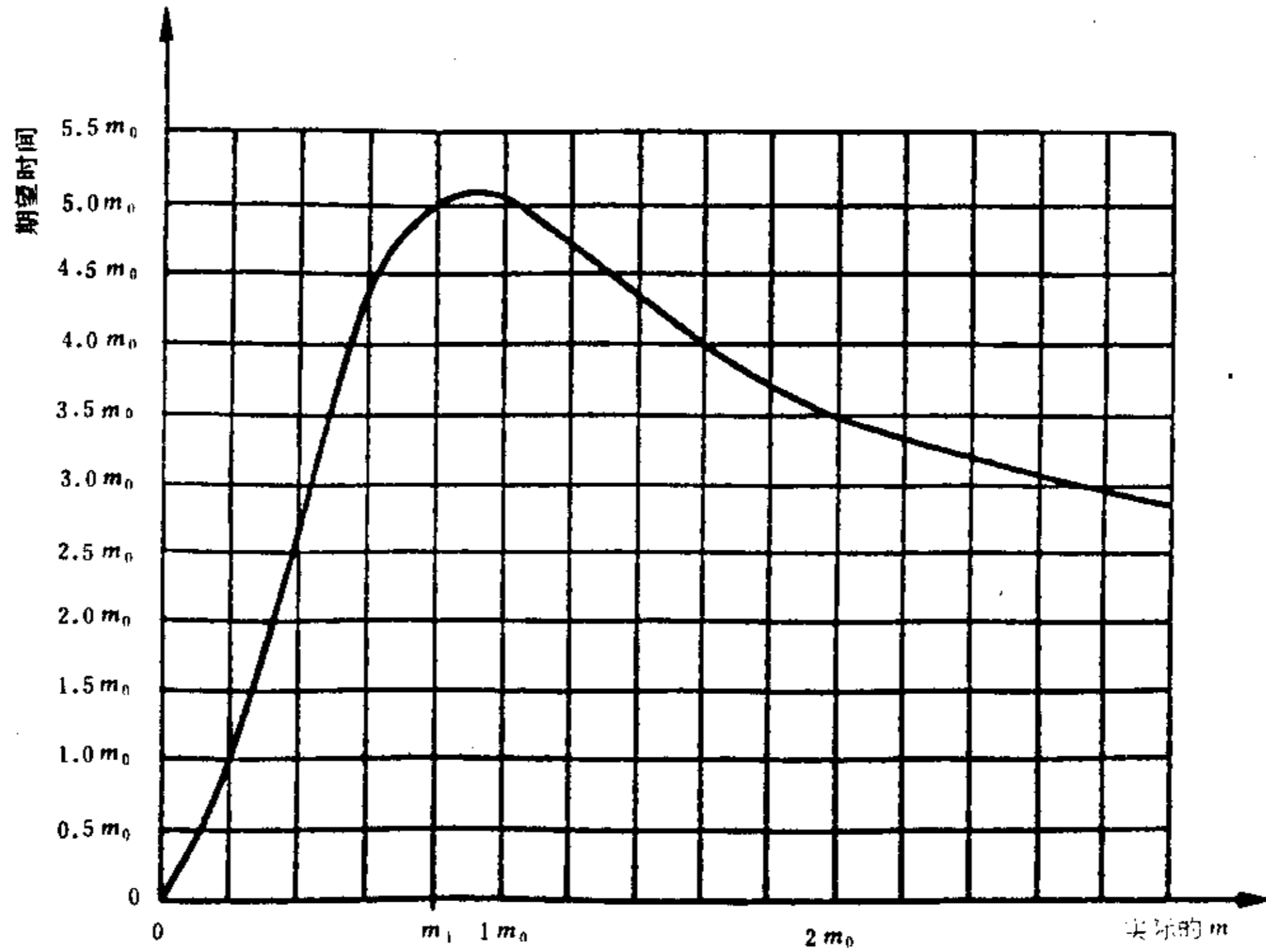
图 31 试验方案4:10判定的期望相关试验时间
