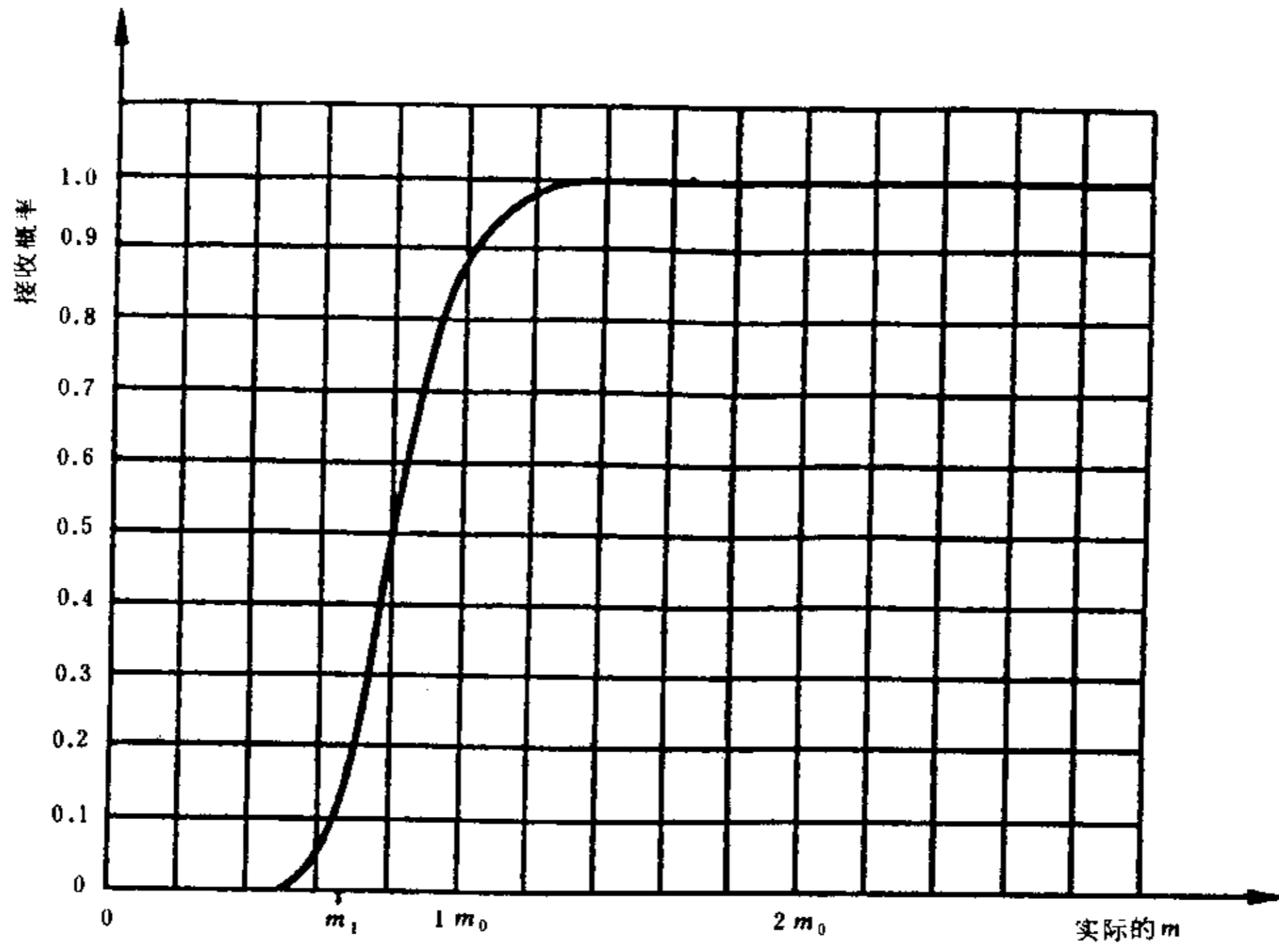
图 3 试验方案4:1工作特性曲线
