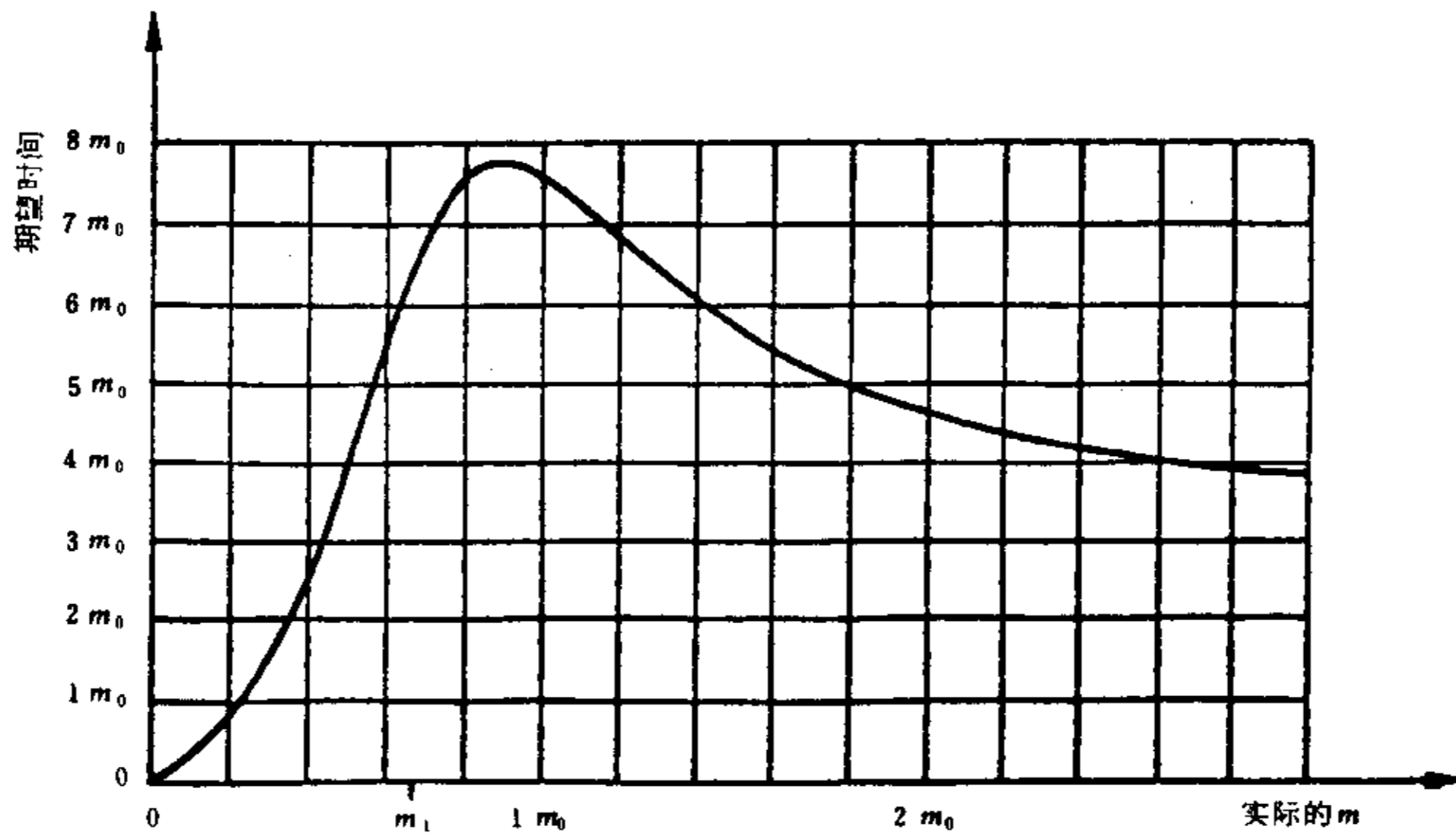
图 16 试验方案4:5判定的期望相关试验时间
