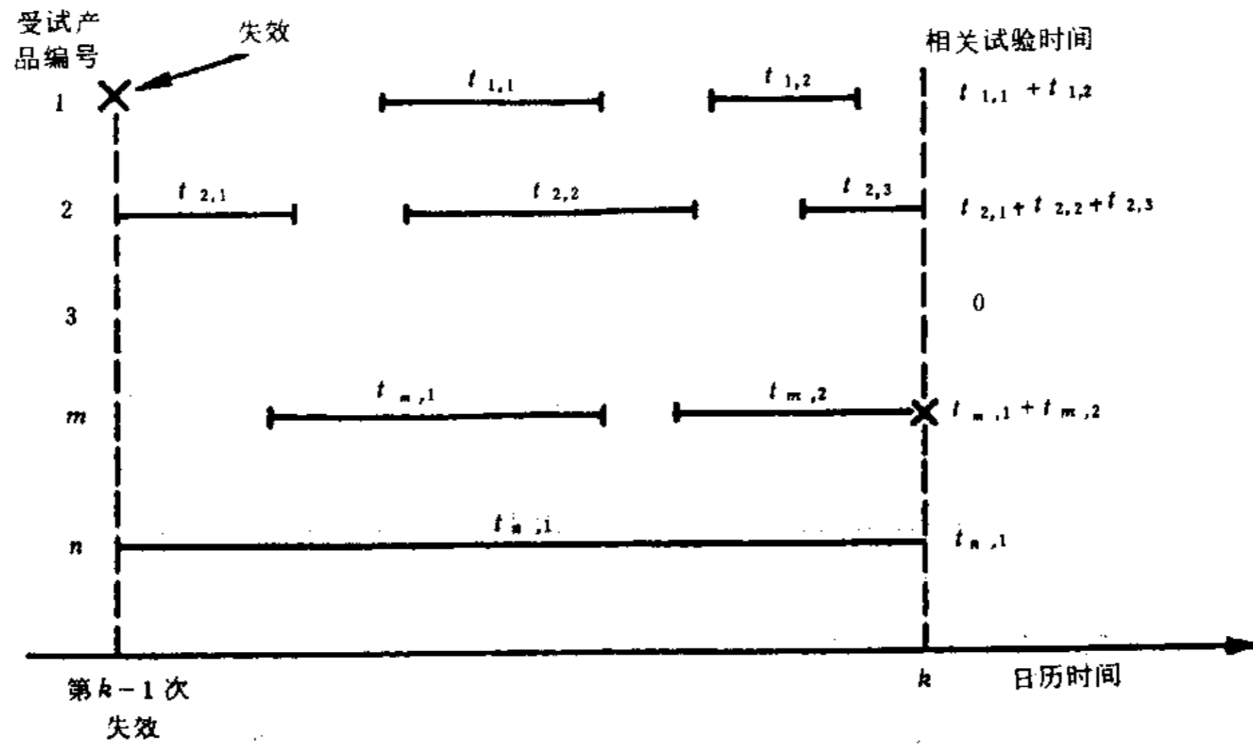
图 1 相关试验时间的周期编号 在判定点上未出现失效时的累积相关试验时间 T^* 为:
