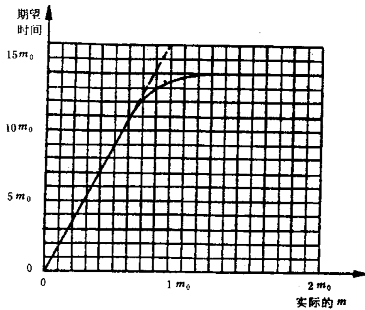
图 38 试验方案5:5判定的期望相关试验时间
