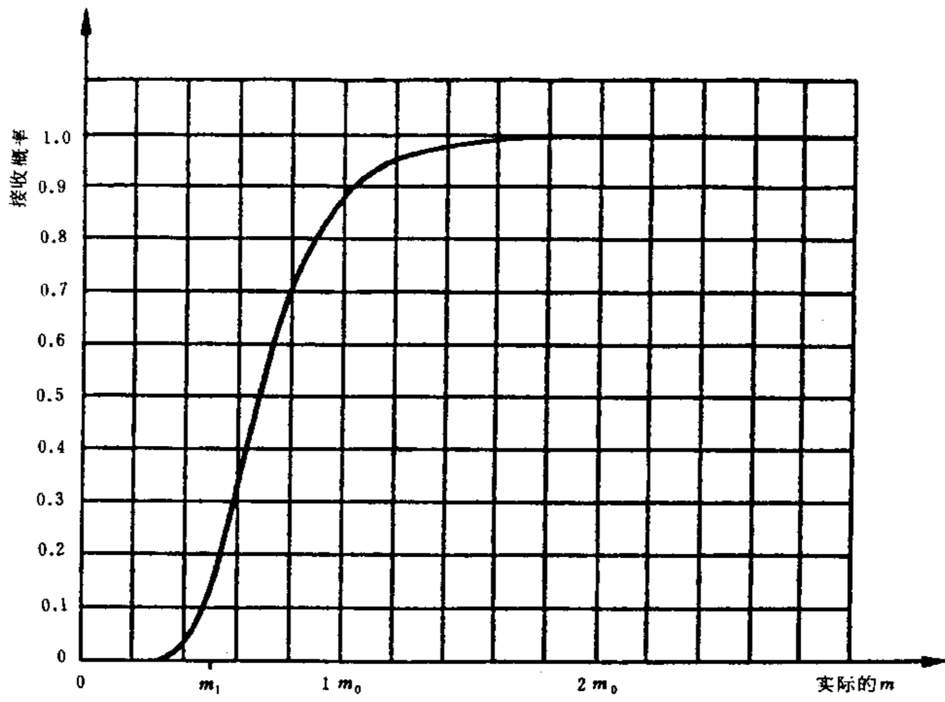
图 6 试验方案4:2工作特性曲线
