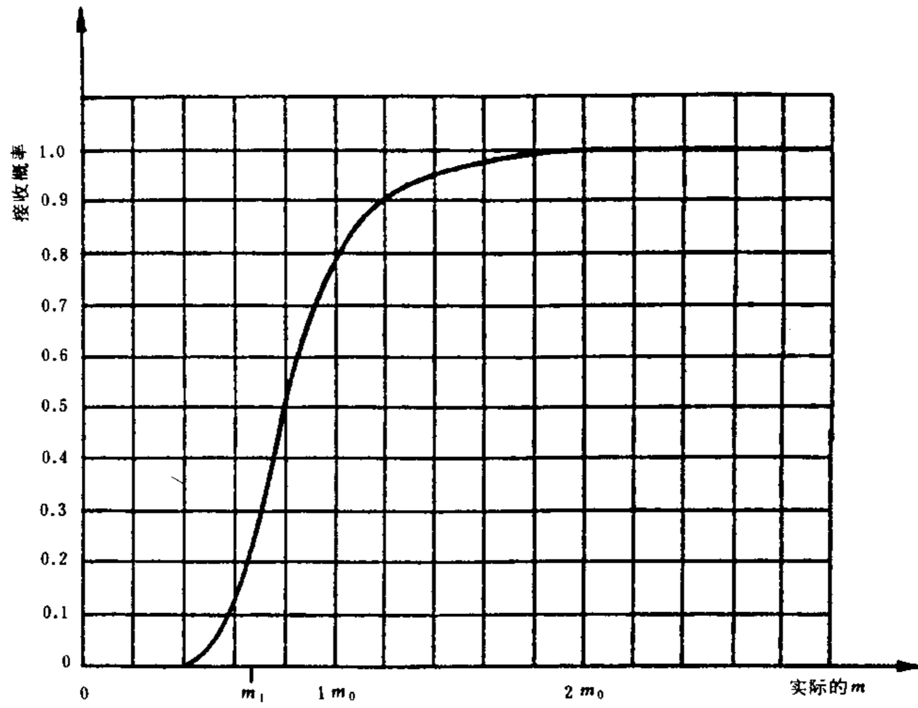
图 15 试验方案4:5工作特性曲线
