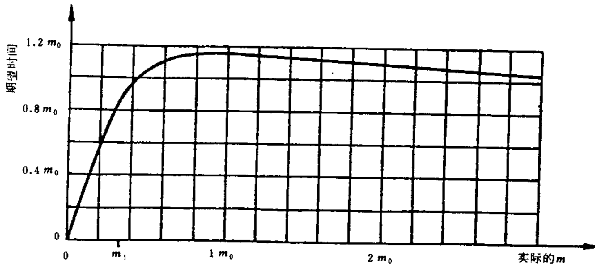
图 22 试验方案4:7判定的期望相关试验时间
