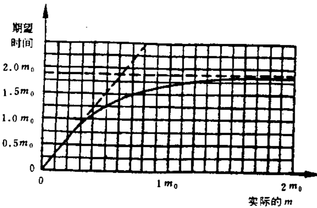
图 43 试验方案5:9判定的期望相关试验时间
