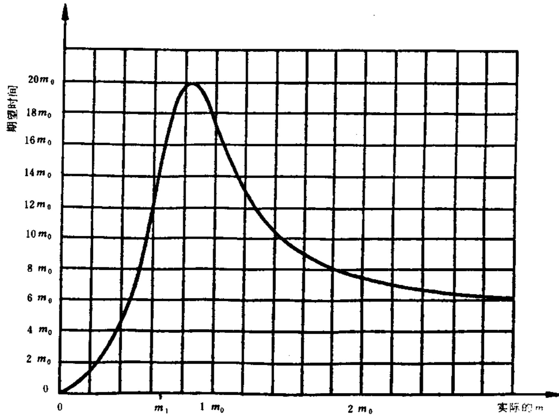
图 4 试验方案4:1判定的期望相关试验时间
