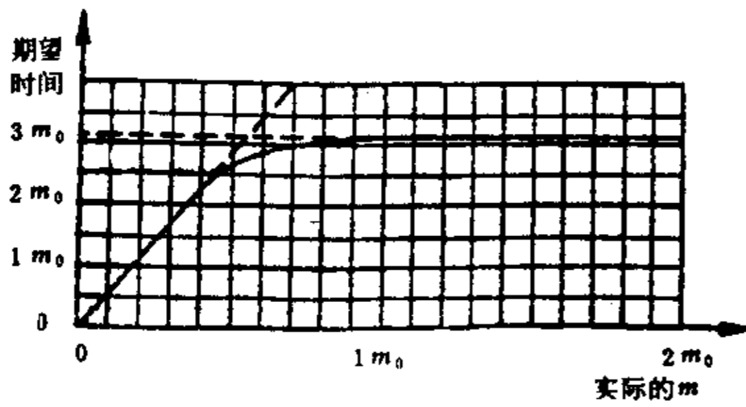
图 35 试验方案5:3判定的期望相关试验时间
