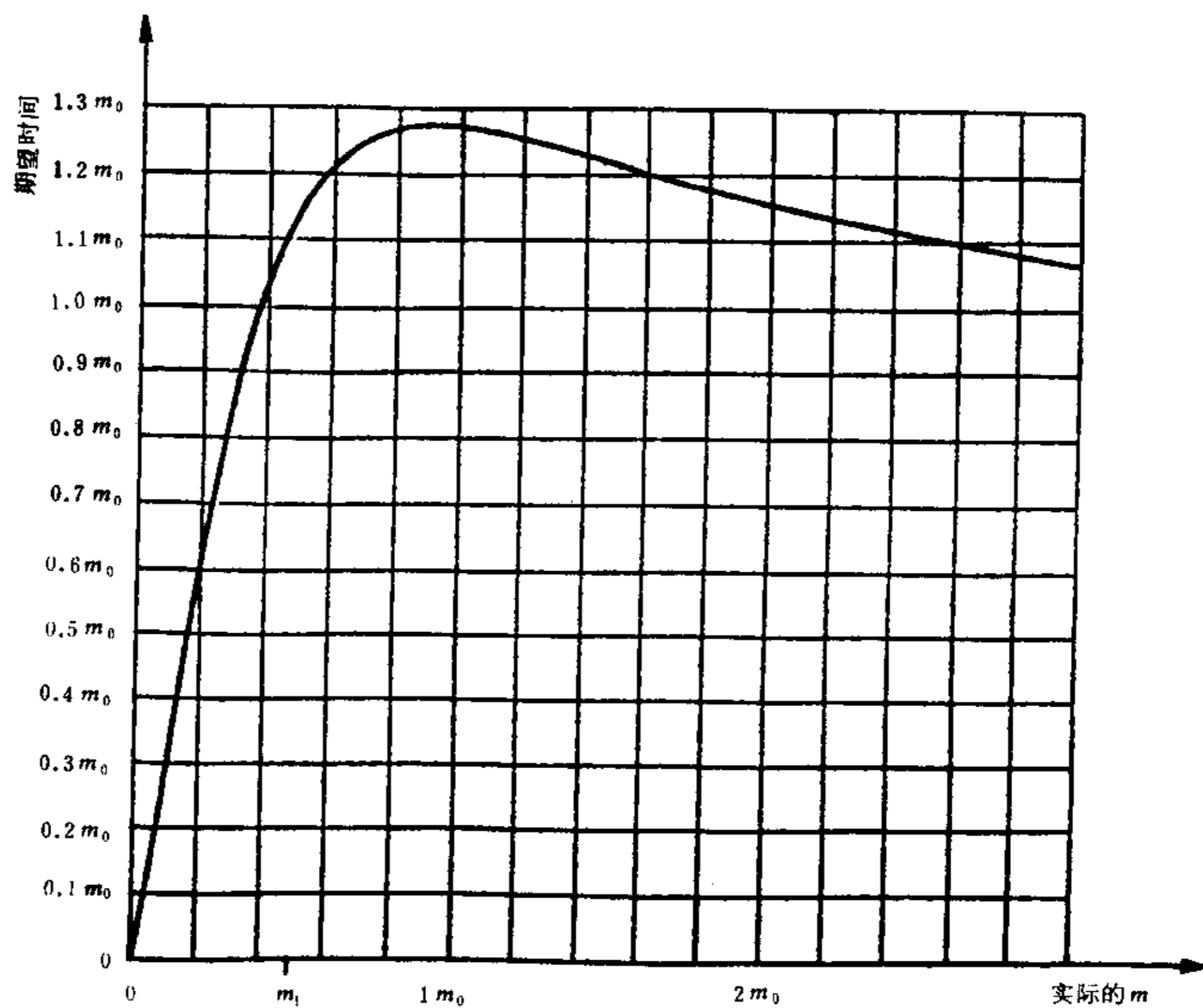
图 28 试验方案4:9判定的期望相关试验时间
