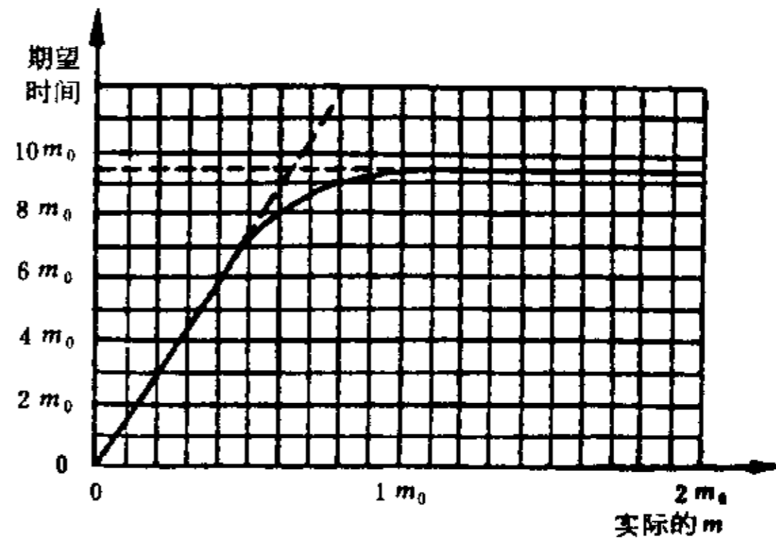
图 34 试验方案5:2判定的期望相关试验时间
