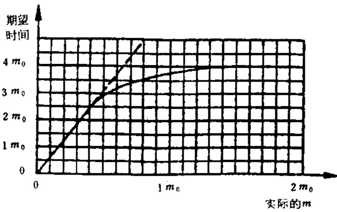
图 39 试验方案5:6判定的期望相关试验时间 图 40 试验方案5:7判定的期望相关试验时间
