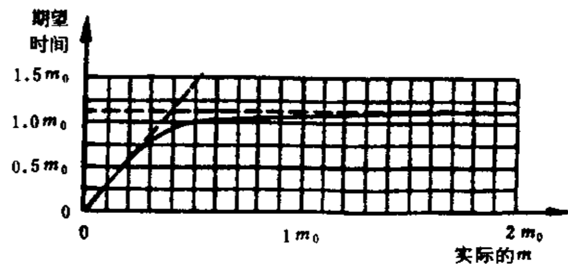
图 36 试验方案5:4判定的期望相关试验时间
