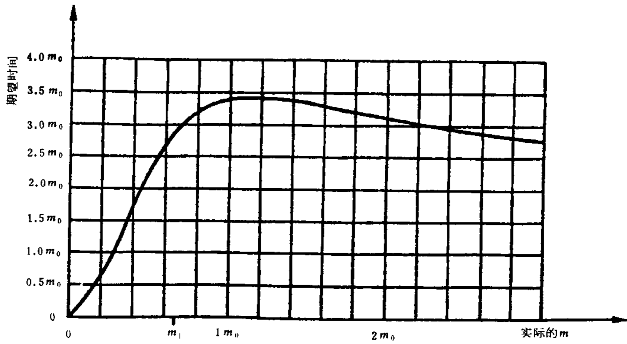
图 24 试验方案4:8工作特性曲线
