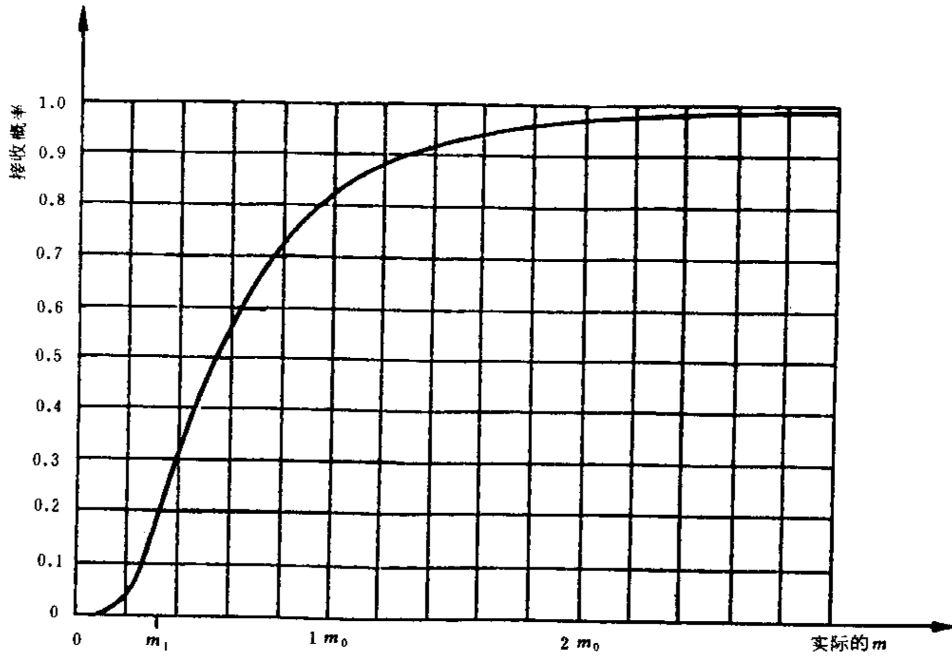
图 21 试验方案4:7工作特性曲线
