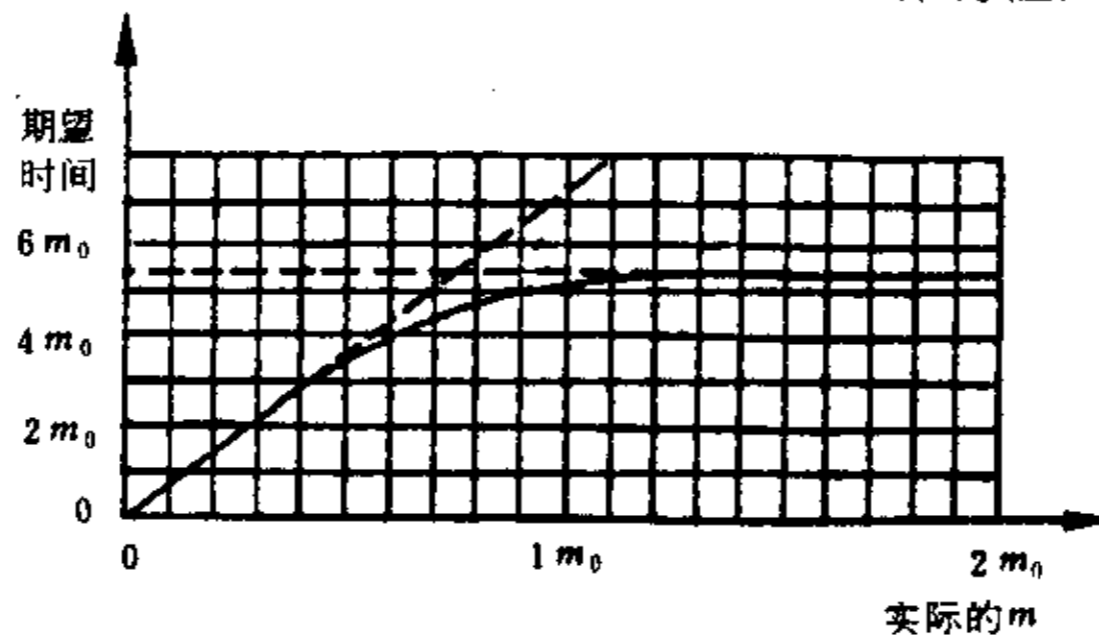
图 42 试验方案5:8判定的期望相关试验时间
