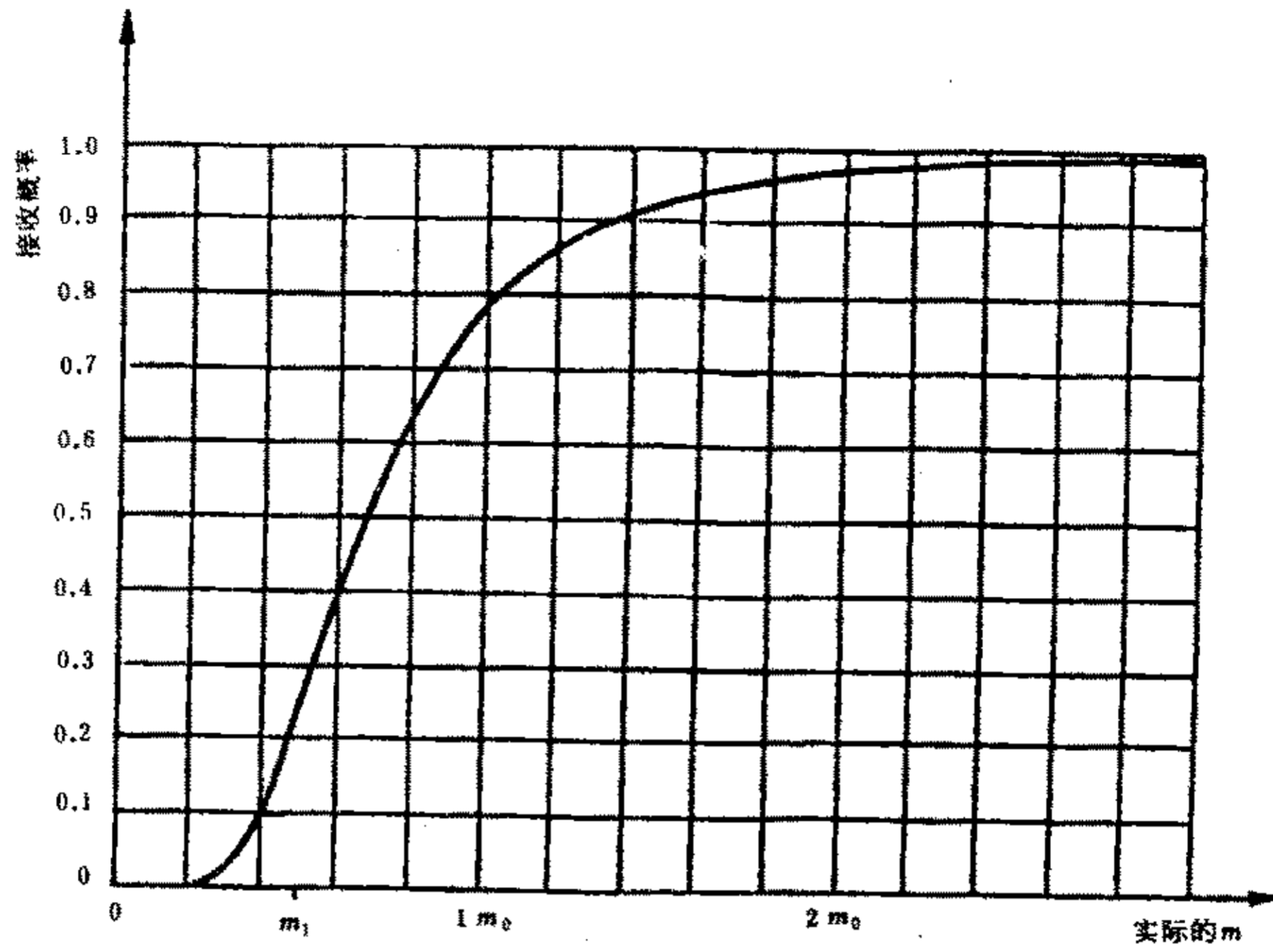
图 18 试验方案4:6工作特性曲线
