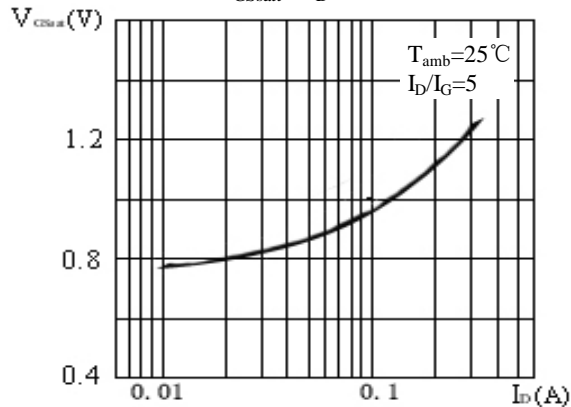
V_{GSsat} - I_D 关系曲线
