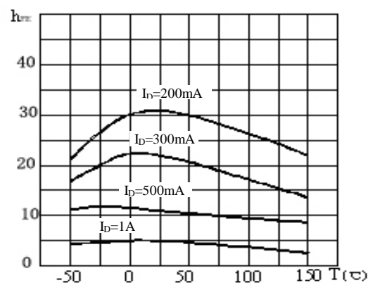
h_{FE} - T 关系曲线
