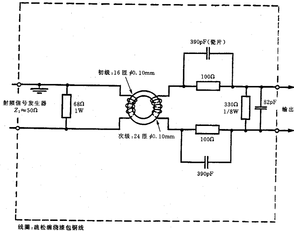
图 A2a) 平衡/不平衡转换器电路
