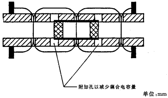
图 A2c) 变压器中心部分结构详图(截面图)
