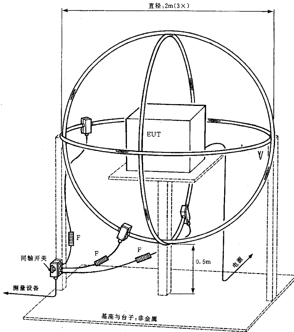
图 B1 测量 X、Y 和 Z 方向的磁场的试验装置(频率范围 9 kHz~30 MHz)
