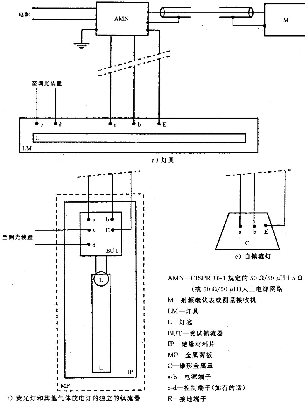
图 6 测量布置
