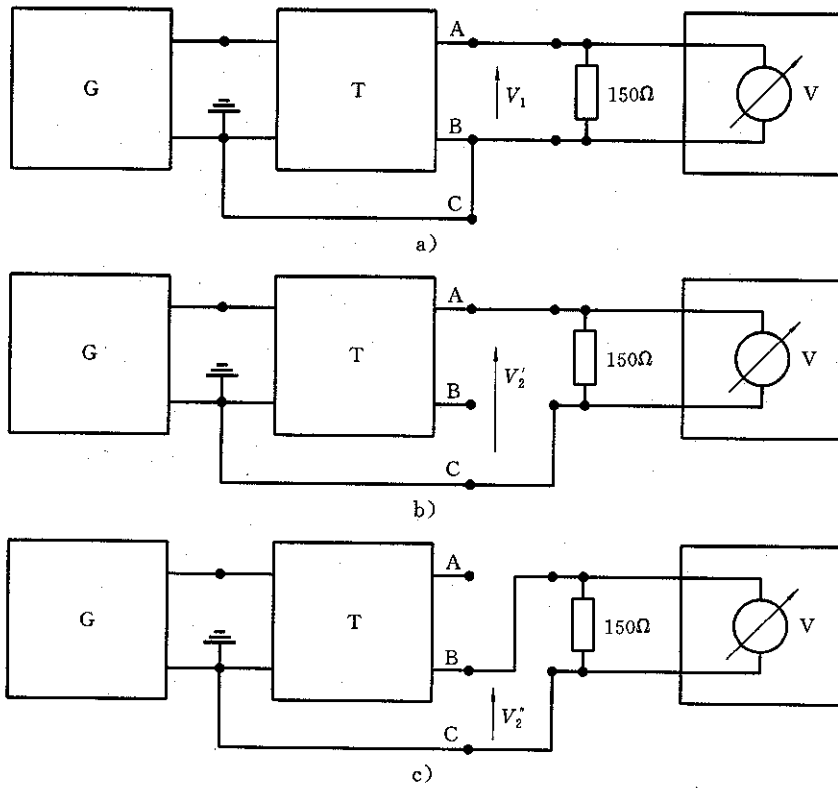
图 A1 隔离试验线路布置
