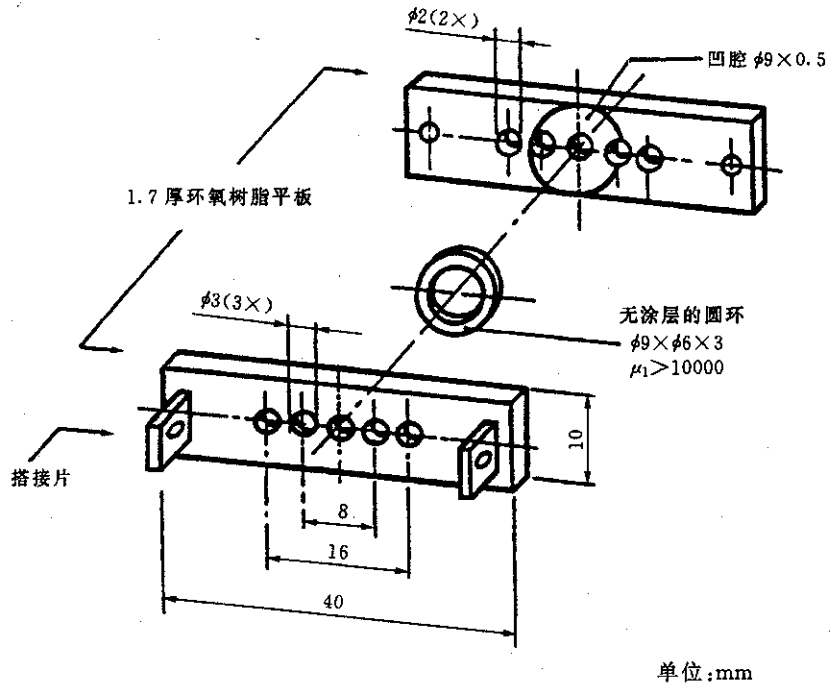
图 A2b) 变压器中心部分结构详图(部分分解图)
