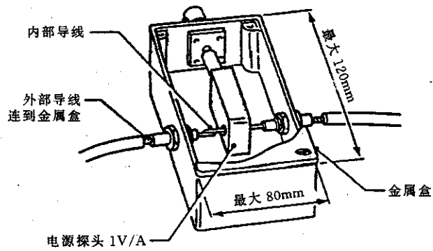
图 B2 大环结构
