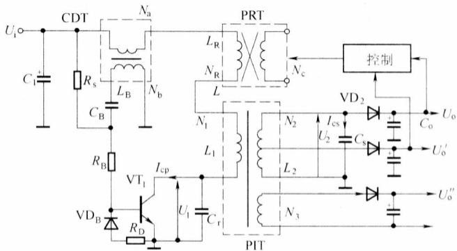
图 3-57 初级电压控制方式的电压谐振式变换器的电路
