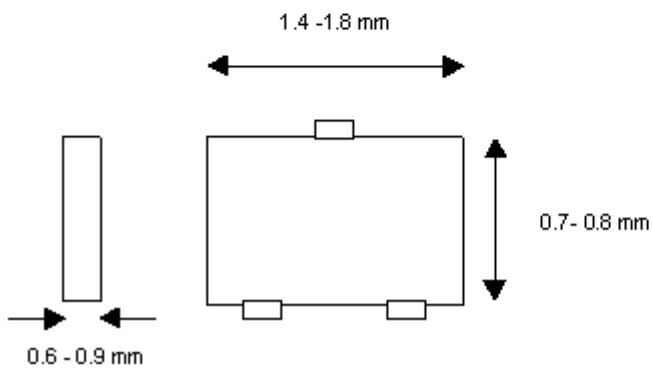
SOT- 416/SC- 90
