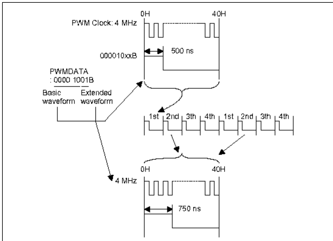
图 11-2 8 位‘延伸’波形
