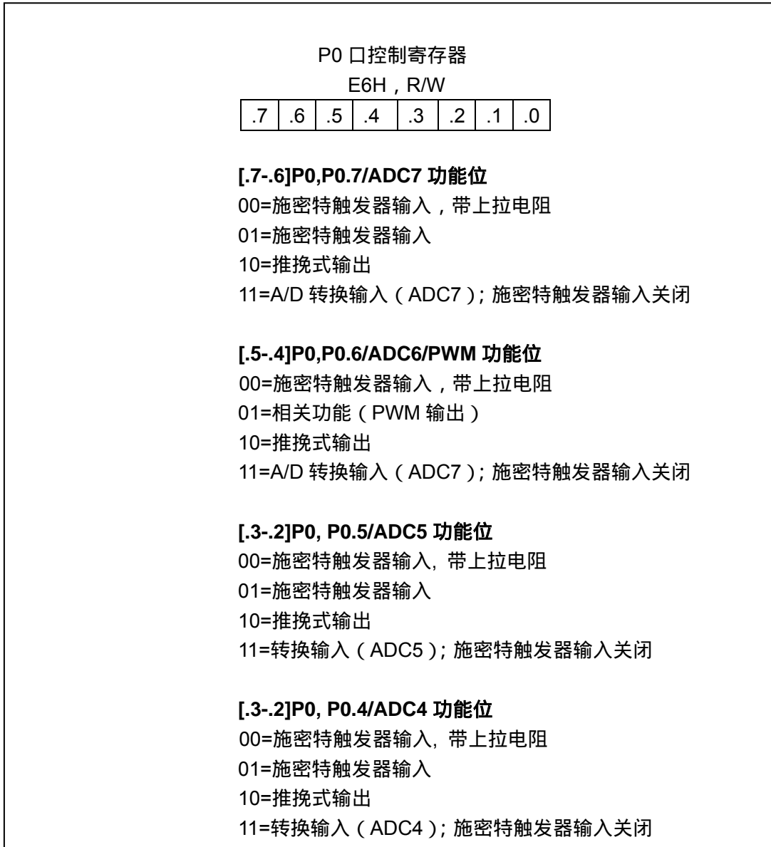
图 9-3 P0 口控制寄存器 (POCONH)
