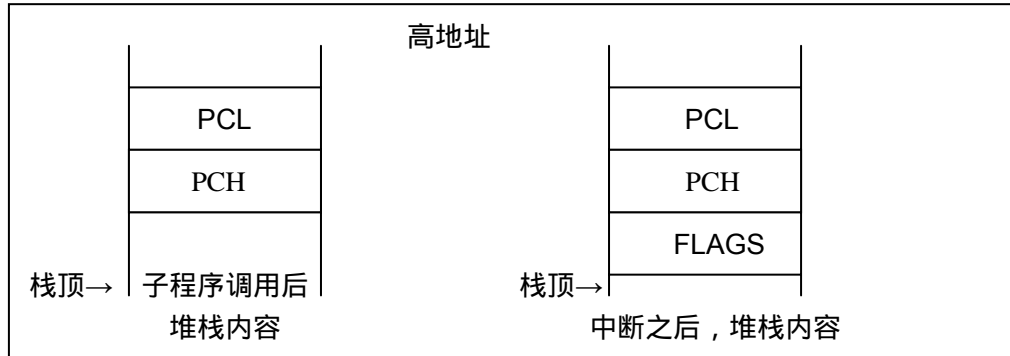
图 2-5 堆栈操作
