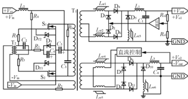
图8 完全利用磁放大器的稳压电路
