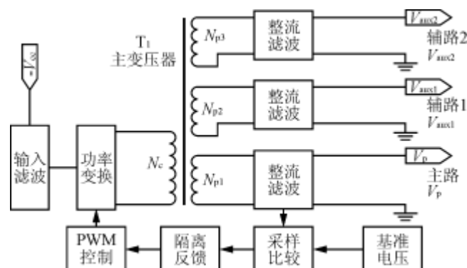
图1 多路输出开关电源框图
