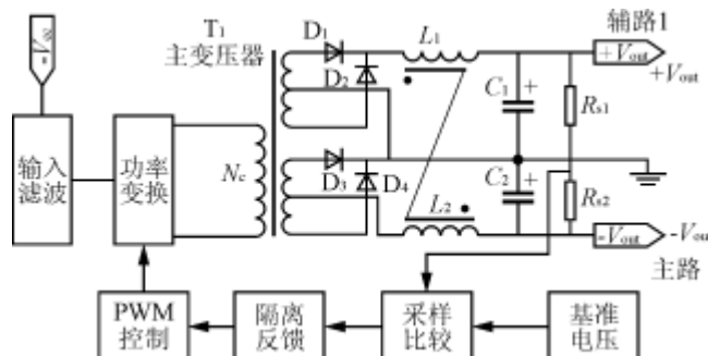
图4 改进型2路输出电路
