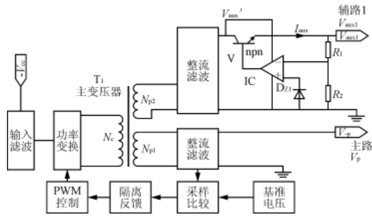
图3 辅助电路加一个线性稳压调节器
