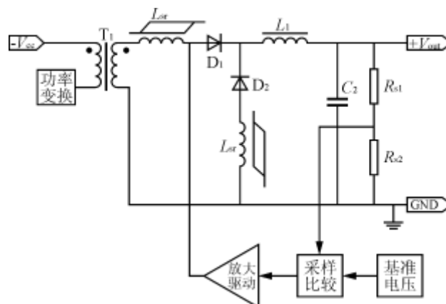
图6 磁放大输出稳压电路
