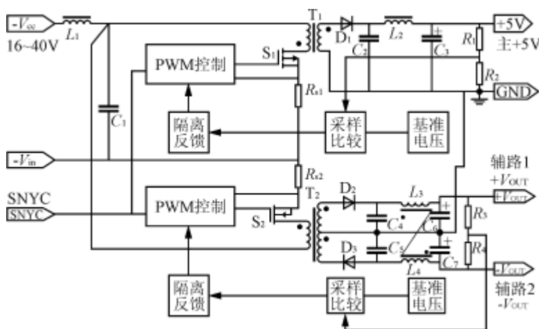
图5 3路电源设计方案
