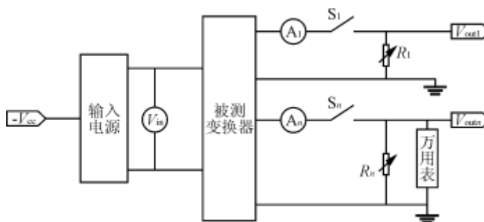
图2 测试仪表及设备连接
