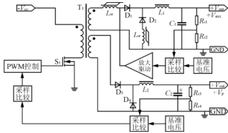
图7 辅路带磁放大器的典型应用电路
