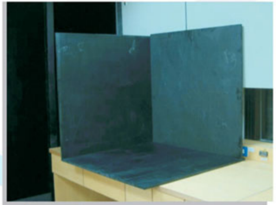
燈具產品專用的測試角落 (法規IEC/EN 60598)
