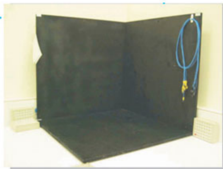
家電產品專用的測試角落 (法規: IEC/EN 60335)
