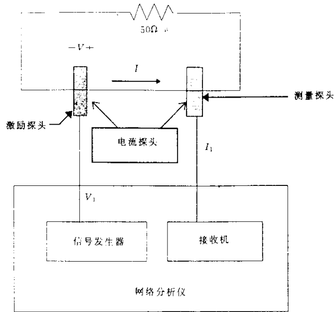
图 C5 校准示意图
