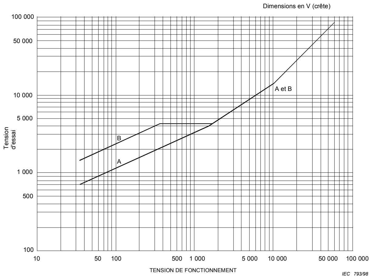
Figure 7 – Tensions d'essai
