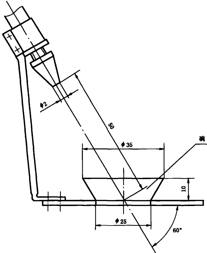
图 101 溅水装置
