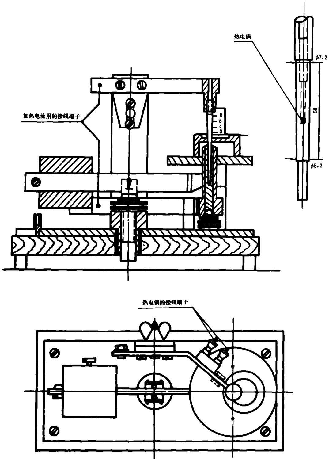
图 9 热轴试验器
