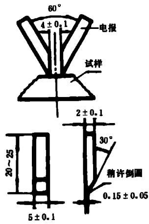
图 10 抗漏电痕迹试验的电报布置和尺寸
