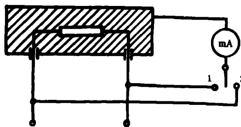
图 4 非 II 类的工具在工作温度下测量泄漏电流的单相联接图
