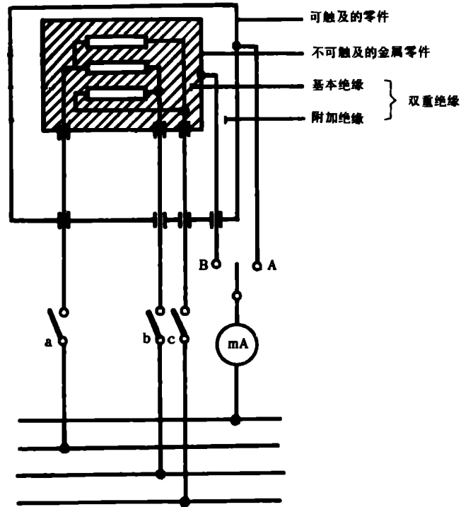
图 5 I 类工具在工作温度下测量泄漏电流的三相联接图
