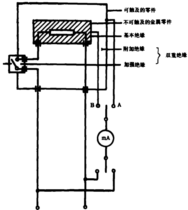
图 3 II 类工具在工作温度下测量泄漏电流的单相联接图
