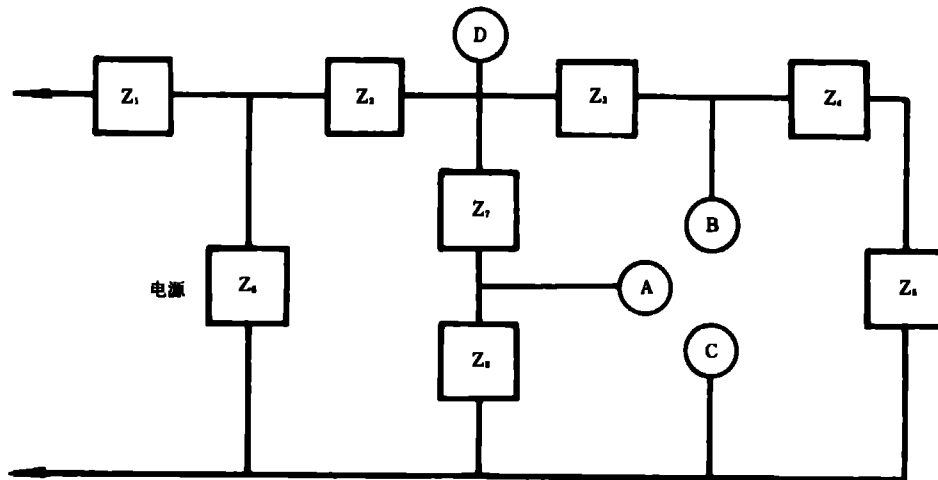
图 C1 带低功率点的电子线路的例子
