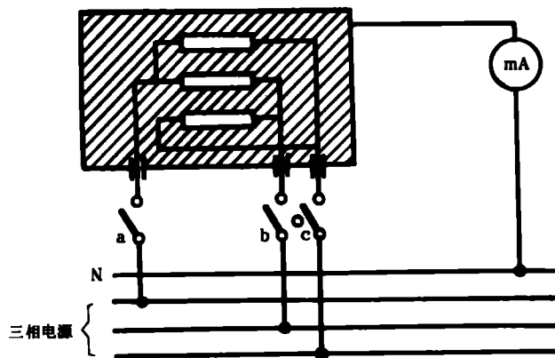
图 6 非 I 类的工具在工作温度下测量泄漏电流的三相联接图
