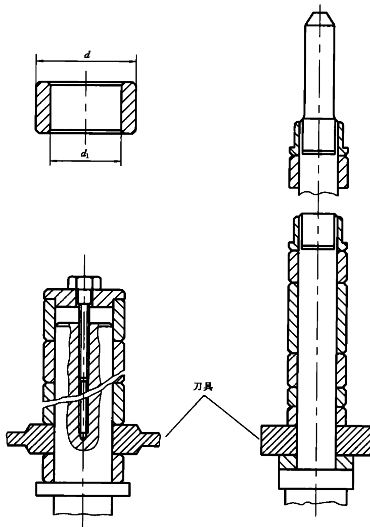
图 102 刀夹轴和轴套
