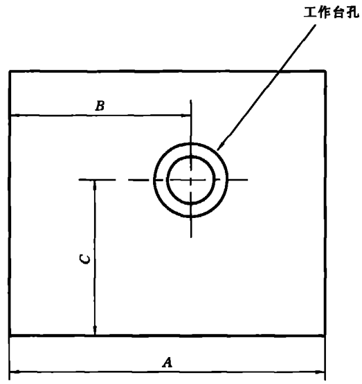
图 104 工作台尺寸
