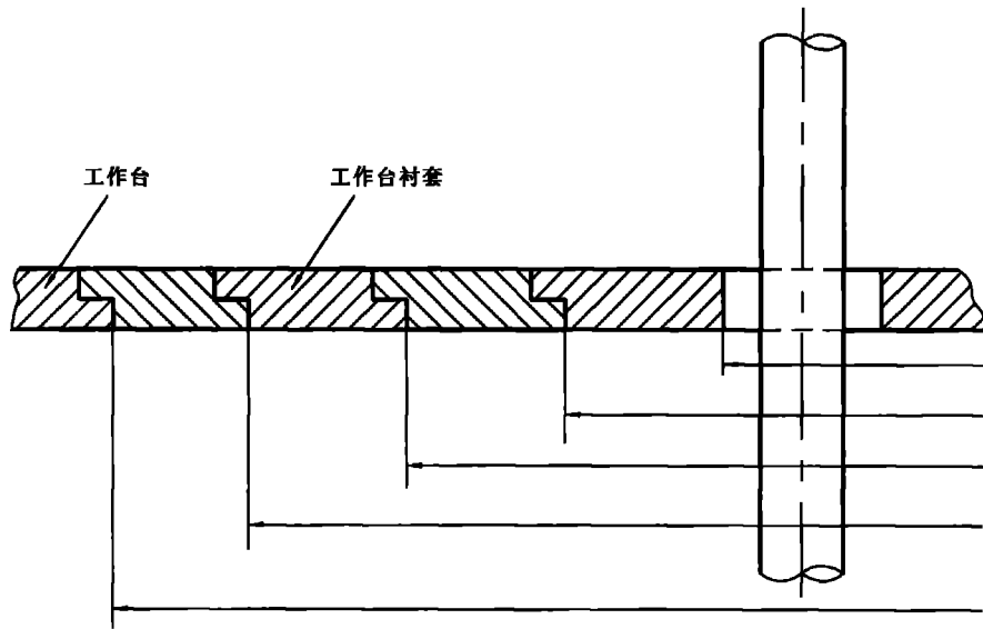
图 104 工作台尺寸
