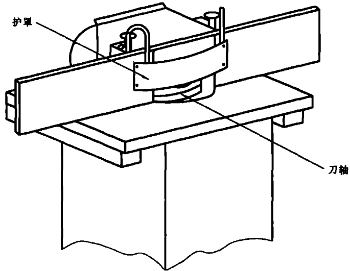
图 108 开棒时的工件导向器和刀轴防护系统
