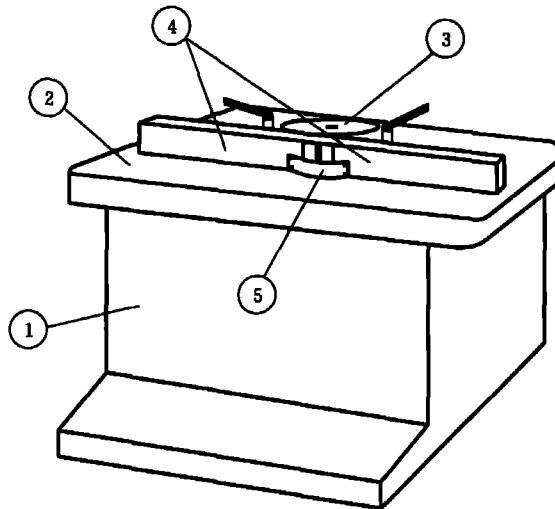
1—基座；2—工作台；3—刀轴；4—平行导向器；5—刀轴护罩
