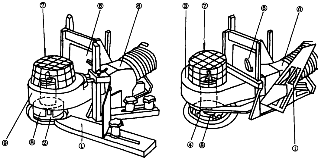
1—导向器的导引板；2—滚道导向；3—手防护罩；4—固定导向器； 5—支架；6—排屑口；7—帽形护罩；8—刀轴
