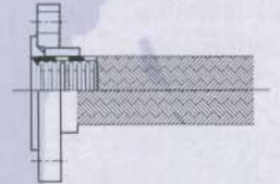
无接管活法兰联接型
