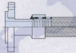
活法兰联接型
