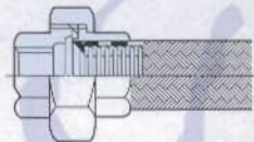
油令内锥螺纹联接型
