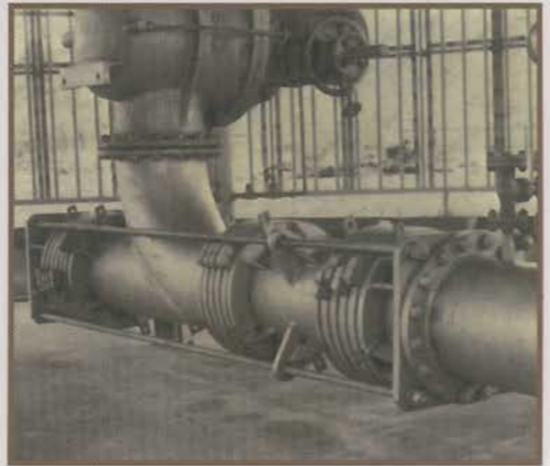
曲管压力平衡型补偿器应用
