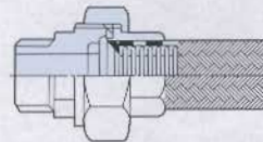
油令外锥管螺纹联接型
