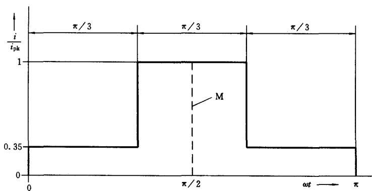
图1 定义“特殊波形”并将设备分类为D类的输入电流包围线 可利用图2的流程图来确定设备的类别。
