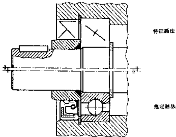
图 13 角接触球轴承在装配图中的画法
