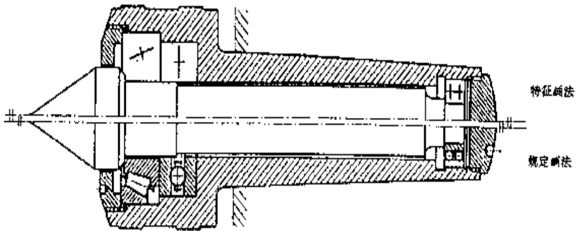
图 15 组合轴承在装配图中的画法
