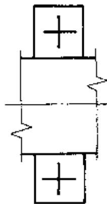
图 2 滚动轴承带附件的剖面线画法
