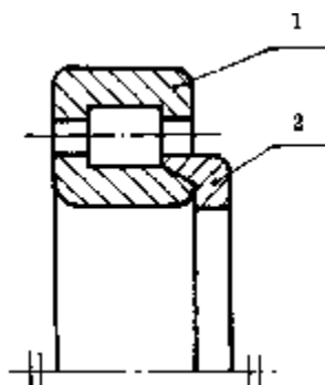
1—圆柱滚子轴承(GB/T 283); 2—斜挡圈(JB/T 7917)
