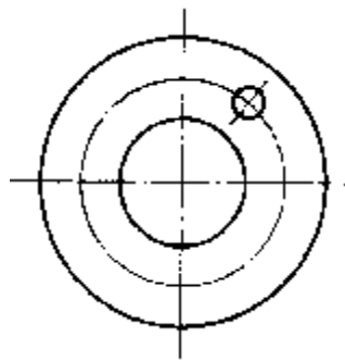
图 11 滚动轴承轴线垂直于投影面的特征画法
