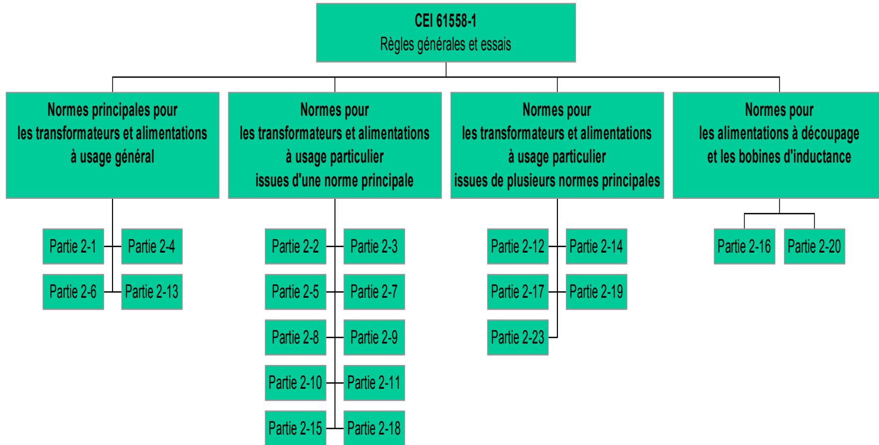
Figure 0 – Principe de la CEI 61558
