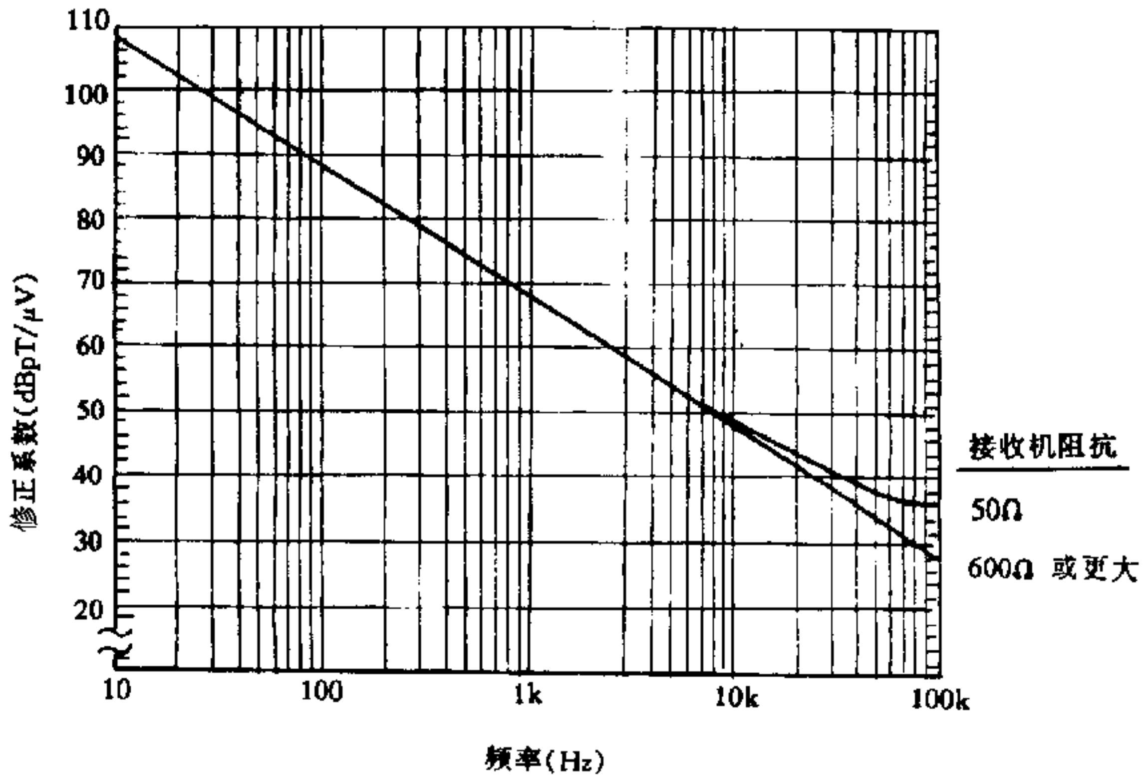
图 RS101-1 环状传感器修正系数
