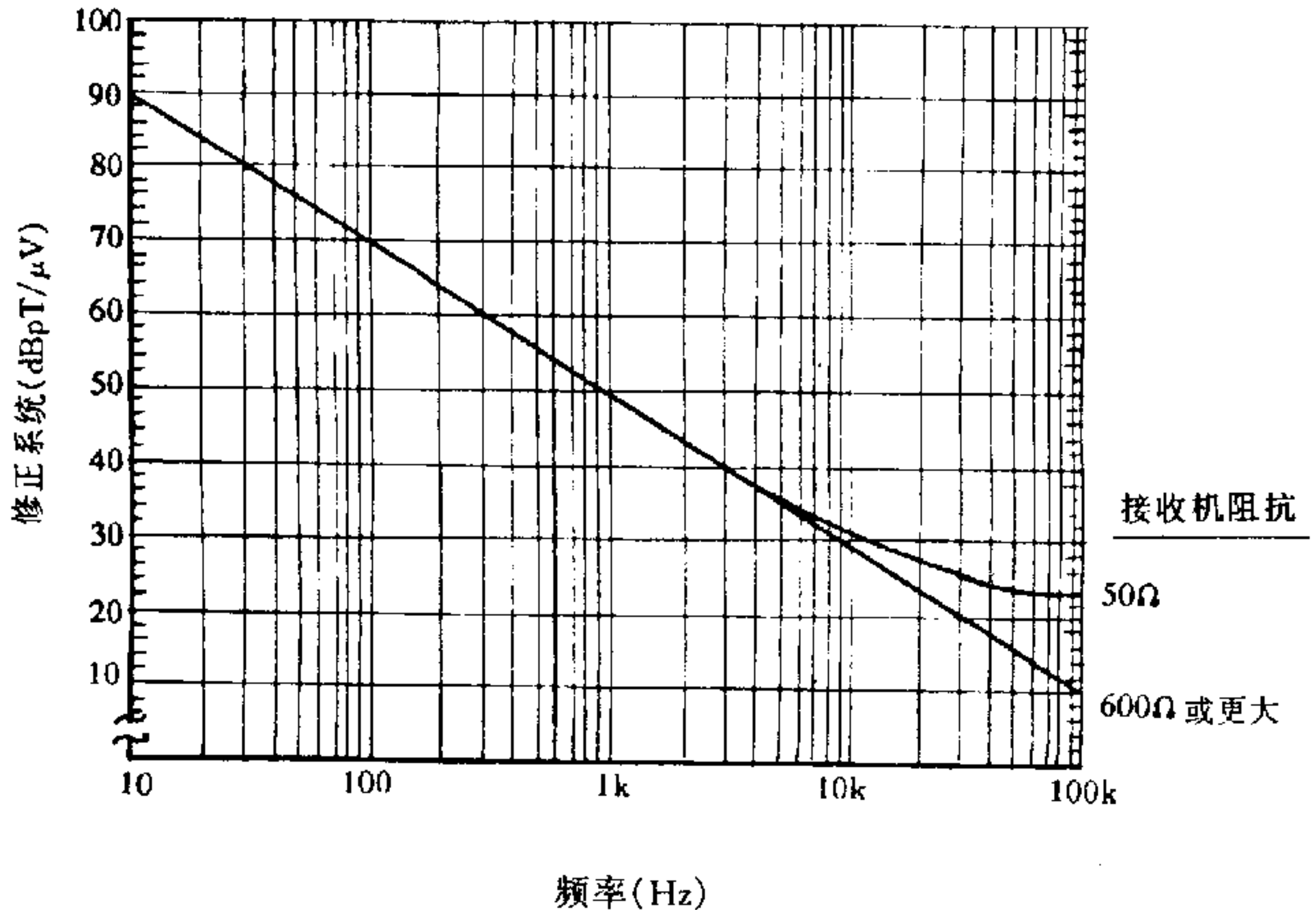
图 RE101-1 环状传感器修正系数
