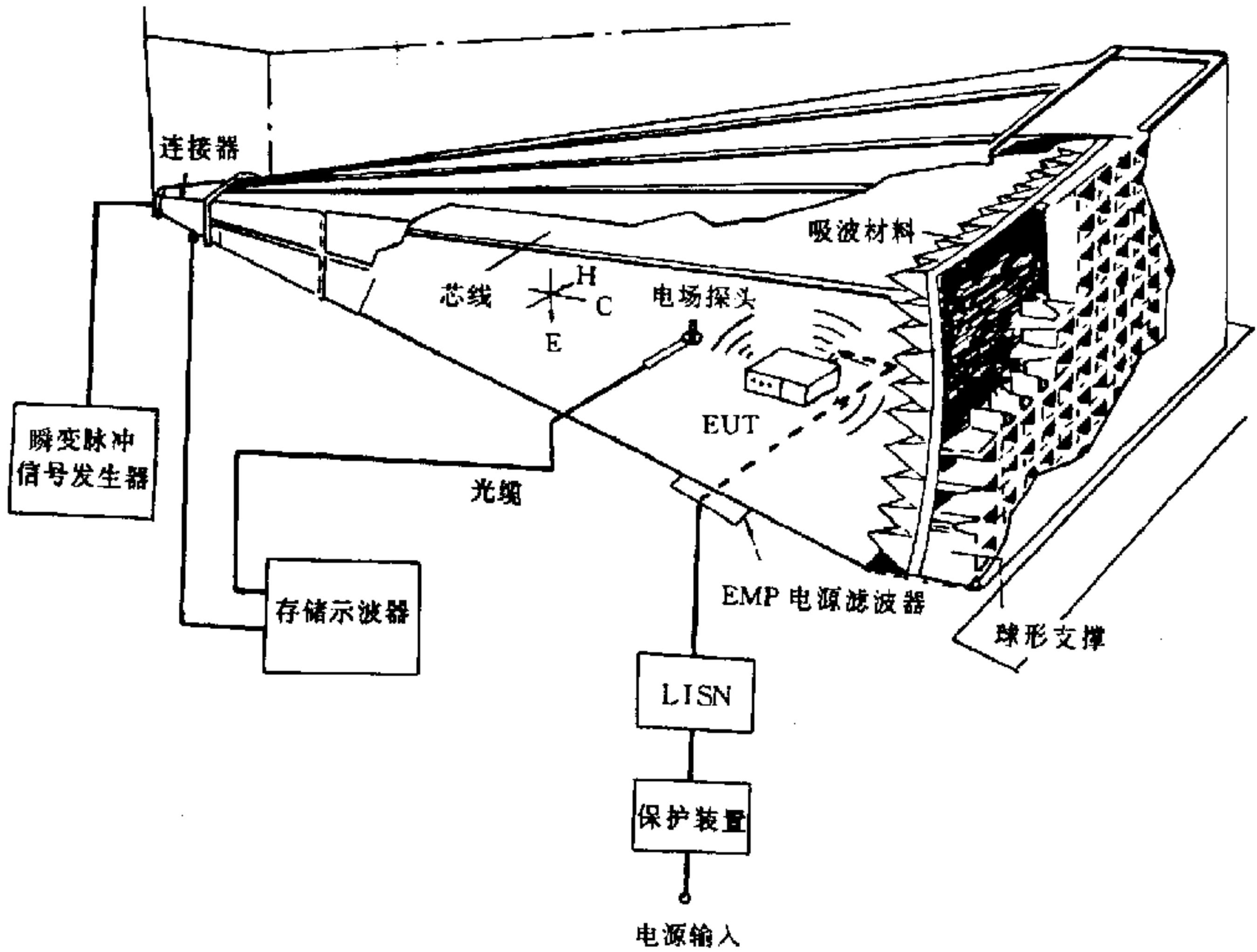
图 RS105-3 采用 GTEM 装置典型测试配置
