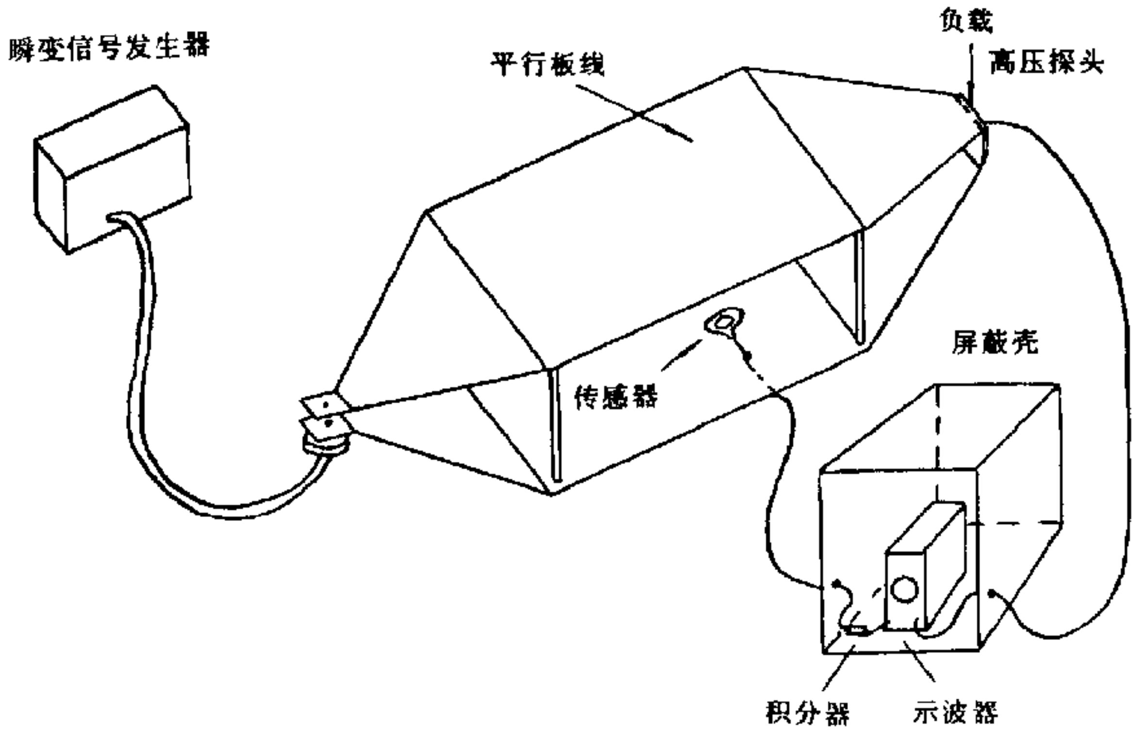
图 RS105-2 采用平行板辐射系统典型校准配置
