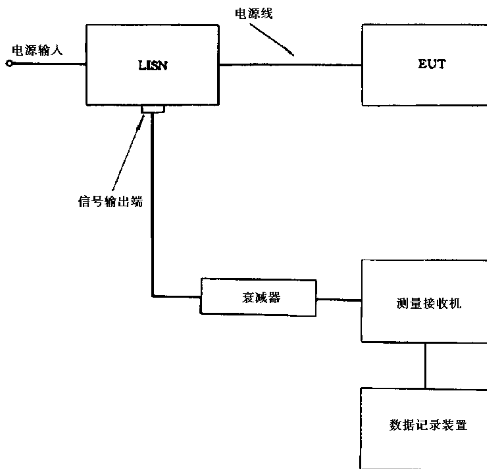
图 CE102-2 测量配置图
