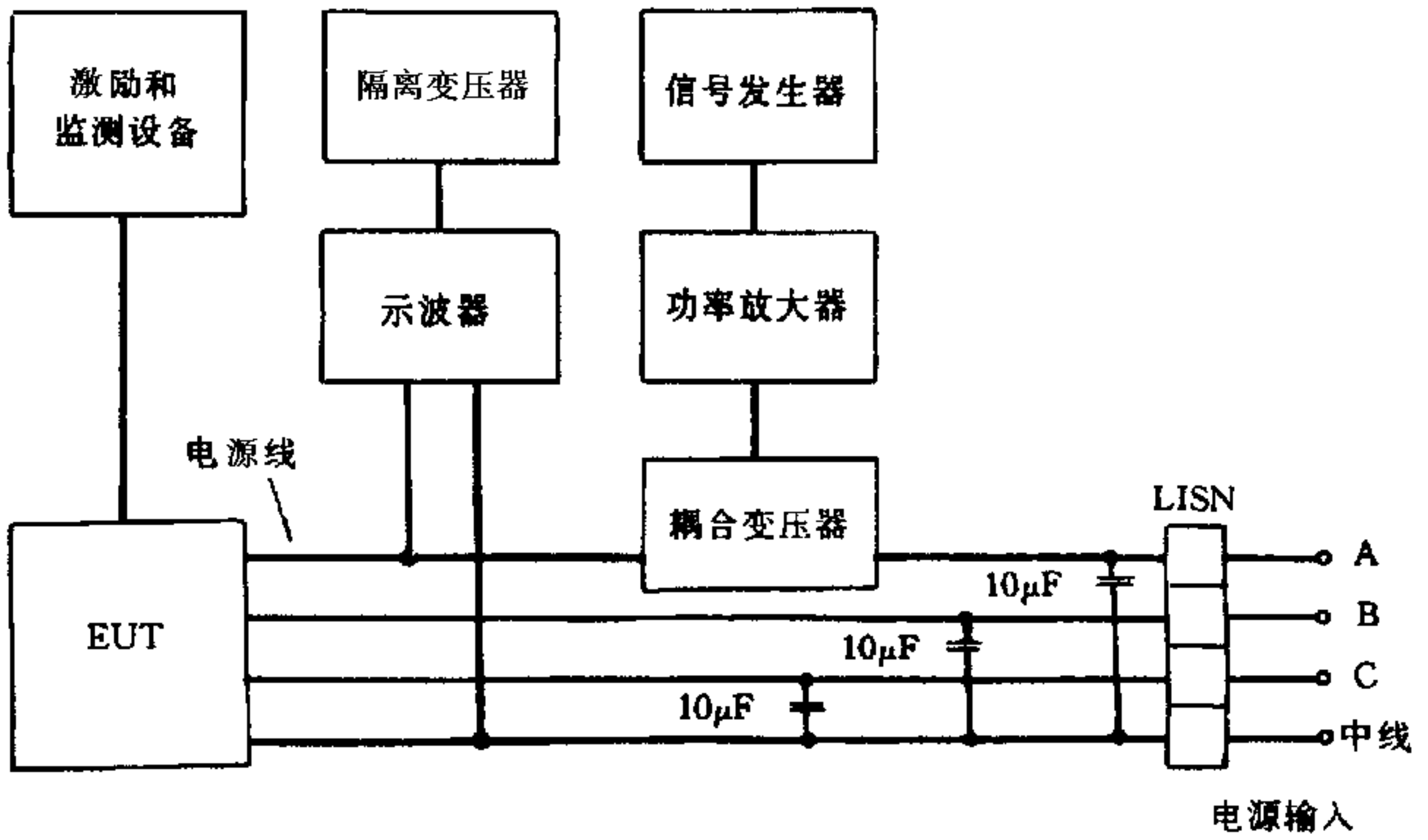
图 CS101-4 三相 Y 型电源线信号注入
