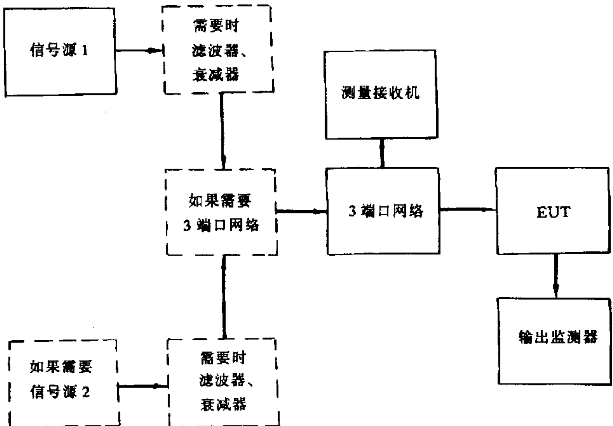
图 CS104 通用测试布置
