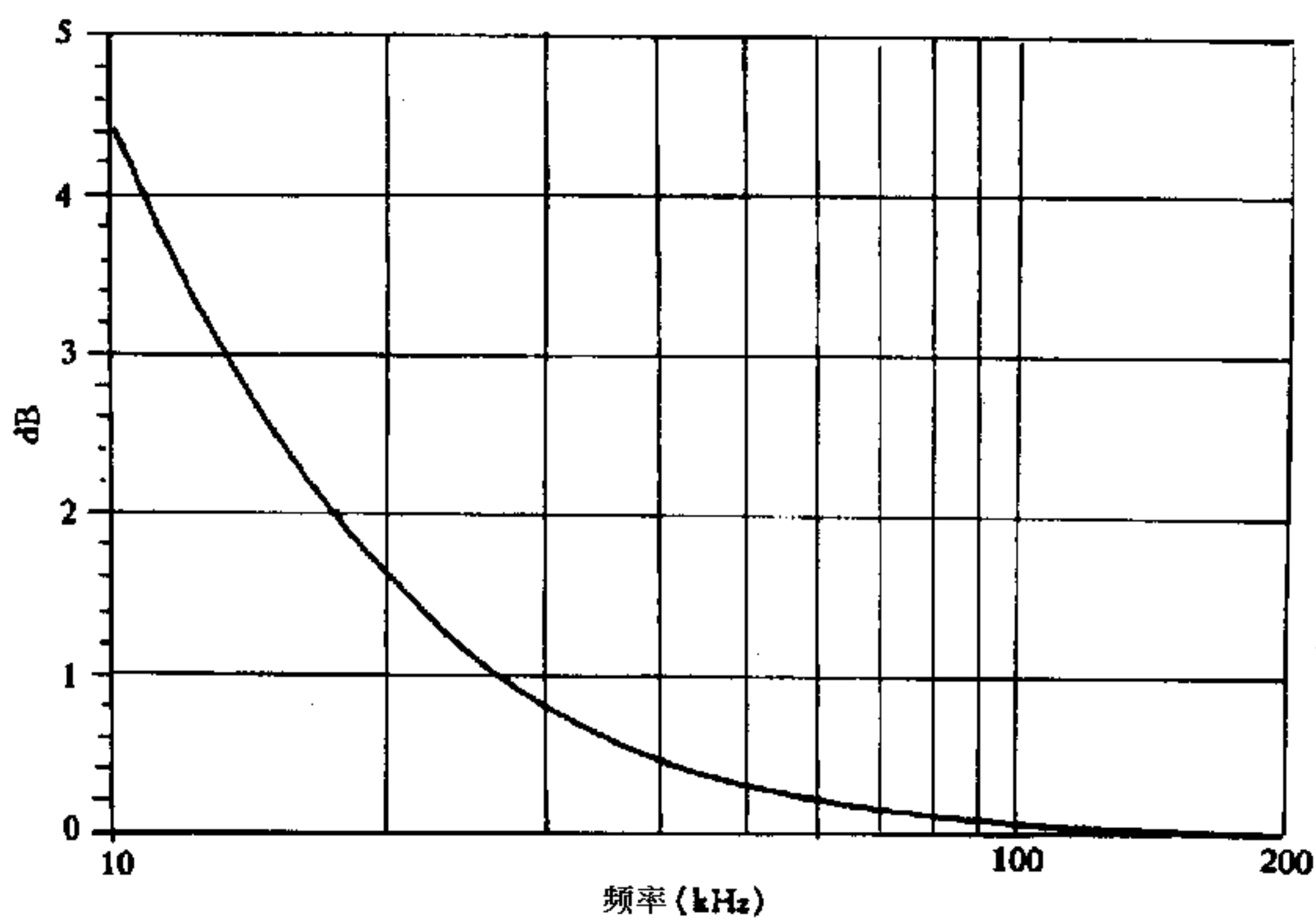
图 CE102-3 LISN0.25 \mu F 耦合电容修正系数
