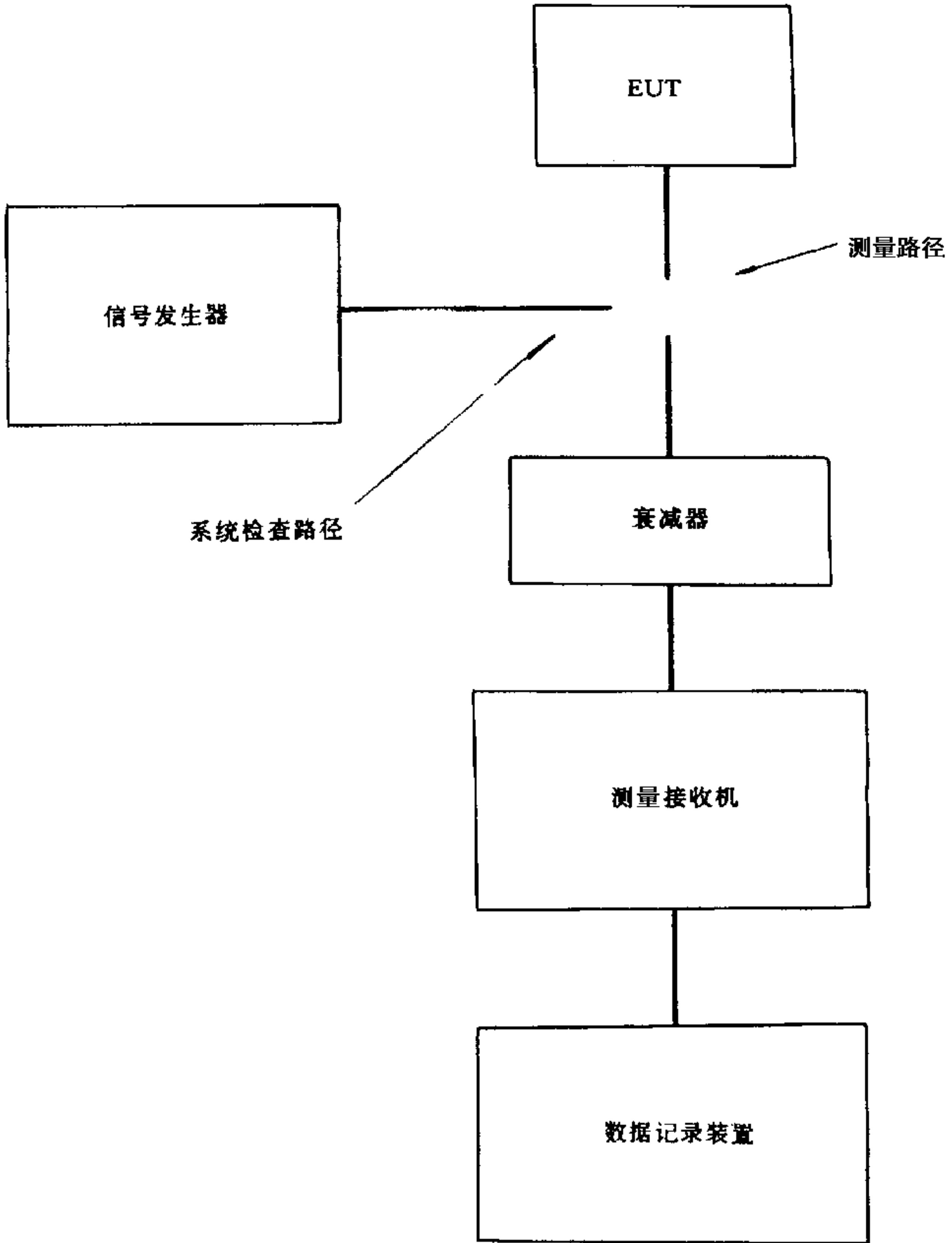
图 CE106 -3 发射机(待发状态)和接收机测试配置
