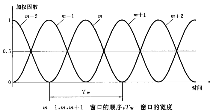
图 B2 汉宁时间窗的外形和排列
