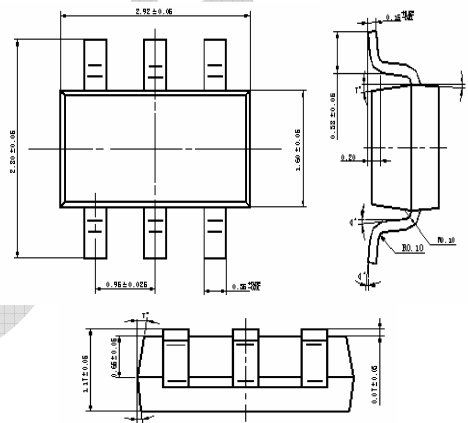
图 8 SOT23-6 封装外形尺寸
