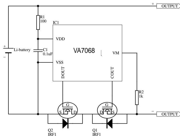
图 3 VA7068 典型应用线路图
