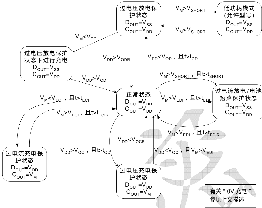
图 4 VA7068 各状态之间的转换图
