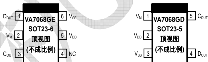
图 2 VA7068 引脚排列
