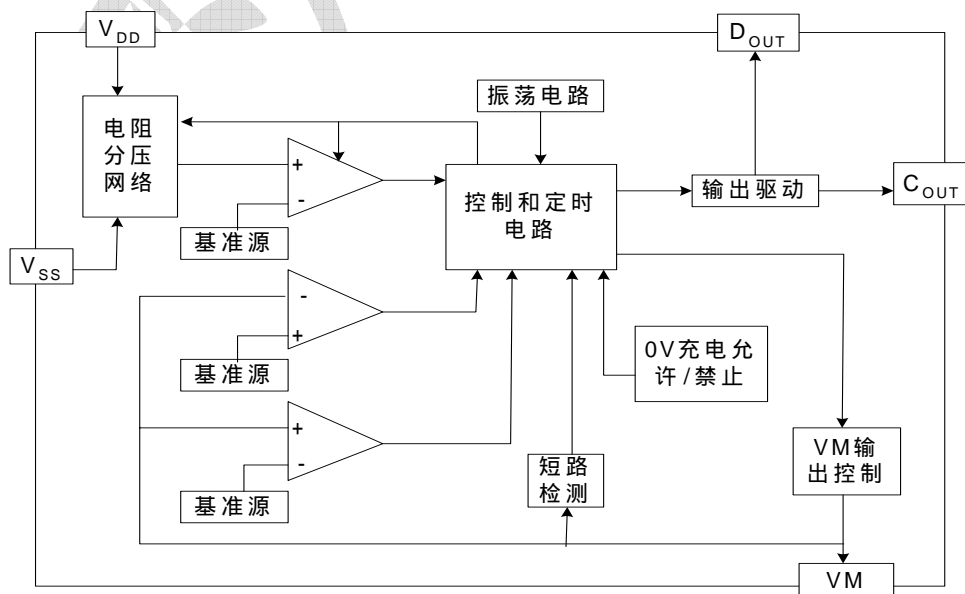
图1 VA7068 功能框图
