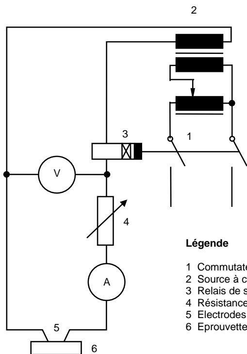
Figure B.4 – Exemple de circuit d'essai
