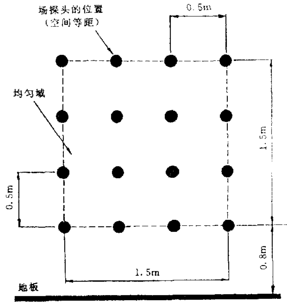
图4 场校准,均匀场的尺寸
