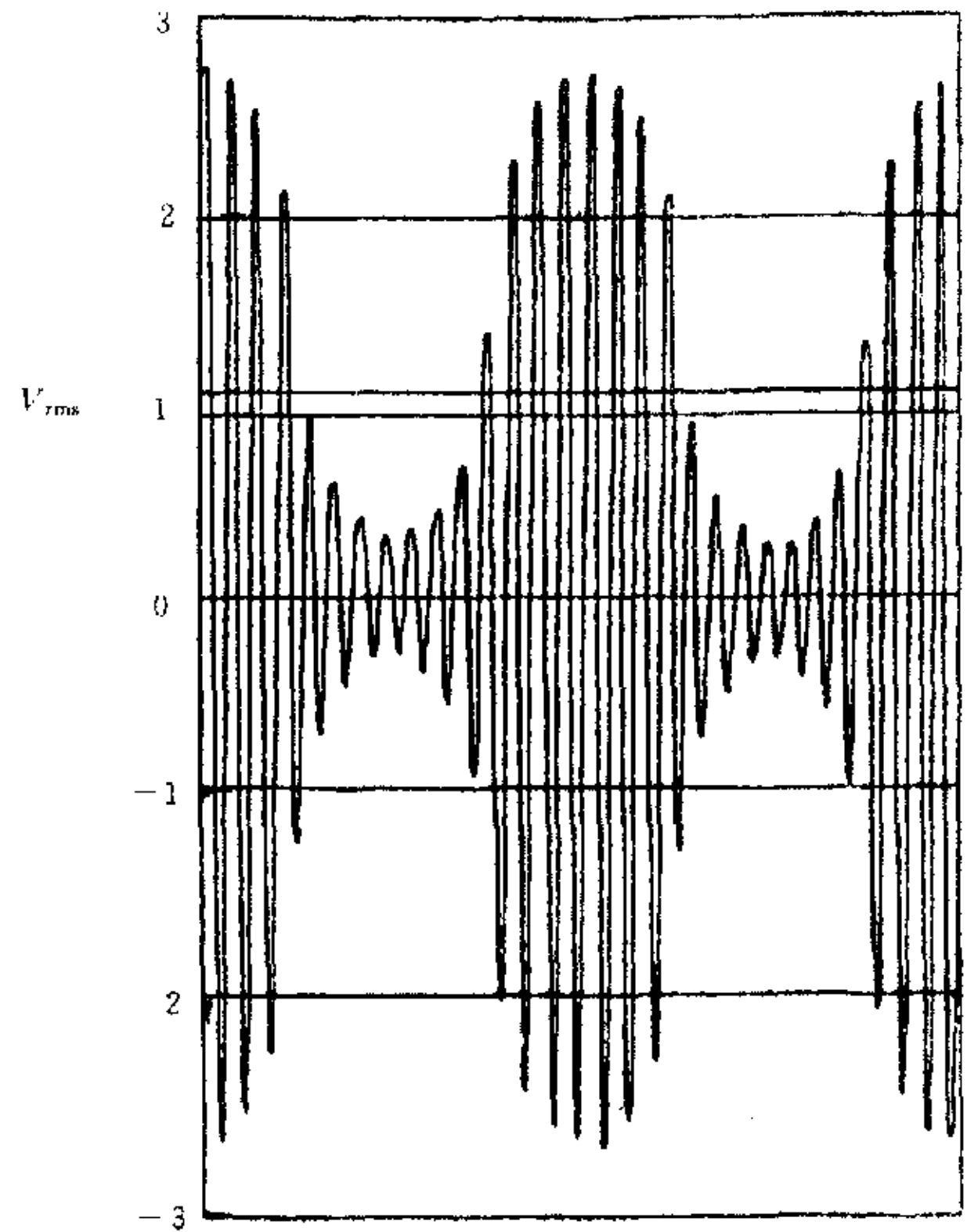
b) 80%幅度调制的 RF 信号
