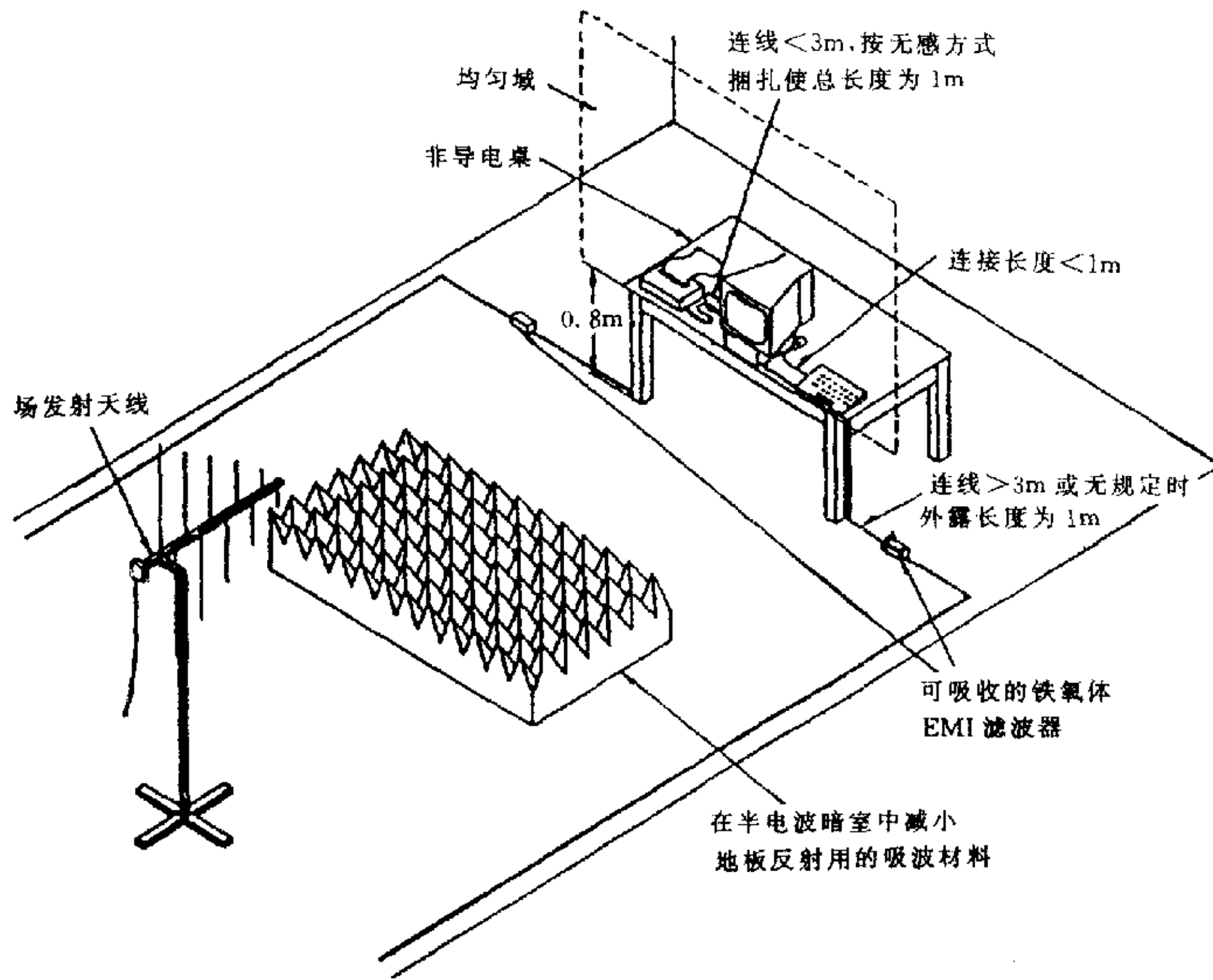
图 6 台式设备的试验布置举例
