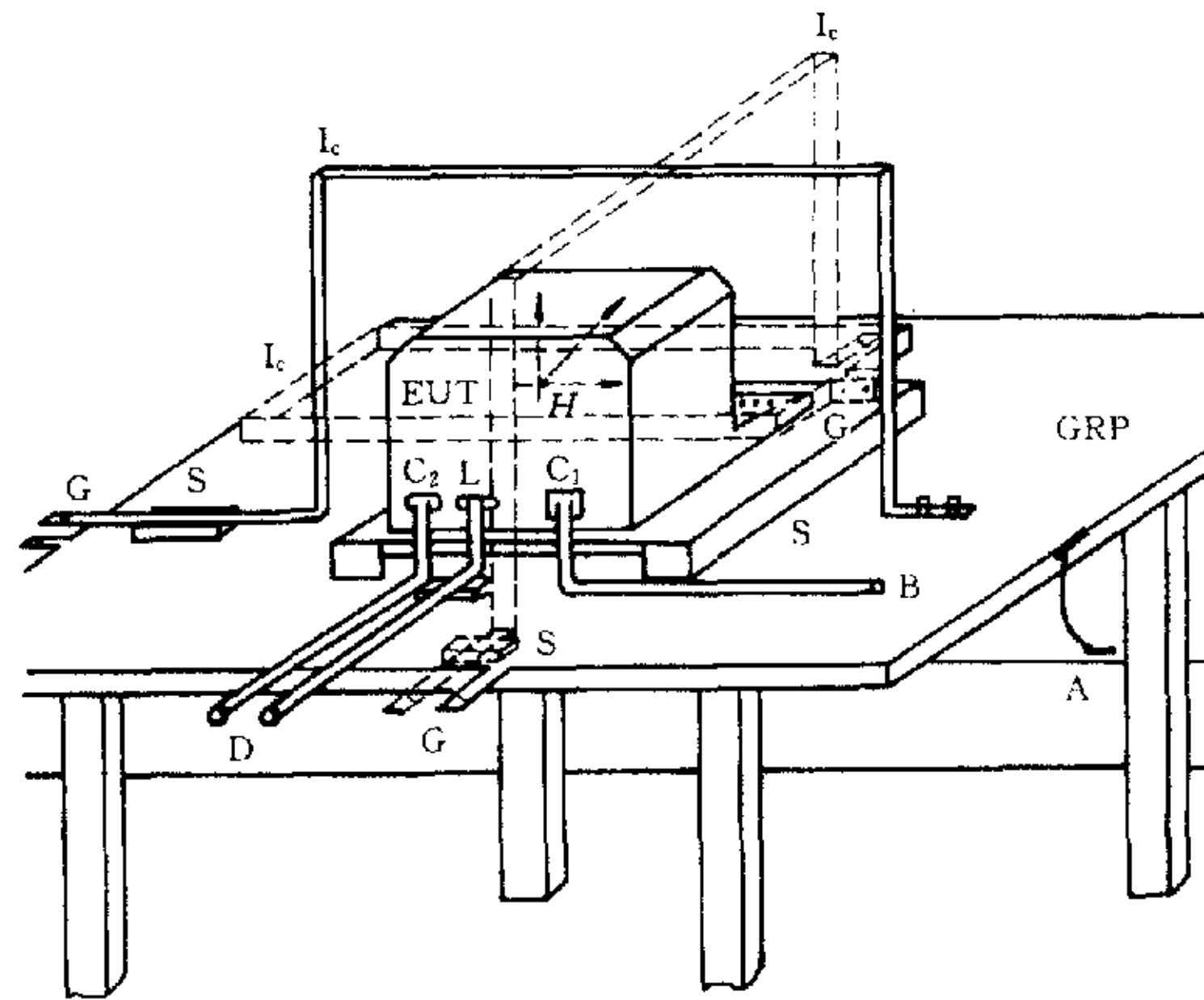
图3 台式设备的试验布置
