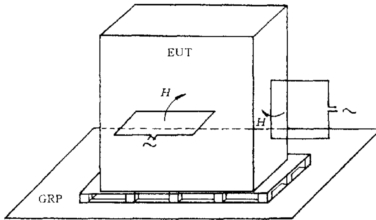
图 5 用邻近法探测磁场敏感性
