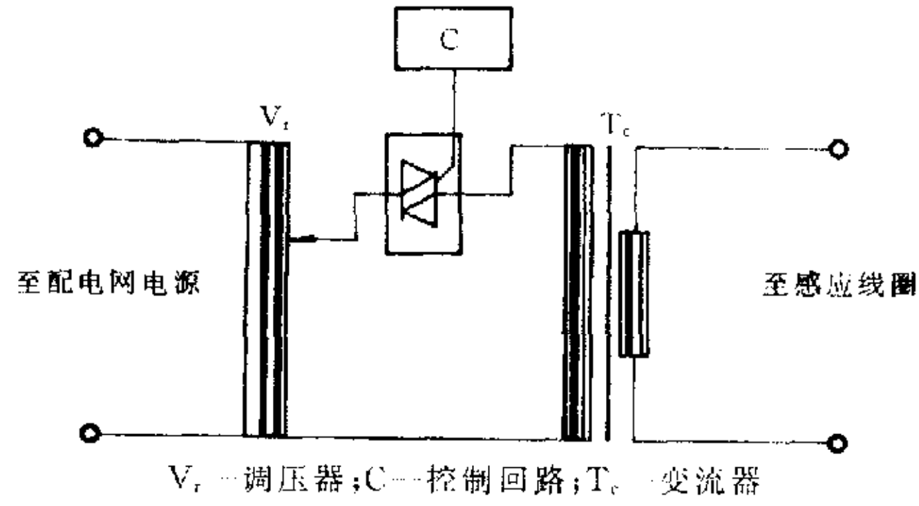
图2 工频磁场试验发生器的原理图
