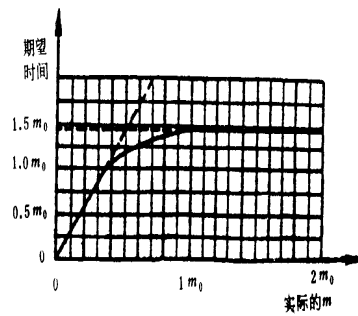
图 40 试验方案 5 : 7 判定的期望相关试验时间
