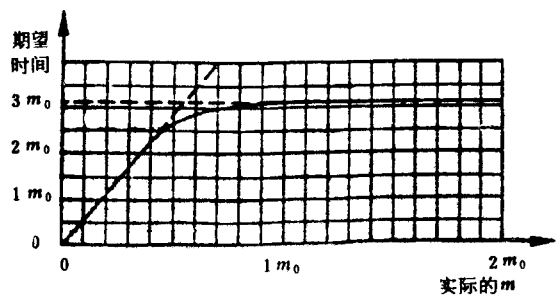
图 35 试验方案 5:3 判定的期望相关试验时间
