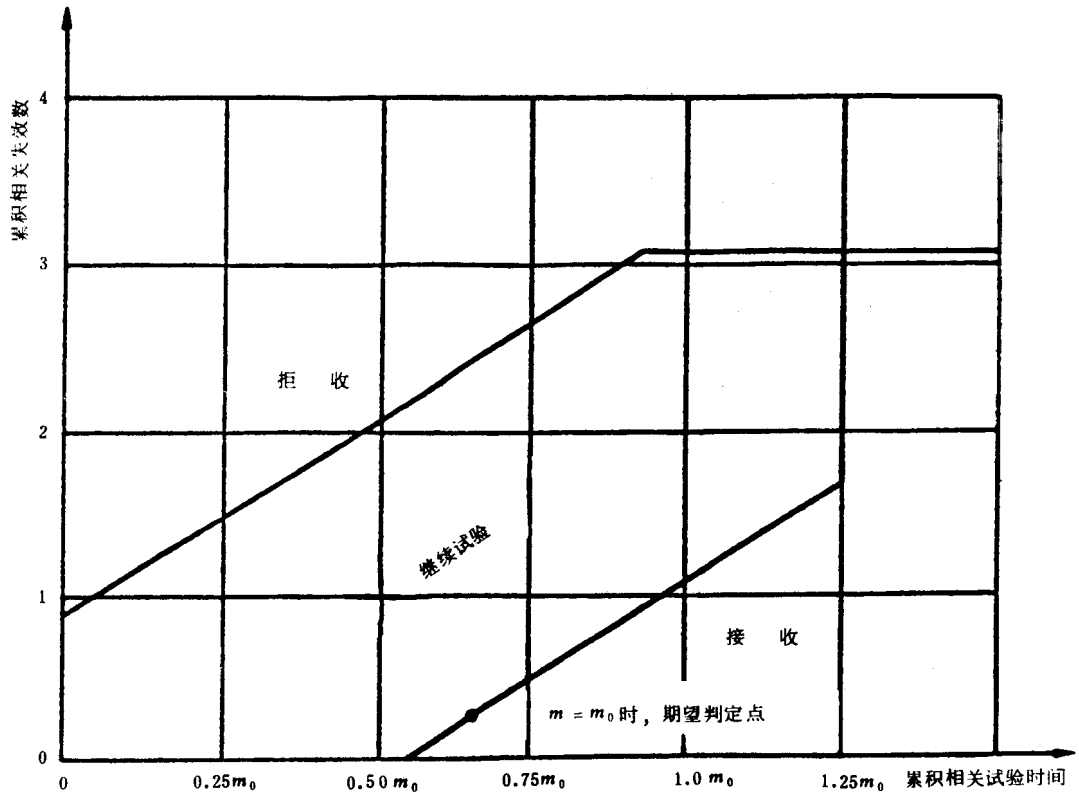
图 11 试验方案 4 : 4 ( \alpha=0.10, \beta=0.10, D_m=5.0 )
