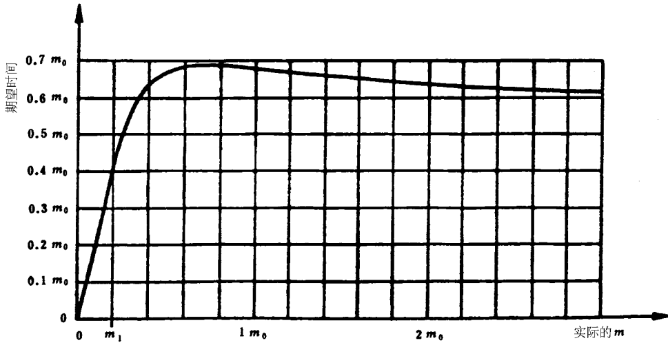
图 12 试验方案 4 : 4 工作特性曲线
