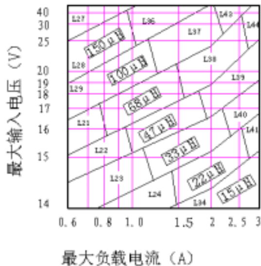
图6 LM2596 —12
