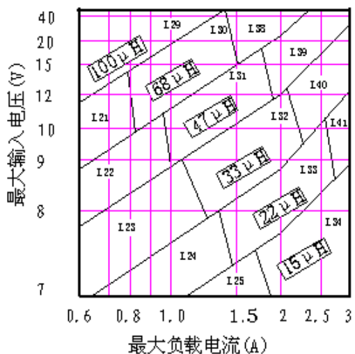
图5 LM2596 —5.0
