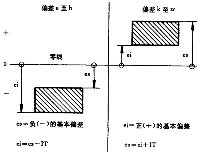
图 1 轴的偏差
