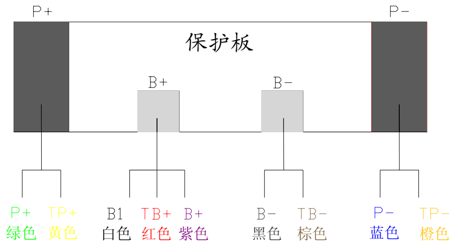
单节保护板测试连线图
