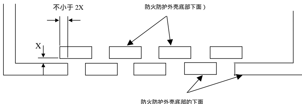
图 4F 挡板结构
