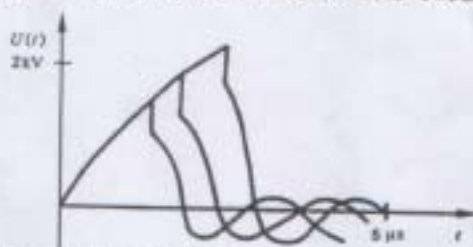
图 S1 不带电涌抑制器而且绝缘未击穿时的波形
