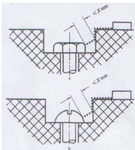
图 F7 带窄沟槽和宽沟槽的未粘合接缝
