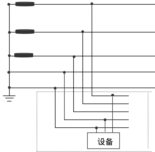
单独的中线和保护接地线
