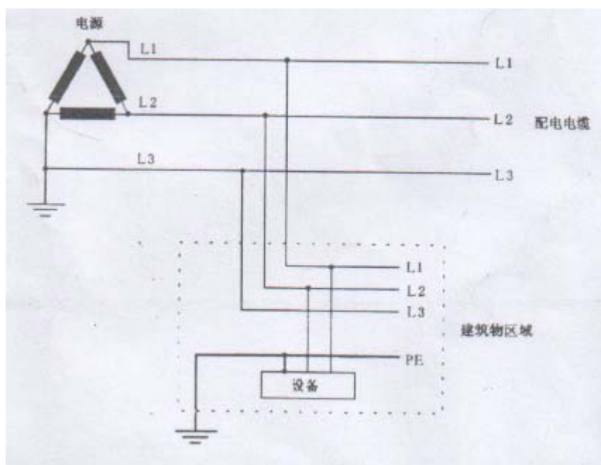
接地的相线和设备上独立的接地线
