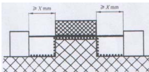
图 F5 带窄沟槽的未粘合接缝
