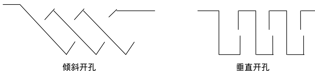
图 4B 防止垂直进入的开孔截面结构设计实例
