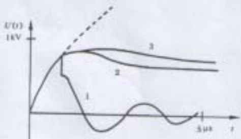
图 S2 不带电涌抑制器绝缘击穿时的波形
