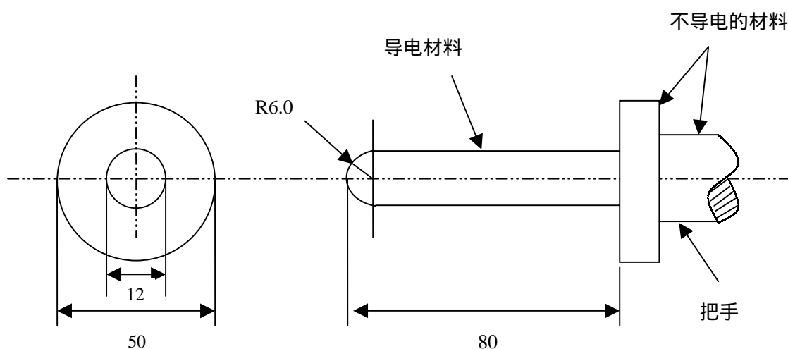
图 2C 试验探头
