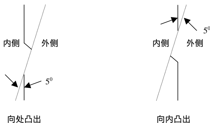
图 4C 百叶窗结构实例
