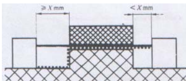
图 F6 带宽沟槽的未粘合接缝
