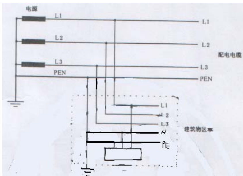
图 V2 TN-C-S 配电系统实例
