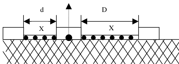
图 F12 绝缘材料外壳的测验实例
