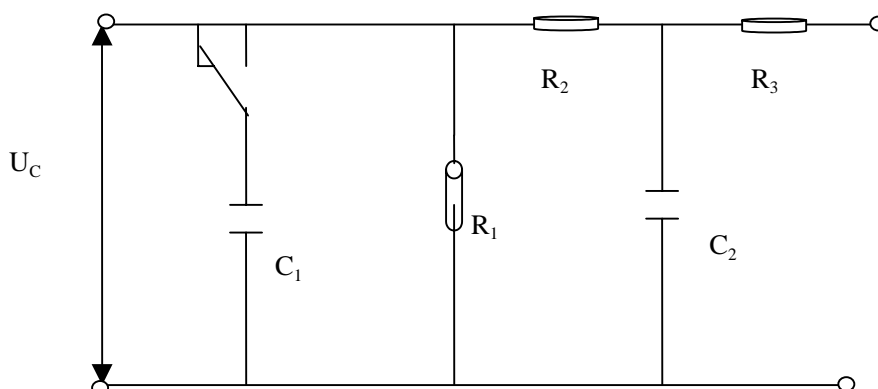
图 N1 脉冲发生电路
