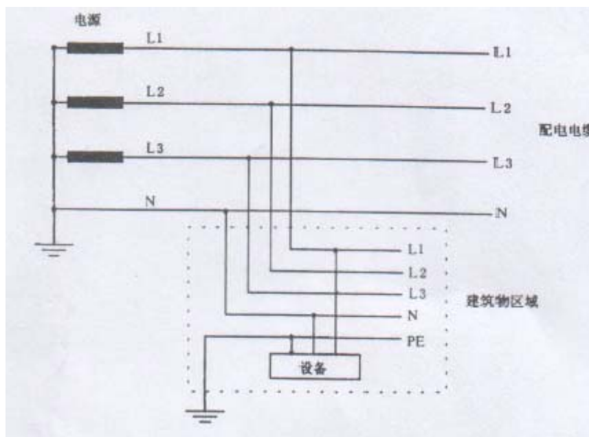
接地的中线和设备上独立的接地线
