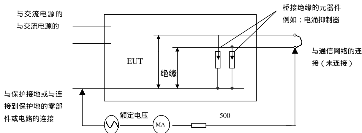
图 6A 通信网络和地之间的隔离试验
