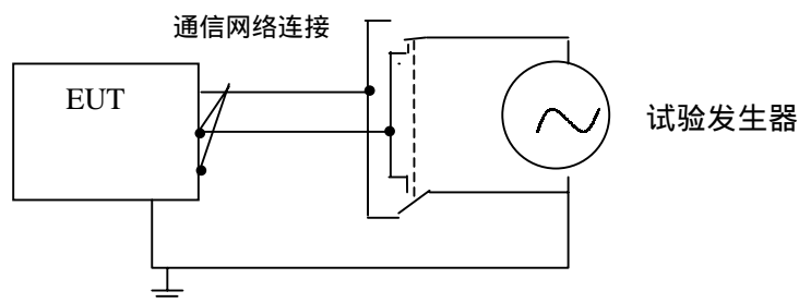
图 2E 试验电压发生器
