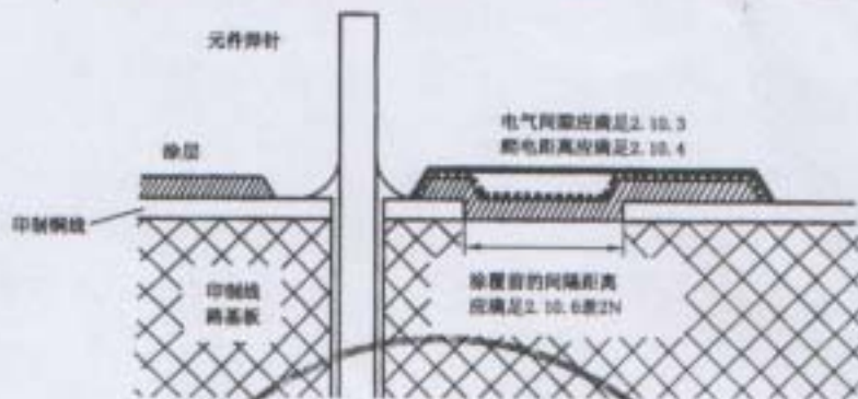
图 F11 印制电路板上的涂层
