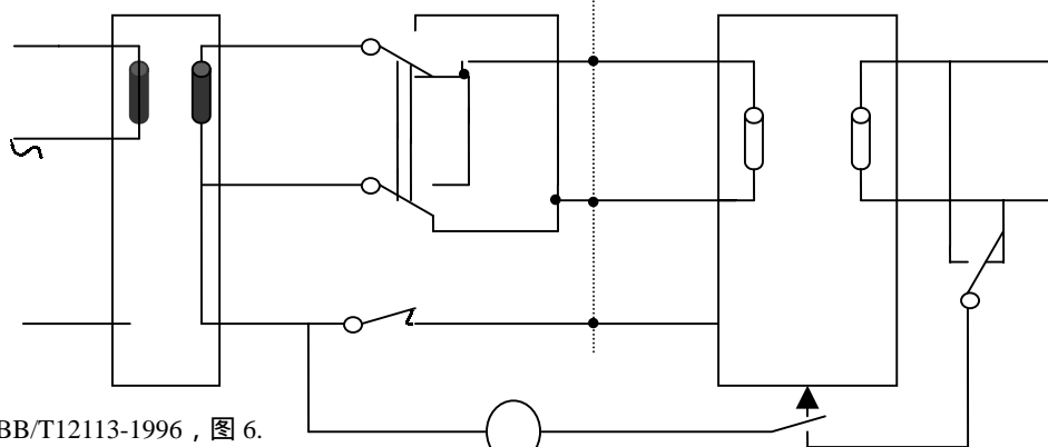
图 5A 接到星形 TN 或 TT 配电系统的单相设备接触电流试验电路
