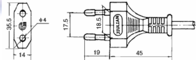
RVVZ-2Y
