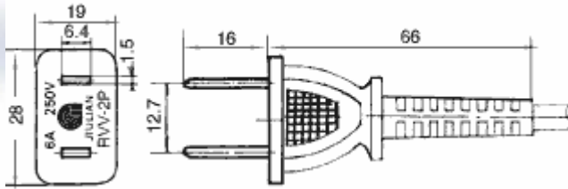
RVV-2P
