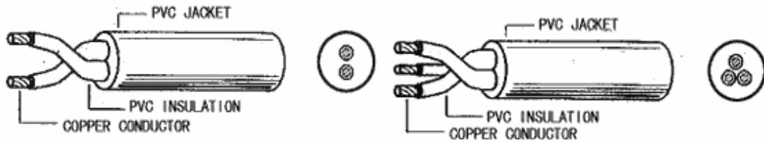
H03VVH2-F & H03VV-F
