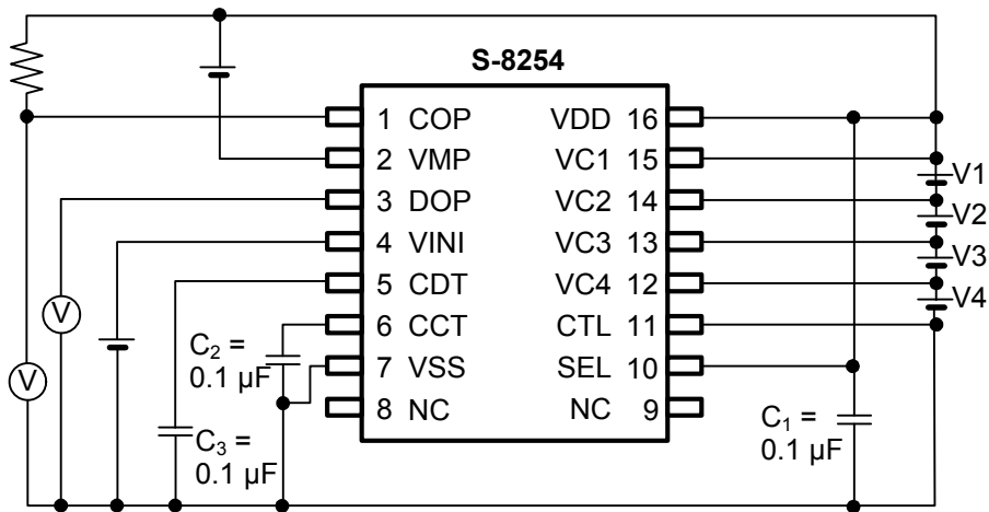
图5 测定电路3
