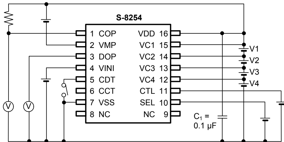
图4 测定电路2
