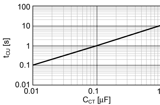
2.11 t_{CU} - C_{CT}
