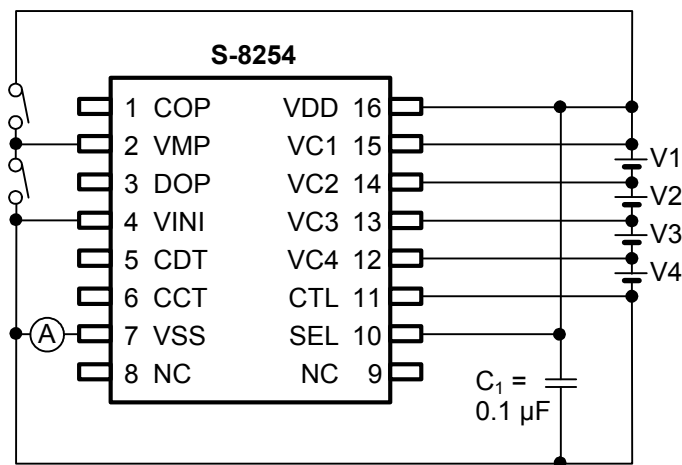
图3 测定电路1
