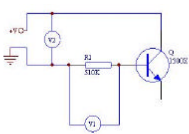
(图1)VCBO测试: 观察V1有变化时记录V2数值.
