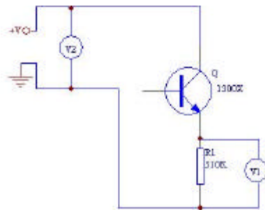
(图2)VCEO测试: 观察V1有变化时记录V2数值.
