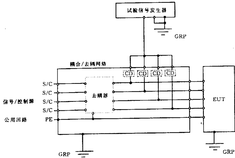
a) 由参考接地板实现的配置(参见 7.1.1)
