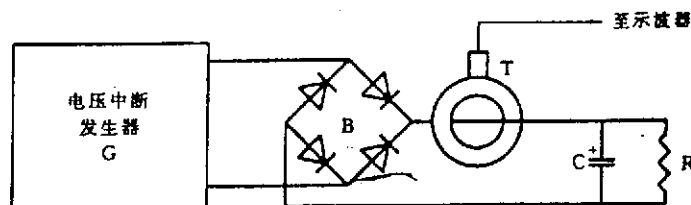
G—电压中断发生器,在 90^\circ 和 270^\circ 上转换;T—电流探头,可输出给示波器来监视;B—整流桥;R—分流电阻器, 100\ \Omega R \leq 10\ 000\ \Omega ; C— 1\ 700\ \mu\text{F} \pm 20\% 的电解电容器
