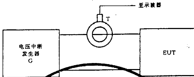
图 A2 确定 EUT 的峰值冲击电流要求的电路
