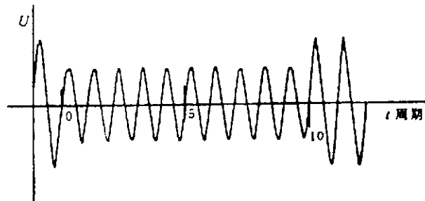
图 1 电压暂降
