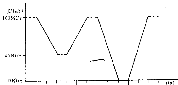
图 1 电压暂降
