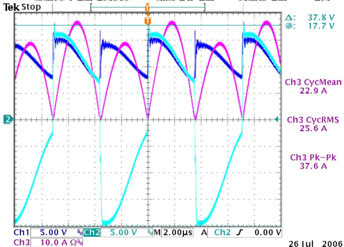
12V20A 低壓側的電壓電流波形 CH1:輸出電容電壓 CH2:變壓器電壓 CH3:電流
