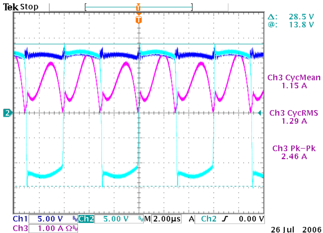
12V1A 低壓側的電壓電流波形 CH1:輸出電容電壓 CH2:變壓器電壓 CH3:電流
