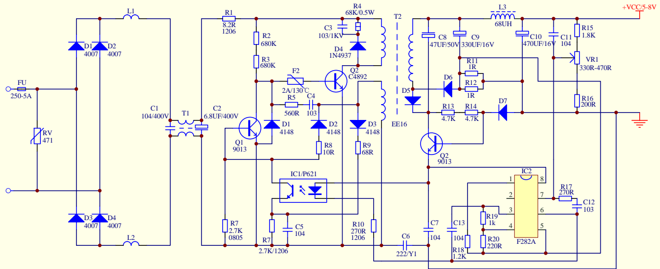
此图由日本MITSUMI公司为三洋生产的手机充电器剖析图，经测试，输出电压可调，将输出电压调至5V，输出电流1A（短路过流取样电阻）时电压还很稳定，可是将次级输出部分改为431组成的常规电路后，却无法正常工作，烧机。
