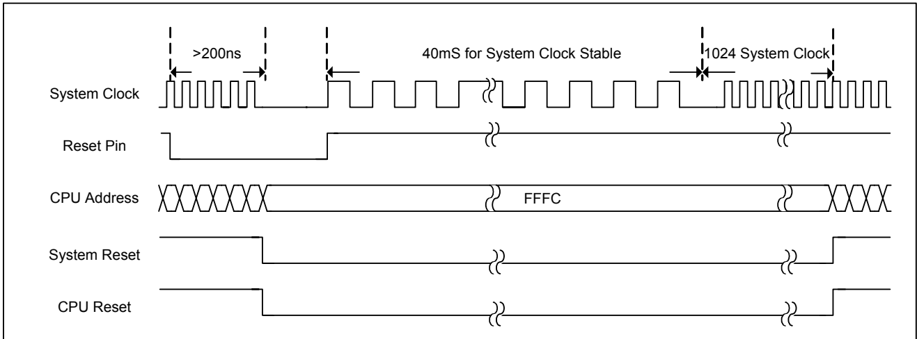
图 5-17 外部复位时序
