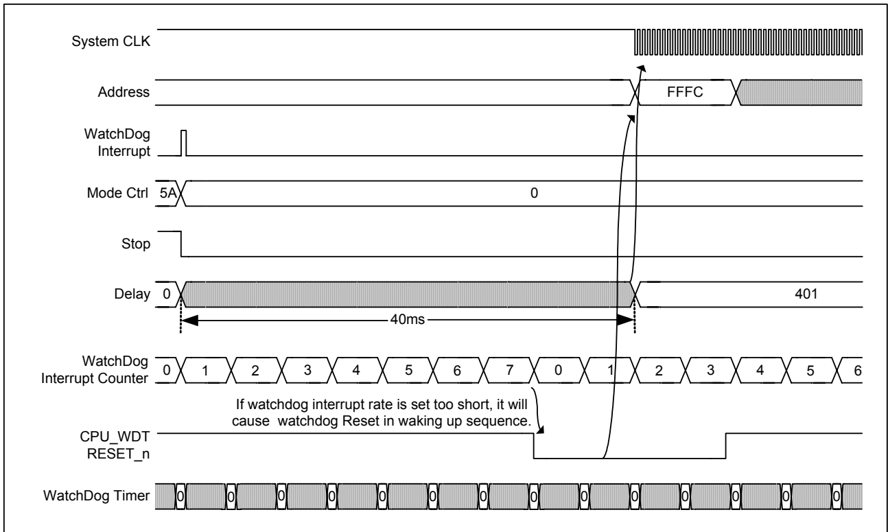
图 5-10 看门狗计数的溢出频率过快，唤醒 STOP 模式失败的时序
