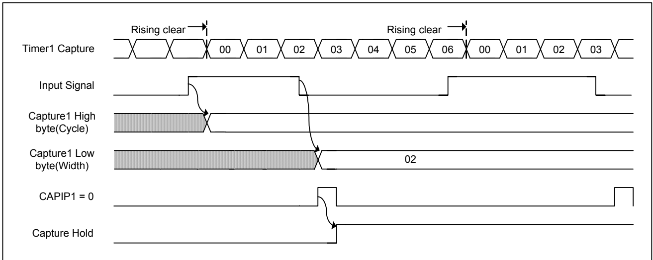
图 5-30 8 位捕获及数据保持的工作时序
