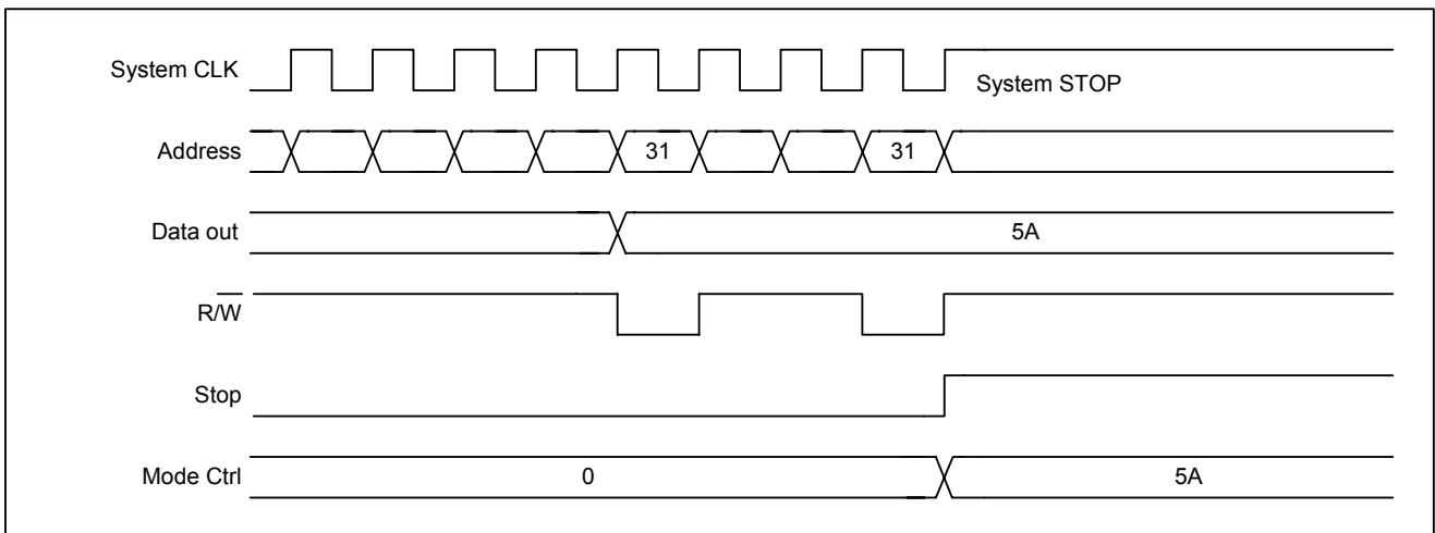
图 5-8 进入 STOP 模式的时序
