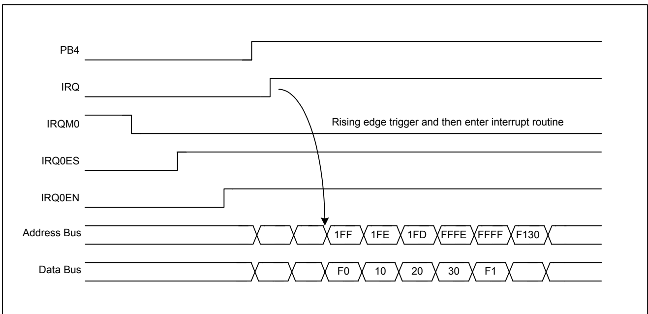
图 5-13 IRQ0 中断触发时序图(PB4)
