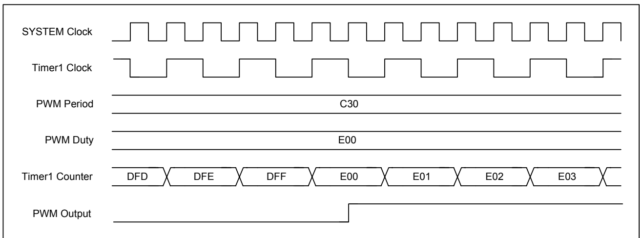
图 5-34 12 位 PWM 输出波形的翻转时序
