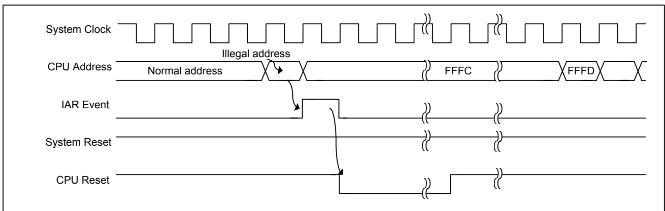
图 5-20 非法地址复位时序
