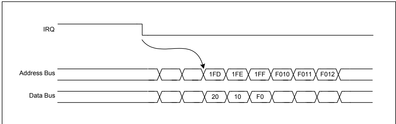
图 5-14 中断退出时序图
