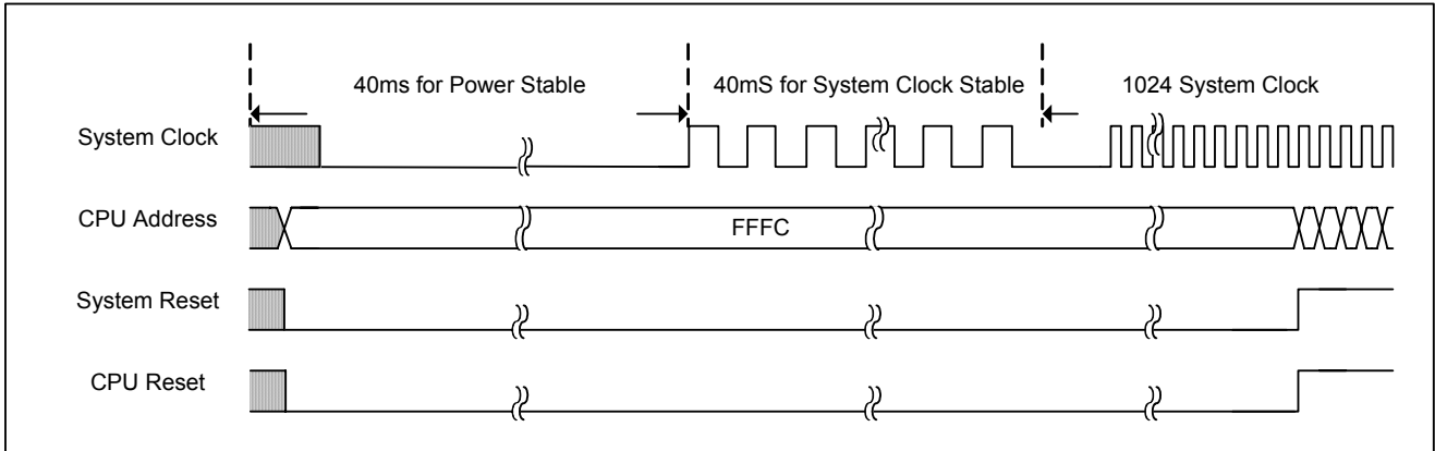
图 5-16 上电复位时序
