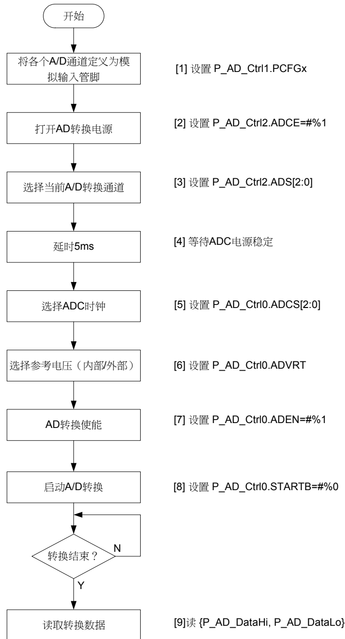
图 5-36 A/D 转换流程
