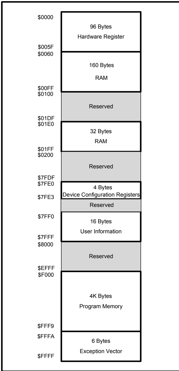
图 5-4 SPMC65P2204A 存储空间分配图
