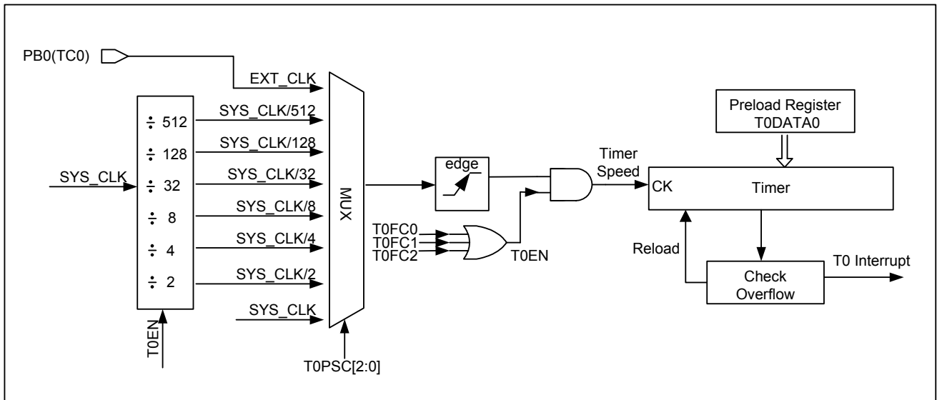
图 5-22 8 位定时/计数器 0 的内部结构
