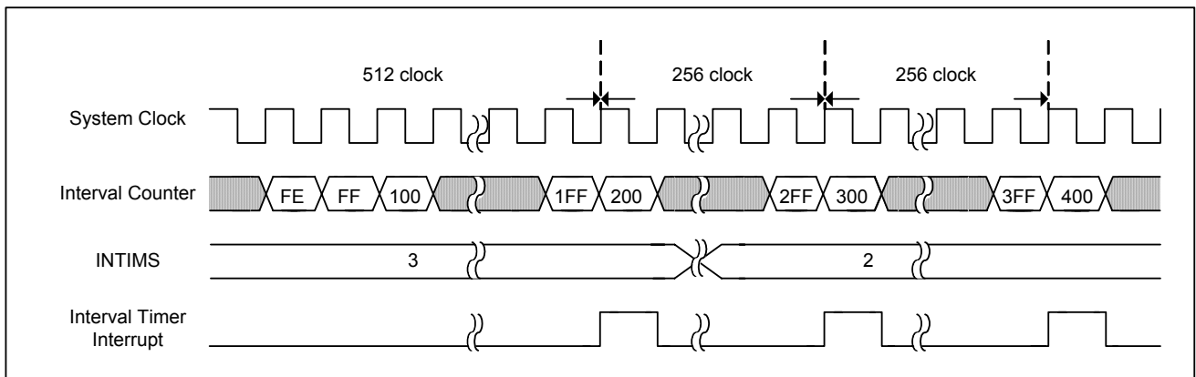
图 5-38 时基定时器工作时序
