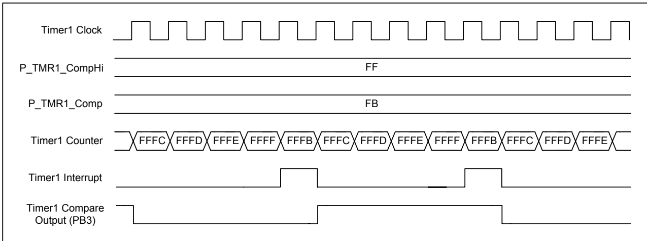
图 5-28 16 位比较输出的时序
