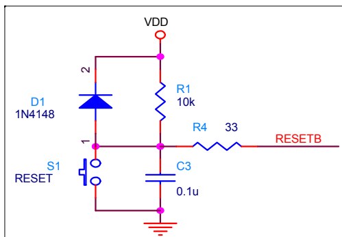
图 5-15 外部复位电路
