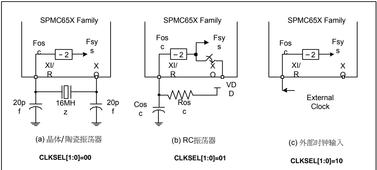
图 5-6 三种时钟源的典型应用电路
