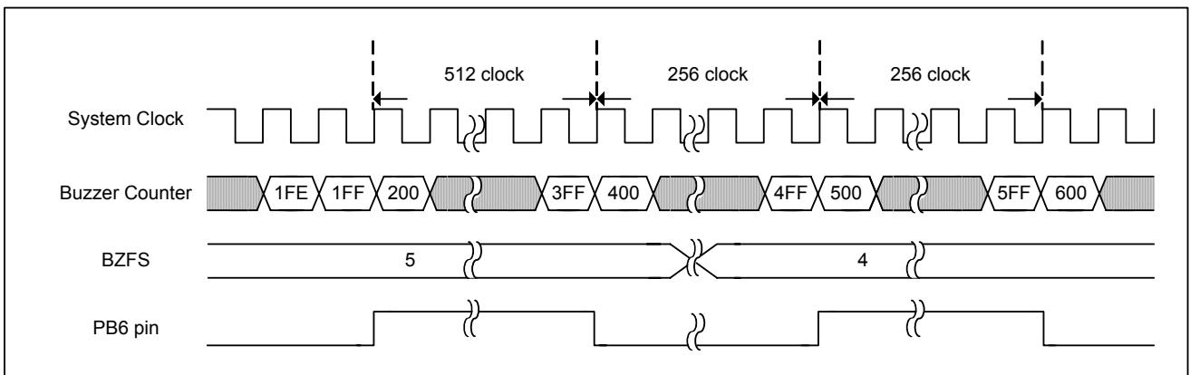
图 5-39 蜂鸣器运行时序
