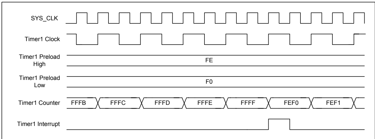
图 5-26 16 位定时/计数器计数溢出及中断时序
