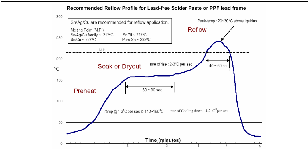
图 7-2 采用 Lead-free 焊膏或 PPF lead frame 的 SMT 温度曲线
