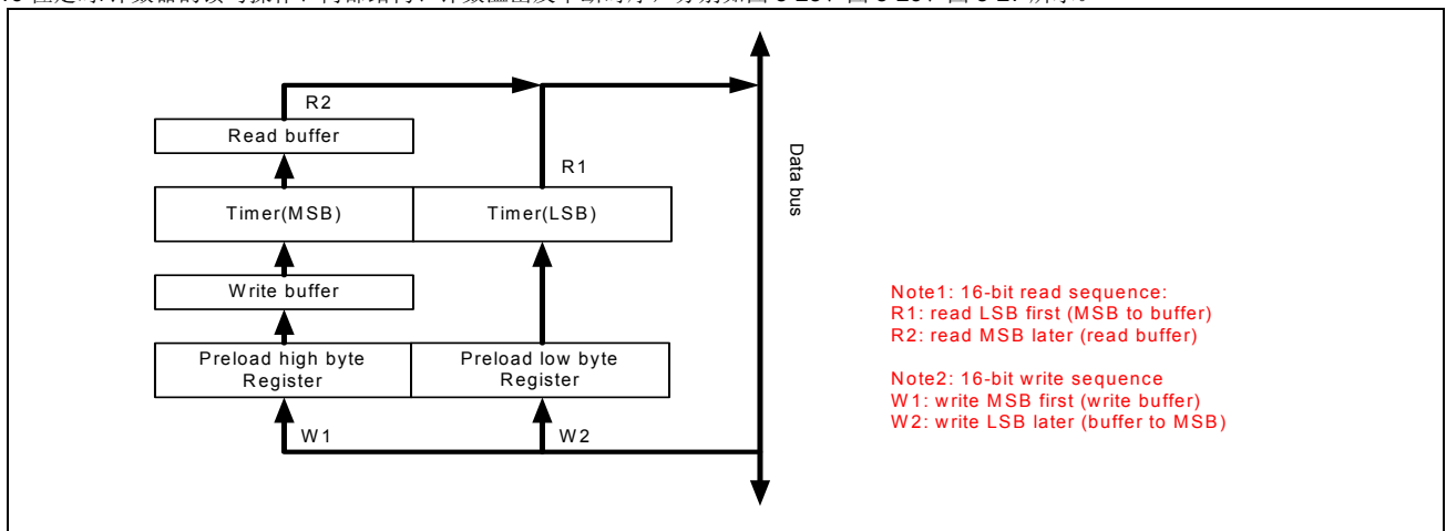
图 5-24 16 位定时/计数器读写操作框图
