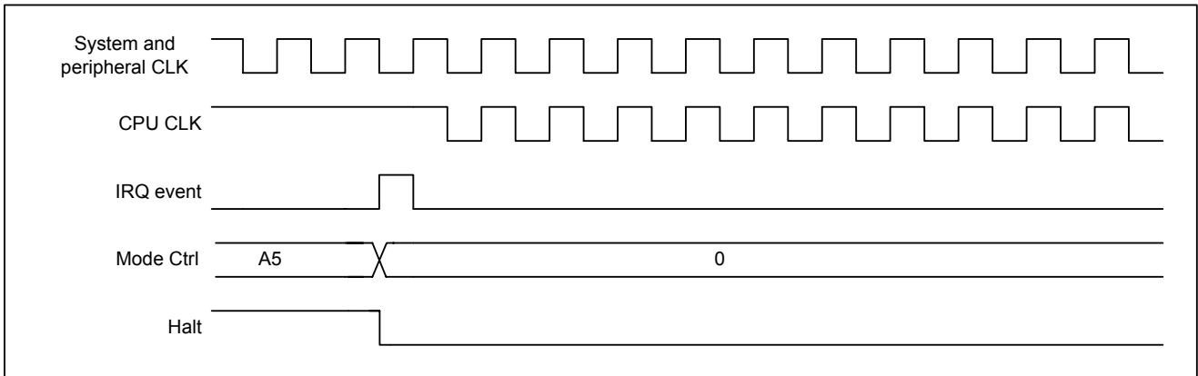
图 5-12 中断唤醒 HALT 模式的时序
