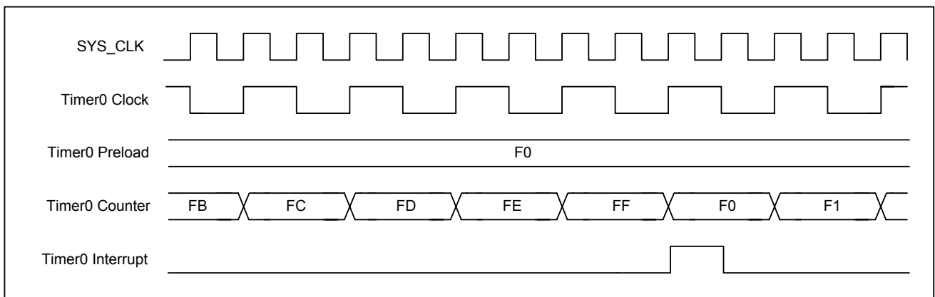
图 5-23 8 位定时/计数器 0 计数溢出及中断时序
