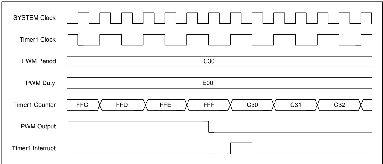
图 5-33 12 位 PWM 模式下计数初值的重载时序
