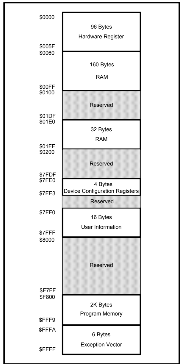
图 5-5 SPMC65P2202A 存储空间分配图
