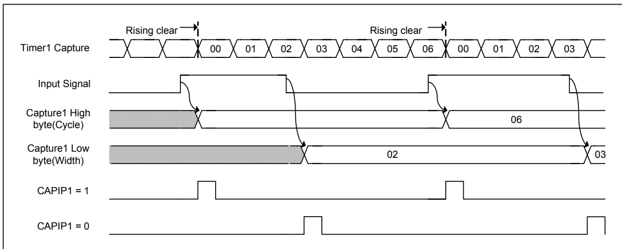
图 5-29 8 位捕获的工作时序
