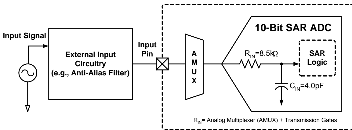
图 6-1 ADC 采样简化结构图
