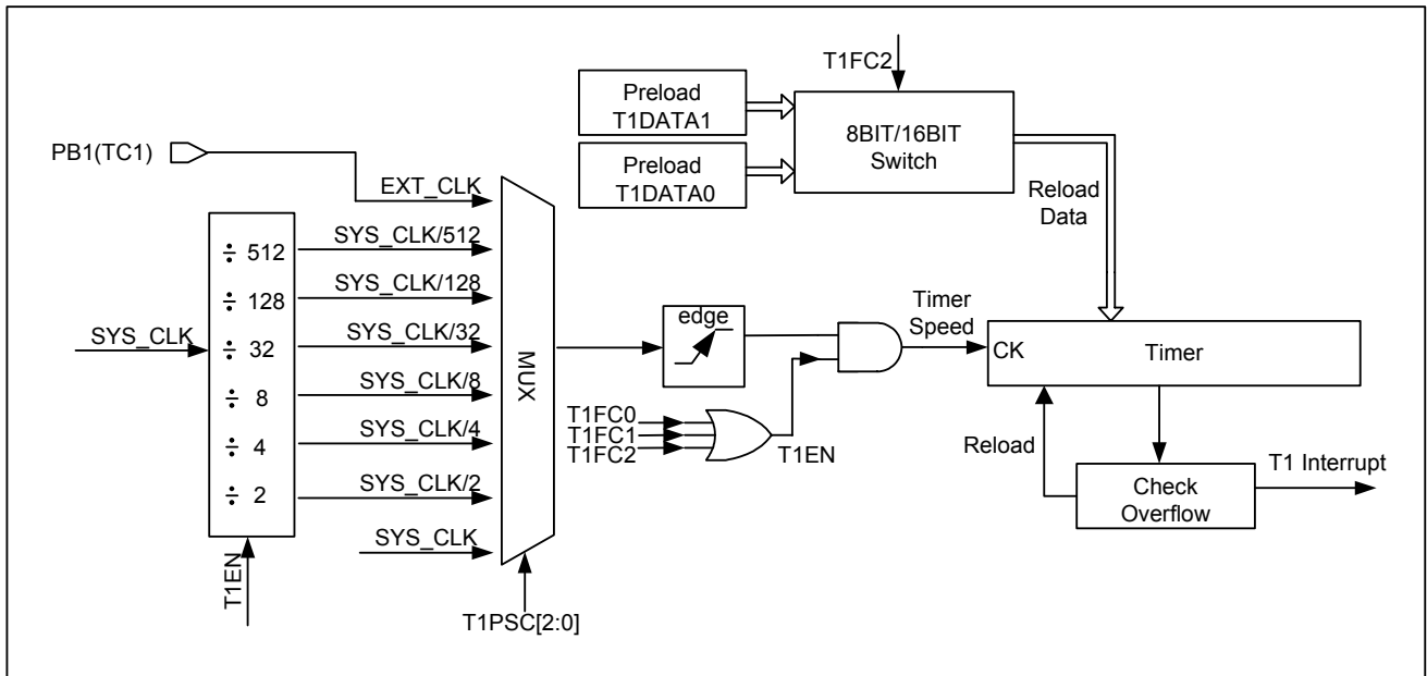
图 5-25 16 位定时/计数器内部结构图
