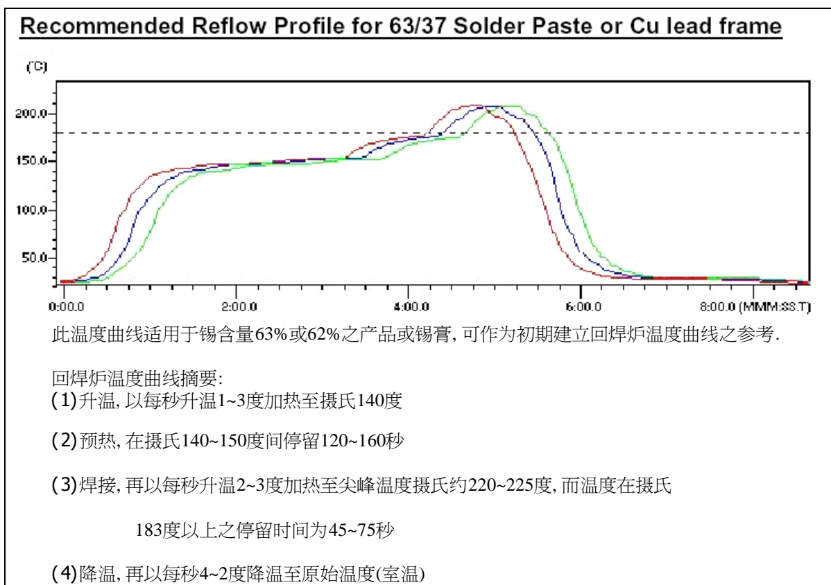
图 7-1 采用 63/37 焊膏或铜 lead frame 的 SMT 温度曲线
