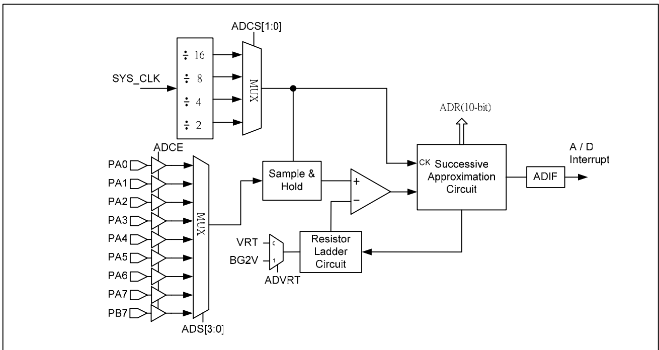
图 5-35 AD 转换原理图
