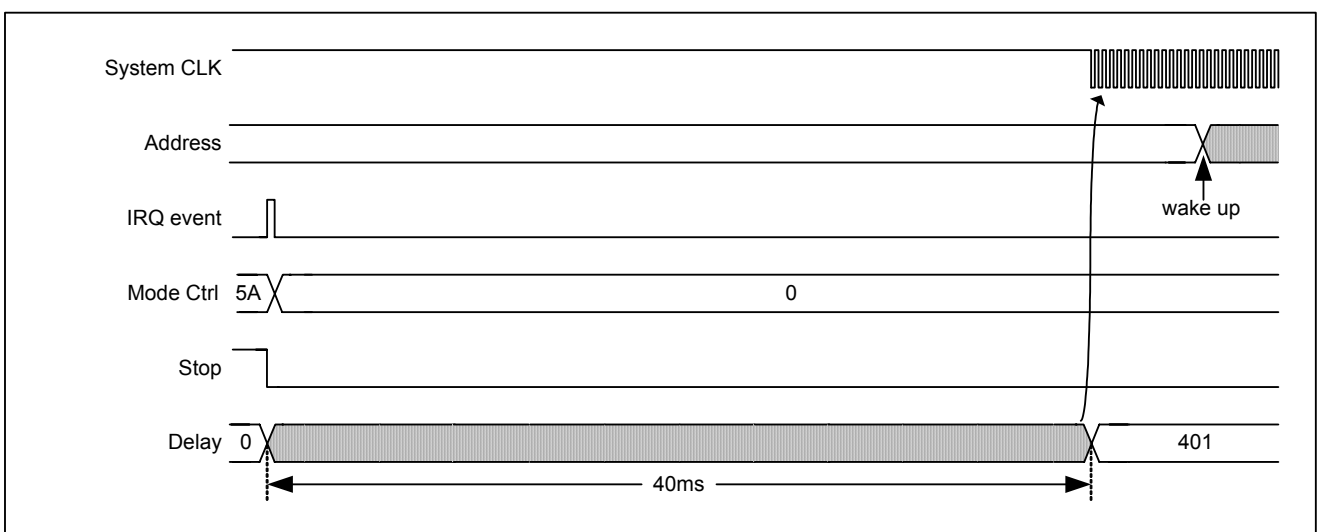
图 5-9 外部中断唤醒 STOP 模式的时序
