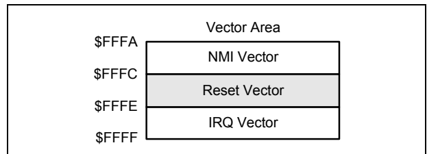
图 5-3 中断和复位向量表
