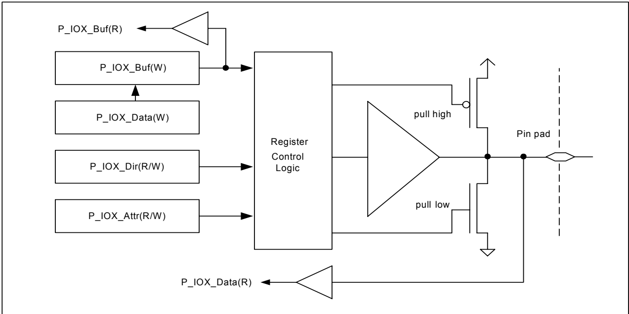
图 5-21 IO 端口结构图
