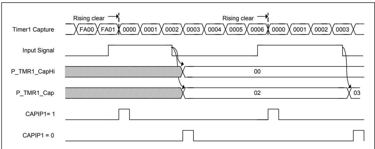
图 5-31 16 位捕获的工作时序
