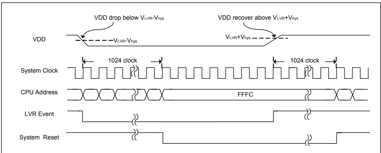
图 5-18 低电压复位时序
