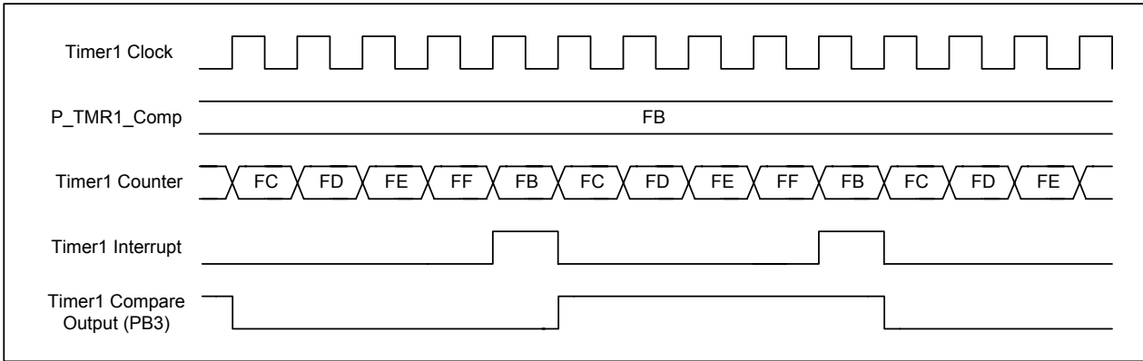
图 5-27 8 位比较输出的时序
