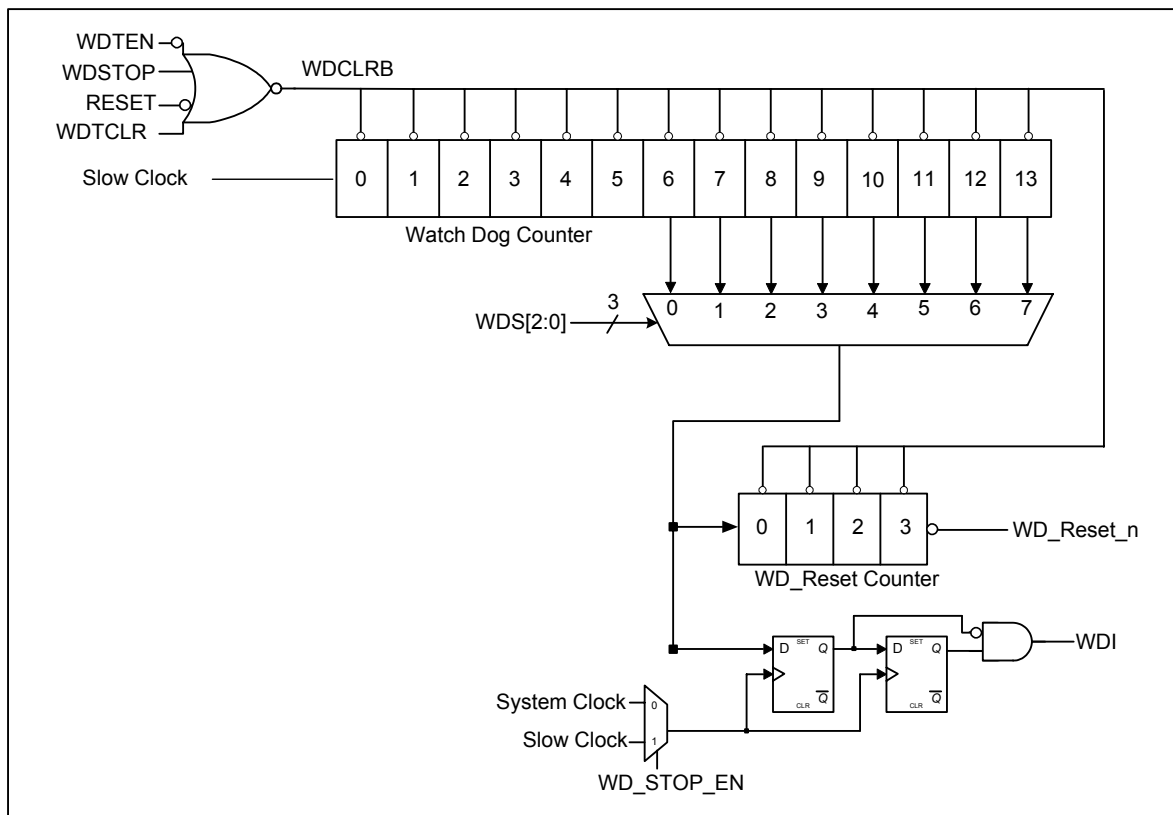
图 5-37 看门狗定时器原理框图
