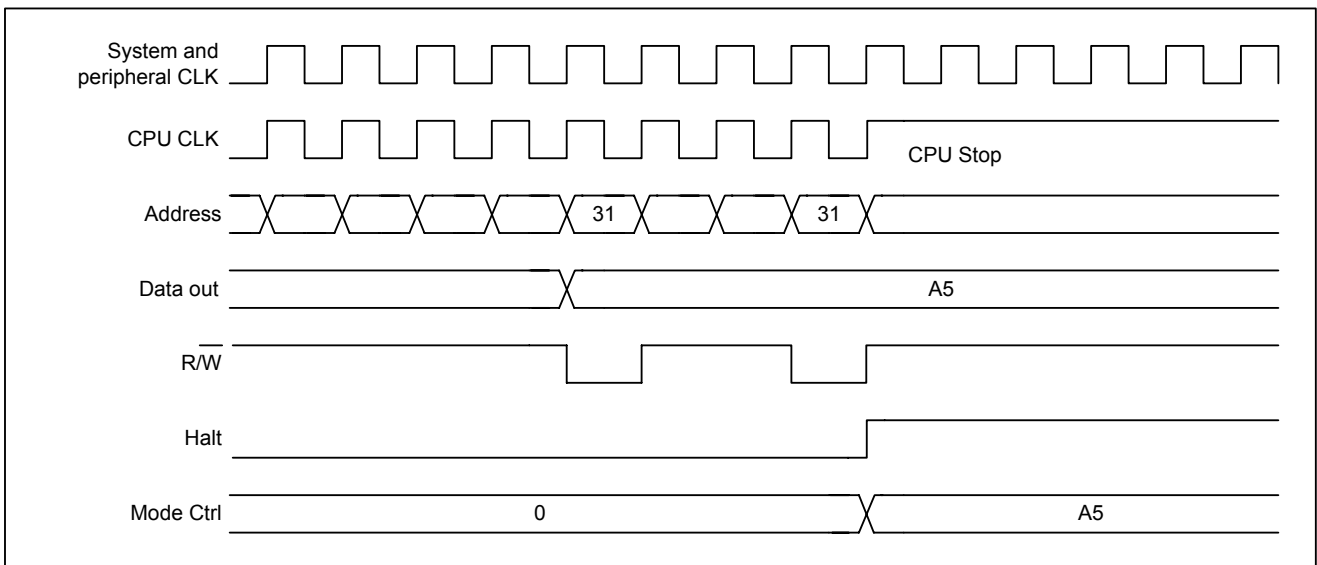
图 5-11 进入 HALT 模式的时序
