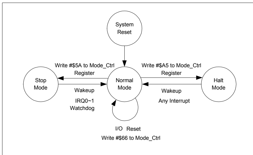
图 5-7 SPMC65P2204A/2202A 的工作模式转换
