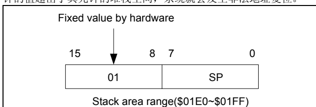
图 5-2 堆栈指针寄存器
