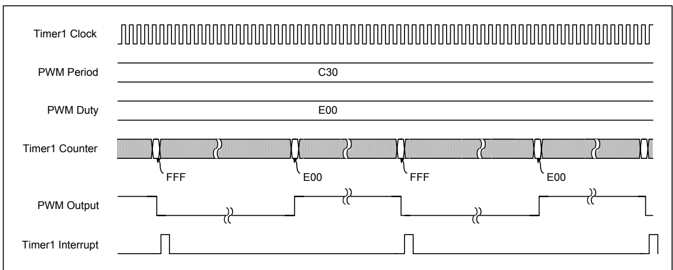
图 5-32 12 位 PWM 模式的工作时序
