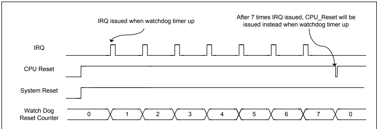
图 5-19 看门狗复位时序
