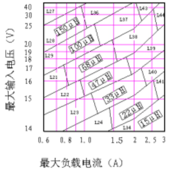
图6 LM2596 —12
