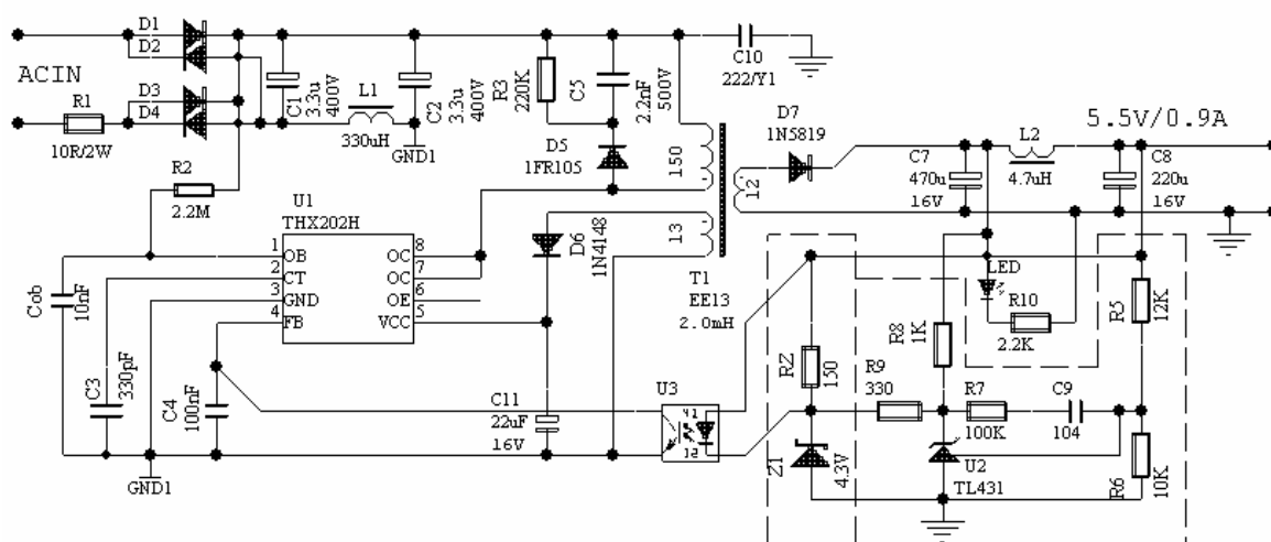
图 3、手机充电器
