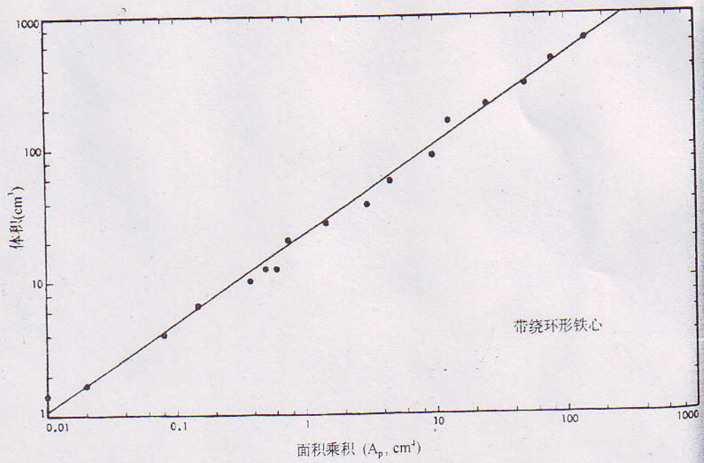
图 2.15 带绕环形铁心体积与面积乘积 A_p 的关系曲线
