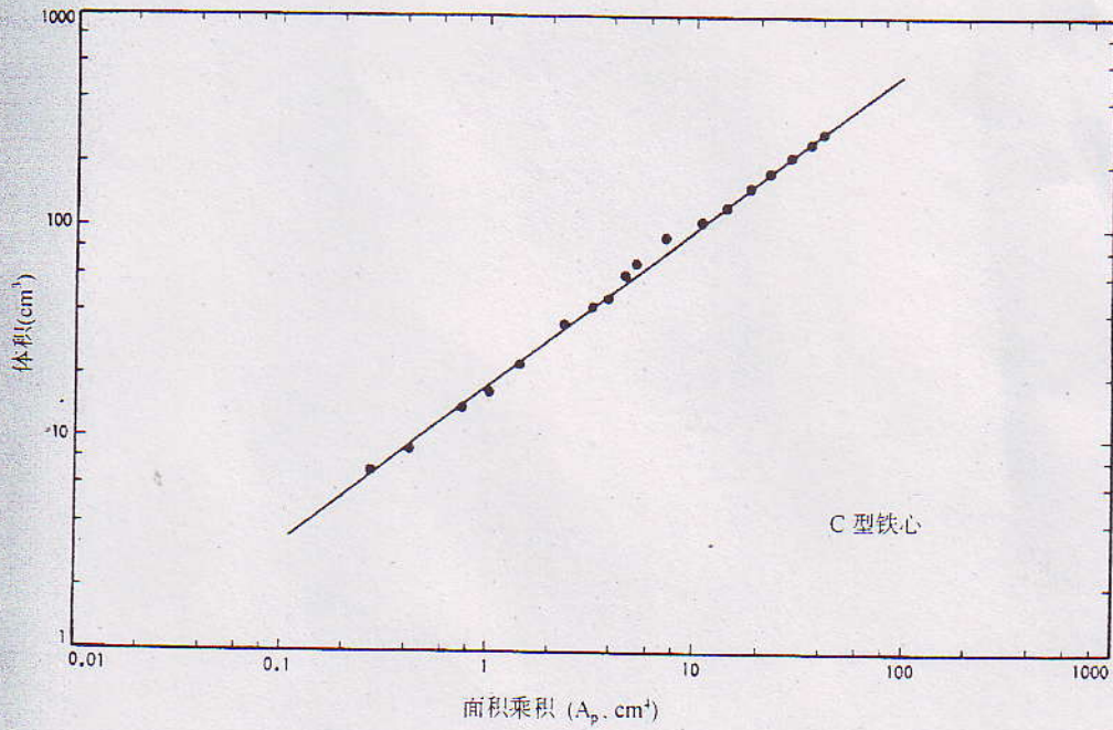
图 2.13 C 型铁心体积与面积乘积 A_p 的关系曲线
