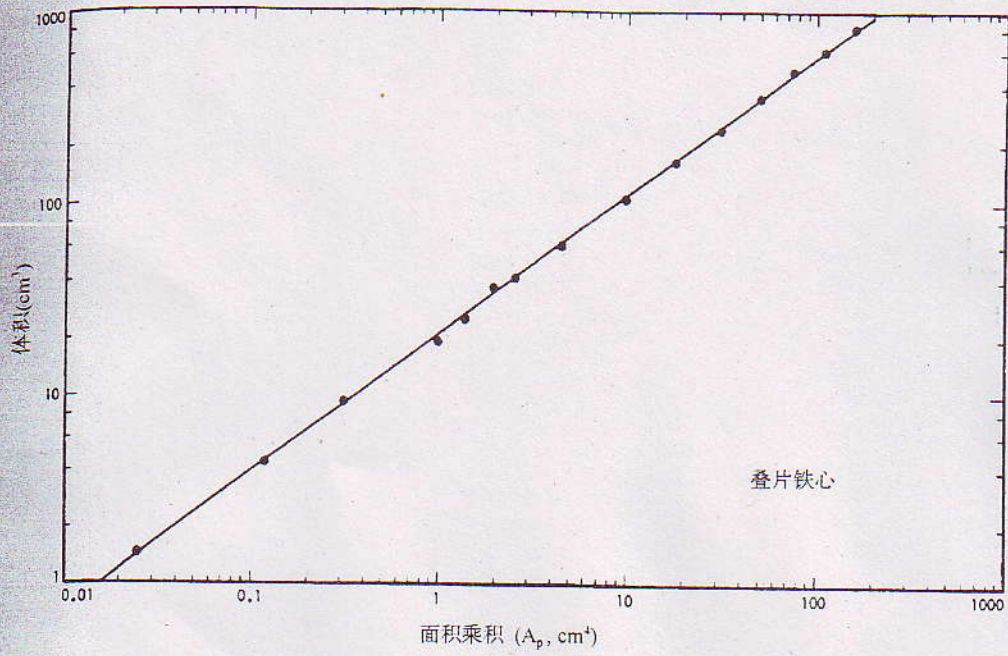
图 2.12 叠片铁心体积与面积乘积 A_p 的关系曲线
