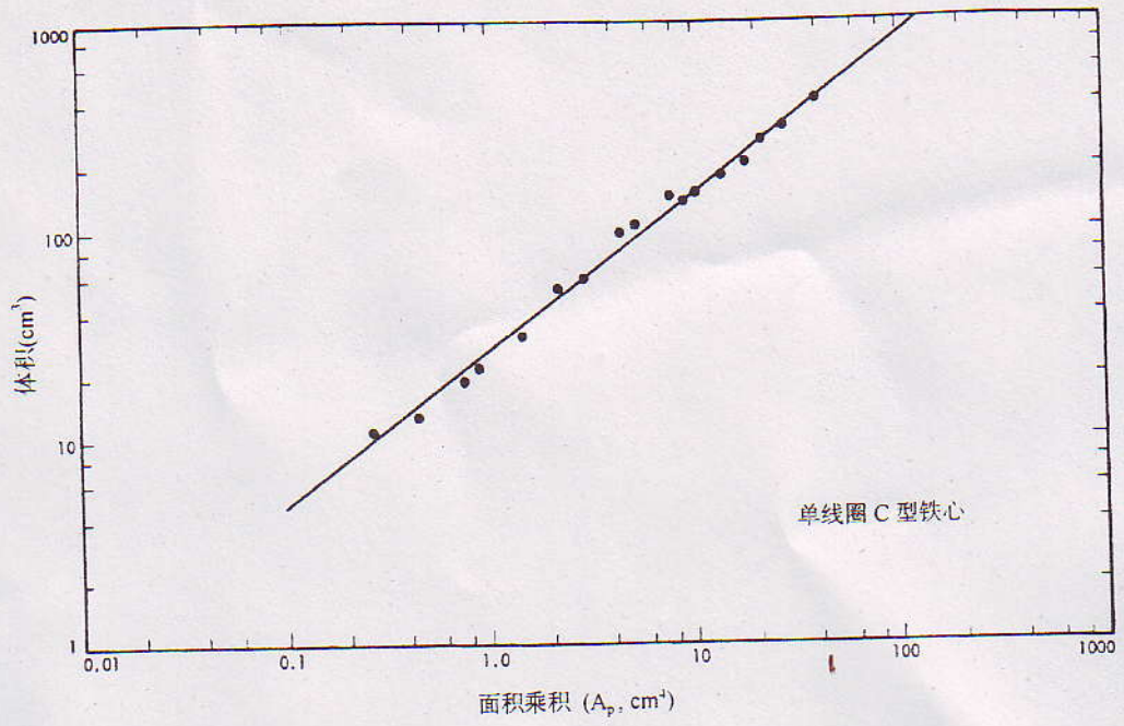
图 2.14 单线圈 C 型铁心体积与面积乘积 A_p 的关系曲线
