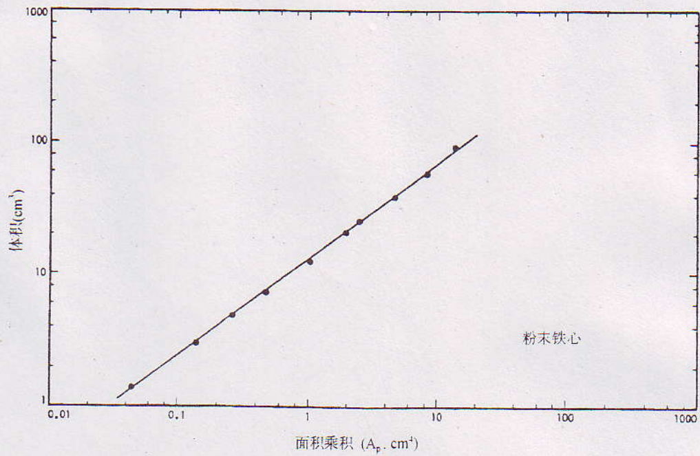
图 2.11 粉末铁心体积与面积乘积的关系曲线
