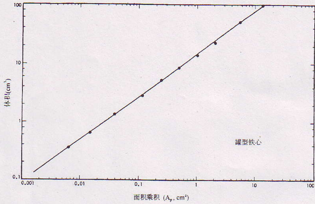
图 2.10 罐型铁心体积与面积乘积的关系曲线
