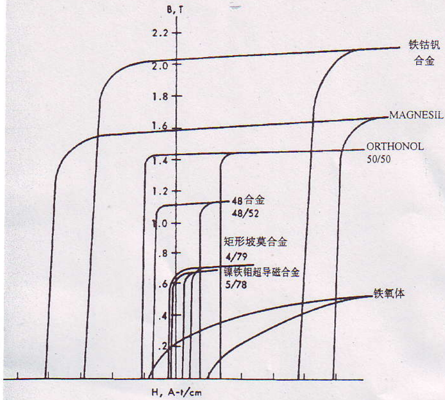
图 3.12 部分磁心材料的典型 dc B-H 回线
