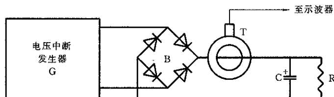
G—电压中断发生器,在 90^\circ 和 270^\circ 上转换;T—电流探头,可输出给示波器来监视;B—整流桥;R—分流电阻器,100 \Omega R \leq 10\ 000 \Omega ; C—1 700 \mu\text{F} \pm 20\% 的电解电容器
