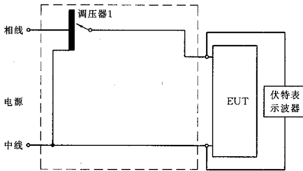
图 C1 b) 采用功率放大器进行电压跌落和短时中断试验原理图
