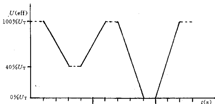
图 1 电压暂降
