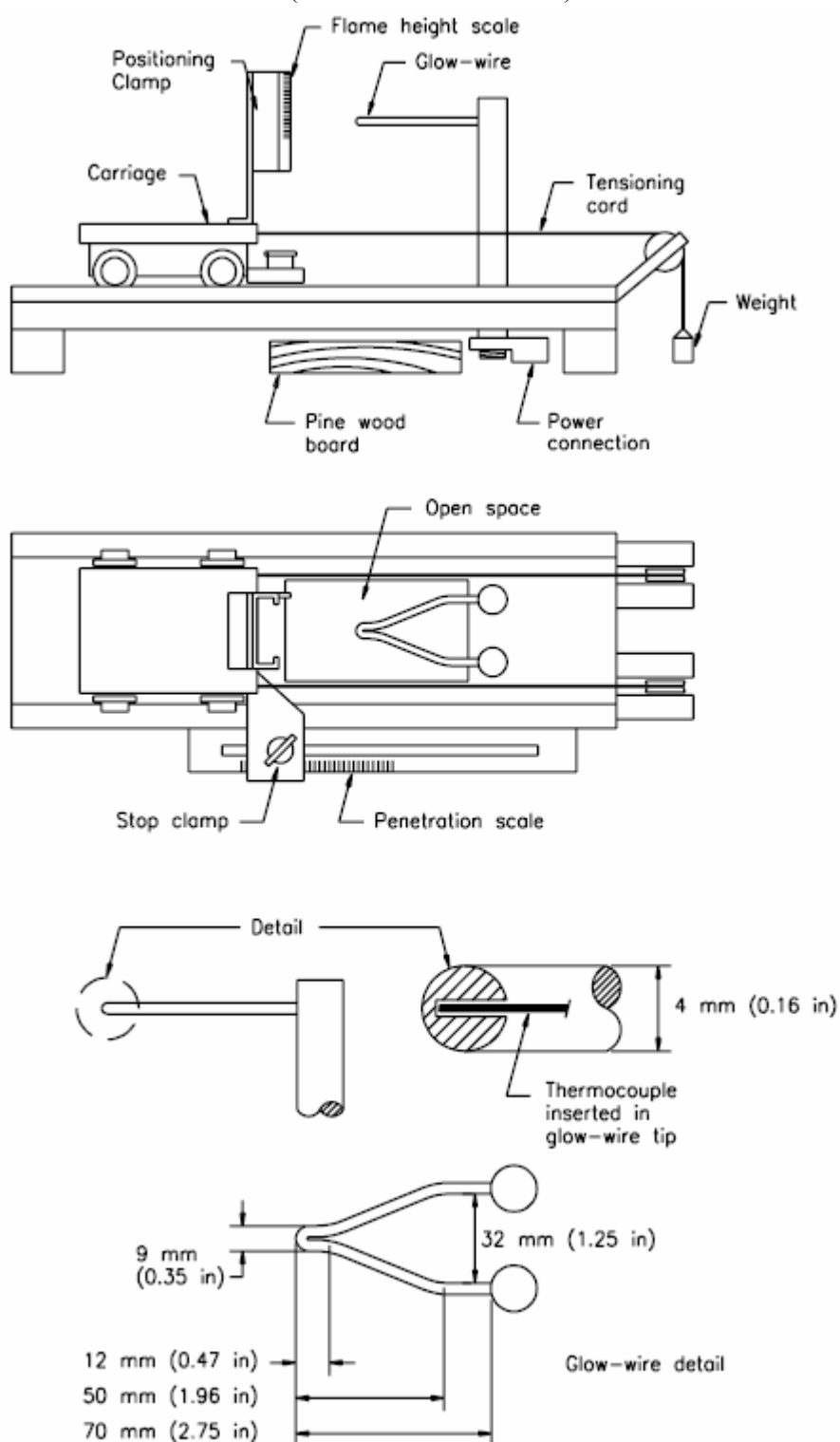
图19.28.1 灼热丝试验设备 (见16.7.6条和 19.28.1条)
