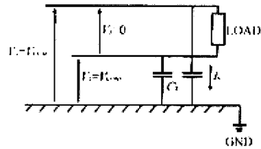
图3 共模信号
