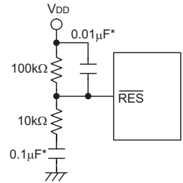
复位电路 注意: “*” 为了避免噪声干扰, 连接 \overline{\text{RES}} 引脚的线应尽量短
