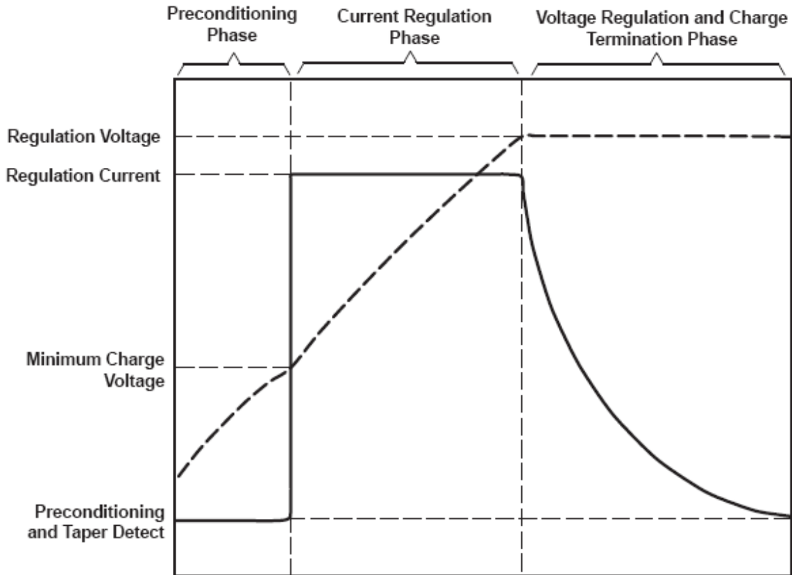
图 5、充电曲线
