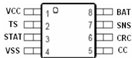
图 1.2、FS3871B MSOP 封装图
