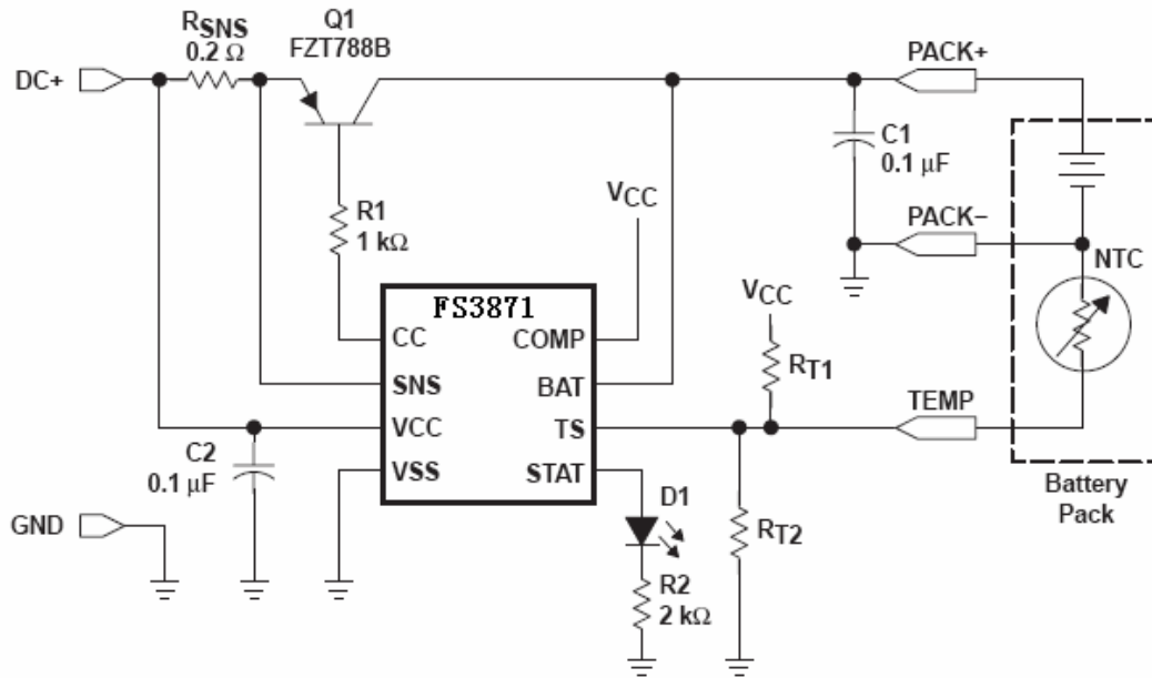
图 3、应用电路图 1
