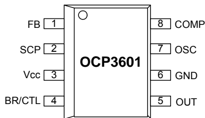
1) SOP8
