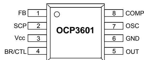
2) MSOP8
