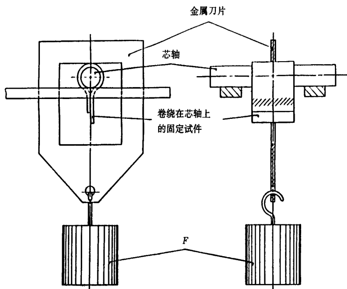
图 2 压痕试验装置
