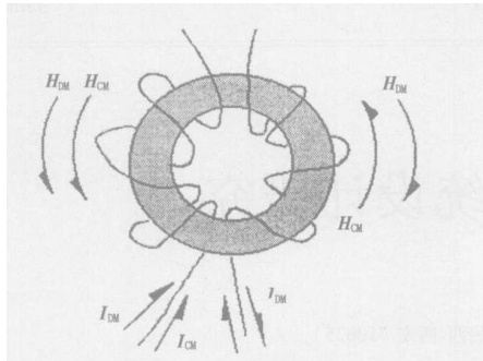
图 4 共模电感的基本结构
