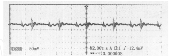
图 6 滤波前电源噪声/50mV
