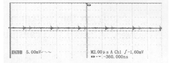
图 7 滤波后电源噪声/5mV
