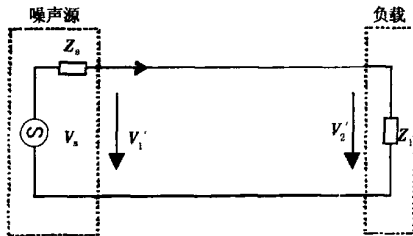
图 2 接入滤波器时
