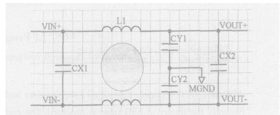
图 3 滤波电路基本结构
