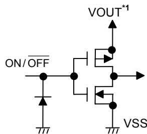
图 14 \overline{\text{ON/OFF}} 端子的构造
