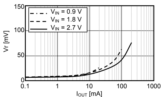
条件 13 S-8357N33
