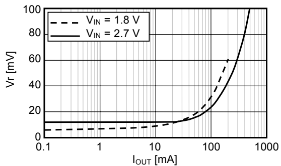
条件 15 S-8356Q33
