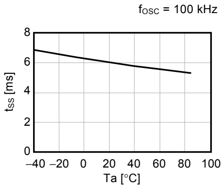
(12) 软启动时间( t_{SS} ) — 温度( T_a ) ( V_{OUT} = 3.3\text{ V} )
