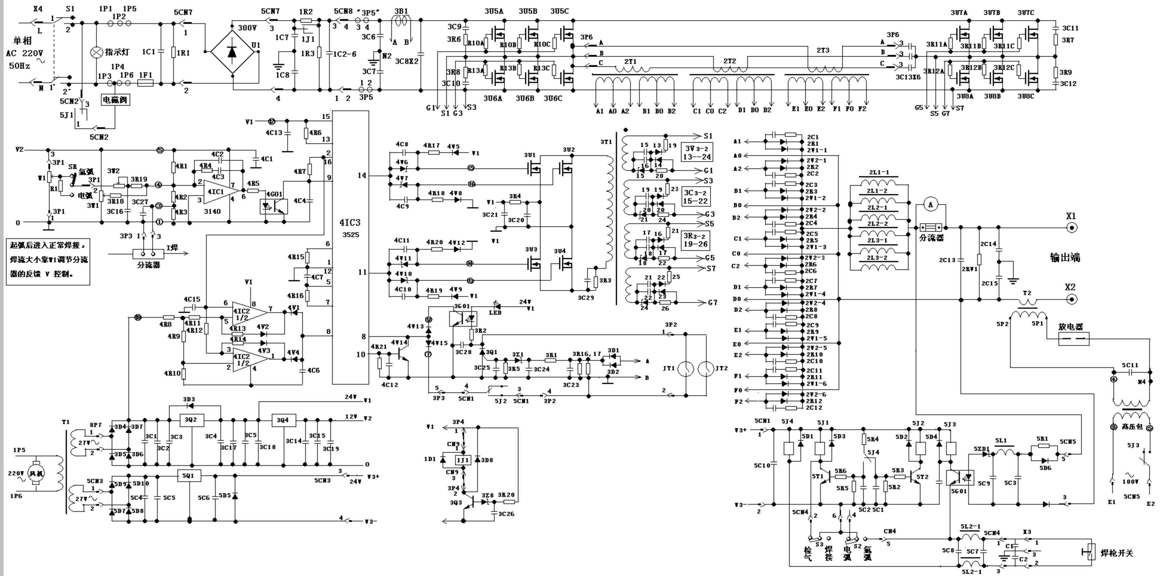
WS-160 逆变氩弧焊机电路原理图
